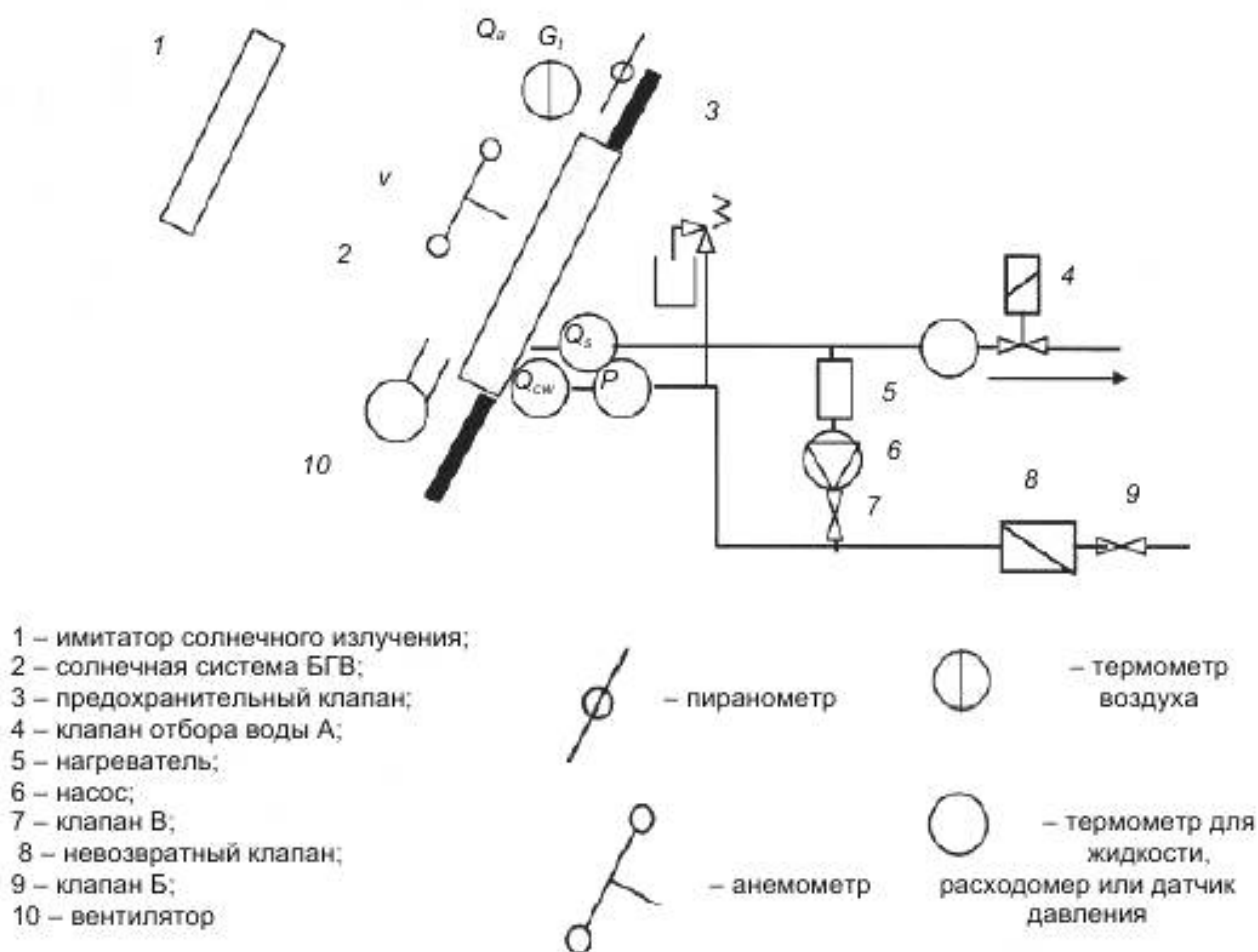
Рисунок В.6 – Схема структуры испытания
