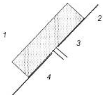
1 – солнечная система БГВ; 2 – наклонная крыша; 3 – трубы системы, через отверстие в крыше; 4 – температура внутри помещения
