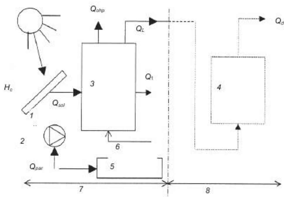
1 – коллектор; 2 – насос; 3 – бак-накопитель; 4 – дополнительный нагреватель 5 – устройство управления; 6 – холодная вода; 7 – система предварительного нагрева; 8 – дополнительные нагревательные установки
