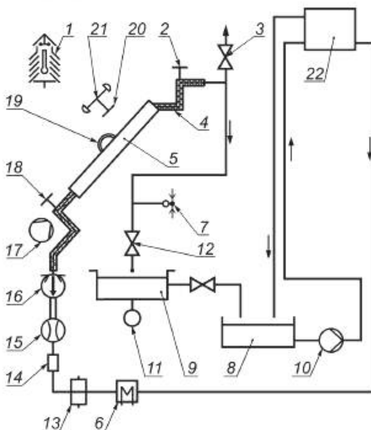
Рисунок 3 — Пример открытого (разомкнутого) испытательного контура
