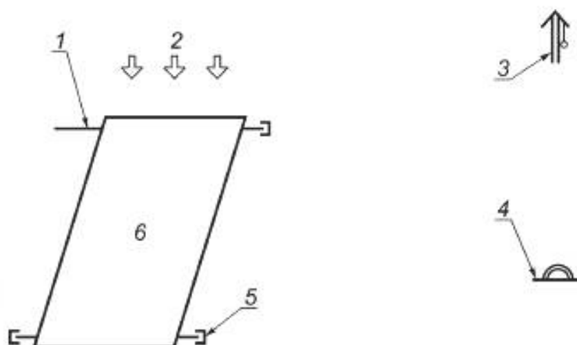
1 — Трубопровод, оставленный открытый; 2 — Солнечная радиация; 3 — Датчик температуры окружающей среды; 4 — Пиранометр на плоскости коллектора; 5 — Трубопровод, запечатанный с накидной гайкой; 6 — Коллектор
