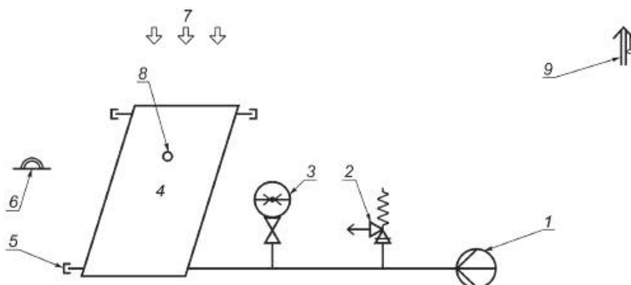
1 — Источник пневматического давления; 2 — Предохранительный клапан; 3 — Манометр; 4 — Коллектор с органическим поглотителем; 5 — Трубопровод, запечатанный с накидной гайкой; 6 — Пирометр на плоскости коллектора; 7 — Естественный или искусственный солнечный радиатор; 8 — Температурный датчик, прикрепленный к поглотителю; 9 — Датчик температуры окружающей среды
