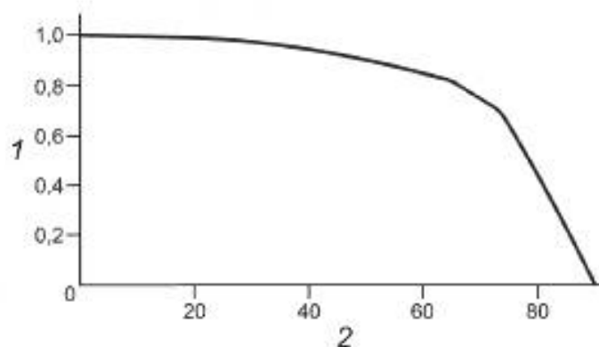
Рисунок 6 — Типовая зависимость K_{\theta} от угла падения
