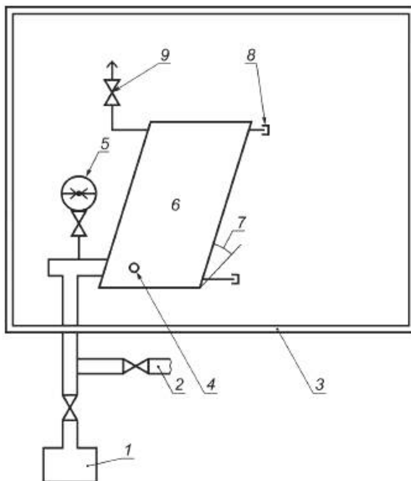
1 — Водный источник; 2 — Дренаж (только для устройств с водоотводом); 3 — Камера термостатирования; 4 — Температурный датчик; 5 — Манометр; 6 — Коллектор; 7 — Угол наклона; 8 — Трубопровод, запечатанный с накладной гайкой; 9 — Воздушный выпускной клапан
