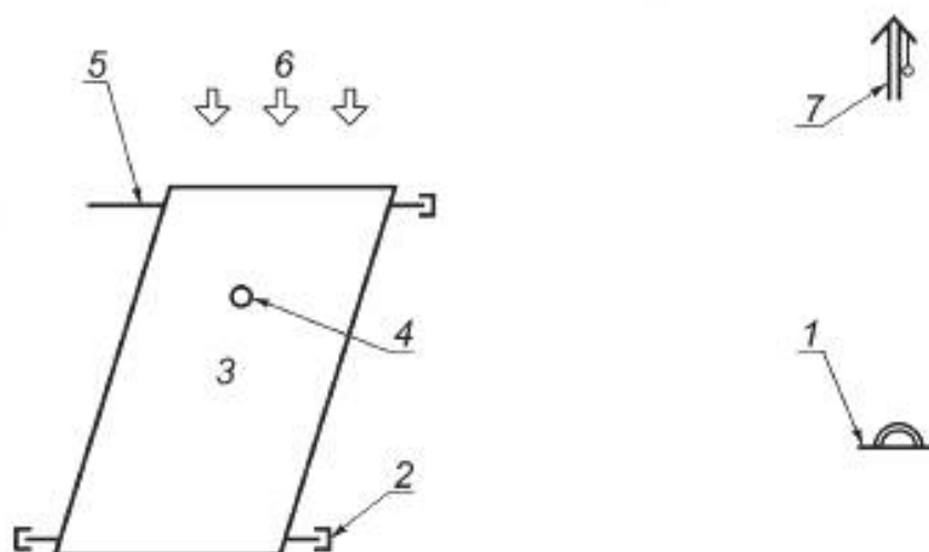
1 — Пирометр на плоскости коллектора; 2 — Трубопровод, запечатанный с накидной гайкой; 3 — Коллектор; 4 — Температурный датчик, прикрепленный к поглотителю; 5 — Трубопровод, оставленный открытым; 6 — Естественное или искусственное солнечное излучение; 7 — Датчик температуры окружающей среды
