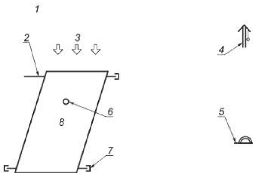
1 — Водные брызги на всех сторонах; 2 — Трубопровод, оставленный открытый; 3 — Естественная или искусственная солнечная радиация; 4 — Датчик температуры окружающей среды; 5 — Пиранометр на плоскости коллектора; 6 — Температурный датчик, прикрепленный к поглотителю; 7 — Трубопровод, запечатанный с накидной гайкой; 8 — Коллектор
