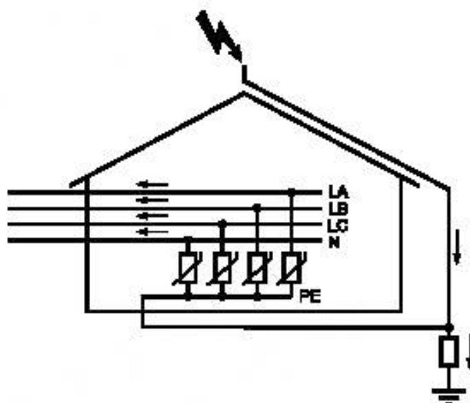
Рисунок 7 — Пример резистивной связи с системой молниезащиты
