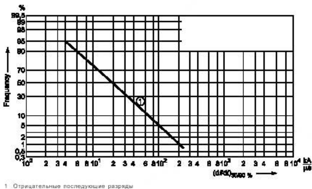
Рисунок А.6 — Частотное распределение производной тока (di/df)_{30/50 \%} отрицательных вторичных разрядов
