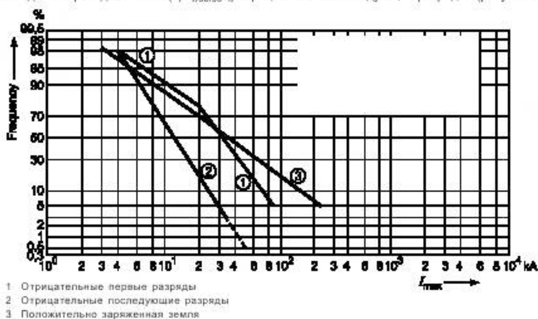
Рисунок А.1 — Частотное распределение максимального тока молнии I_{\max}
