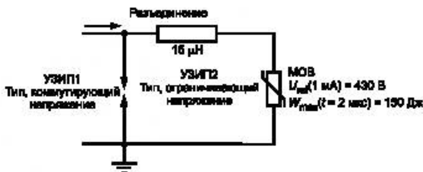
Рисунок Е.9 — Пример координации между коммутирующим напряжением УЗИП и ограничивающим напряжением УЗИП
