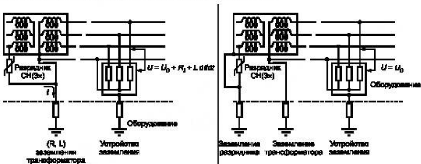
Рисунок 8 — Типовые механизмы связи по земле
