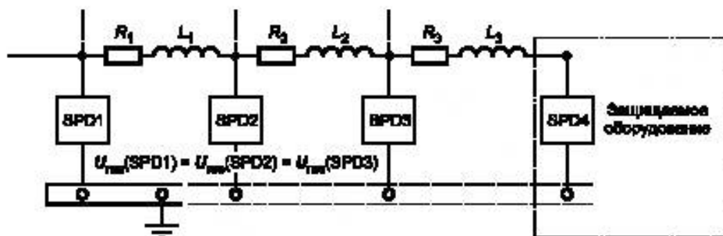
Рисунок Е.16 — Принцип координации для вида I
