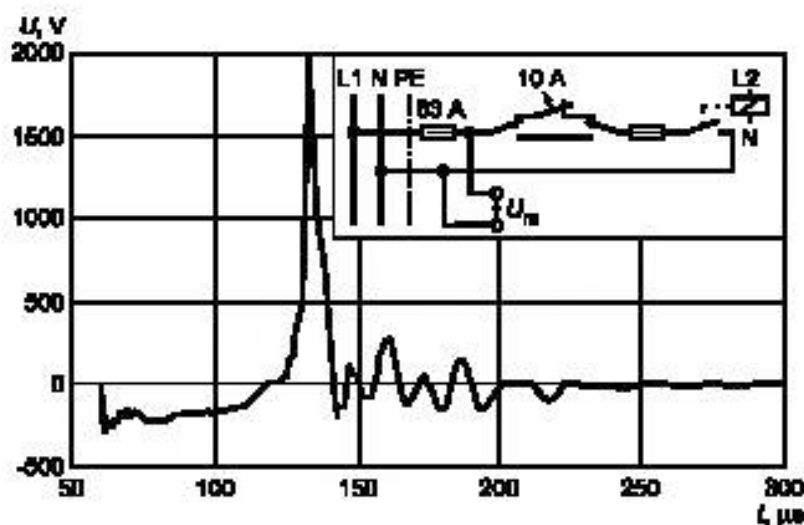
Рисунок 21 — Импульсные коммутационные перенапряжения при срабатывании миниатюрного предохранителя
