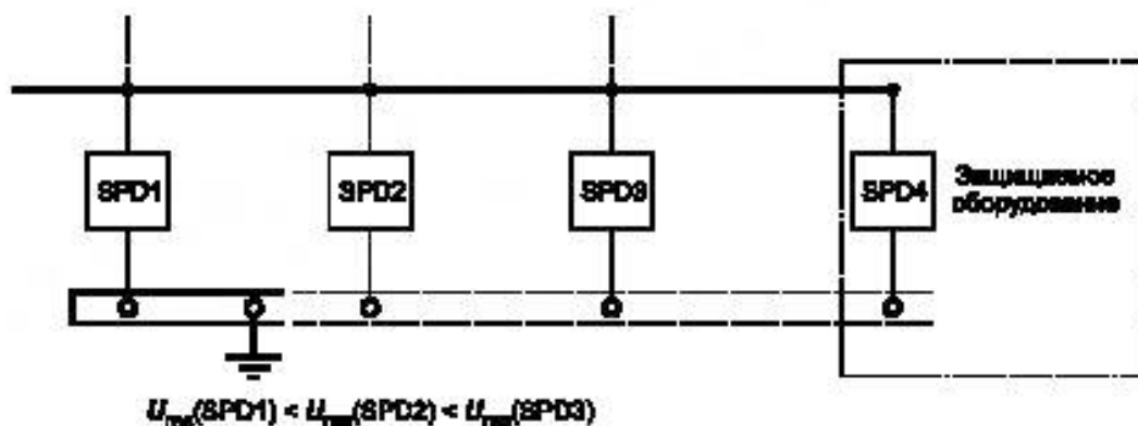
Рисунок Е.17 — Принцип координации для вида II
