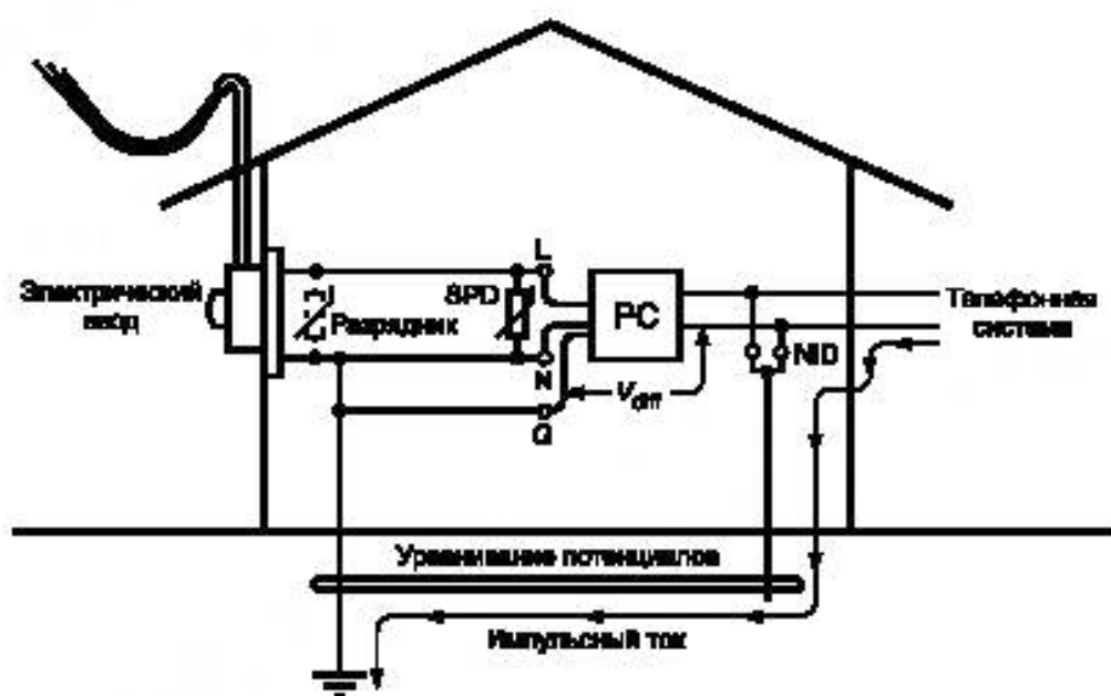
Рисунок D.2 — Разность потенциалов на ПК/модеме во время импульса тока
