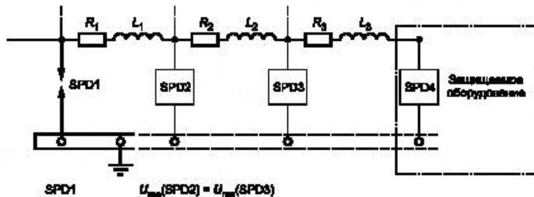
Рисунок Е.18 — Принцип координации для вида III
