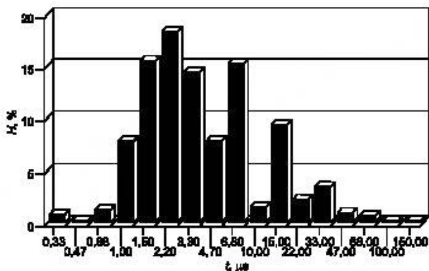
Рисунок 19 — Распределение импульсных коммутационных перенапряжений по продолжительности
