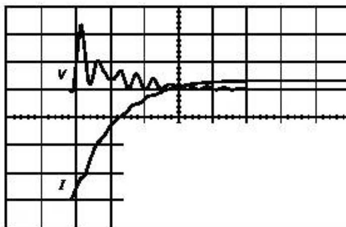
I Входной ток NID 50 А/дел; di/dt = 75 А/мкс V Напряжение между телефонным портом и защитным проводником (РЕ) 2 кВ/дел; максимум 4,3 кВ. Горизонтальная развертка: 2 мкс/дел
