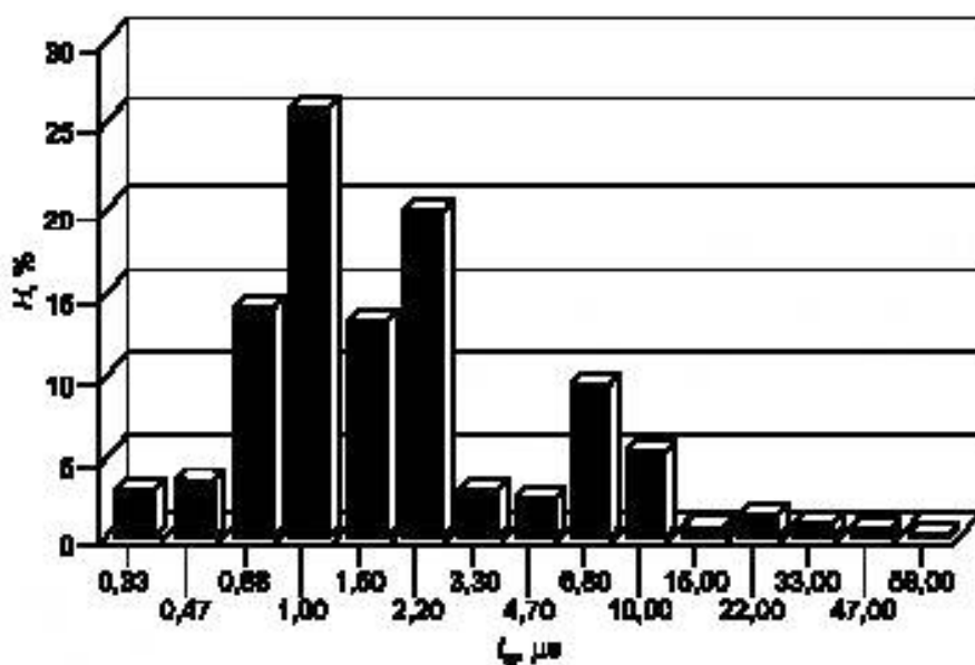
Рисунок 17 — Распределение импульсных коммутационных перенапряжений по времени
