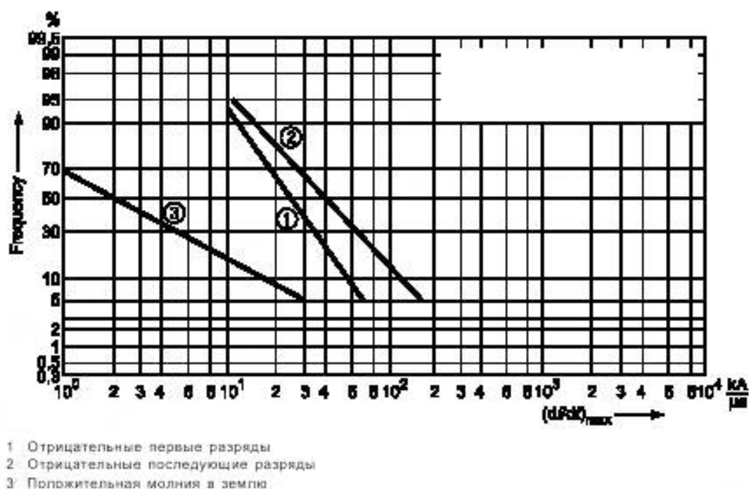
Рисунок А.5 — Частотное распределение максимальной производной переходного тока (di/df)_{\max}
