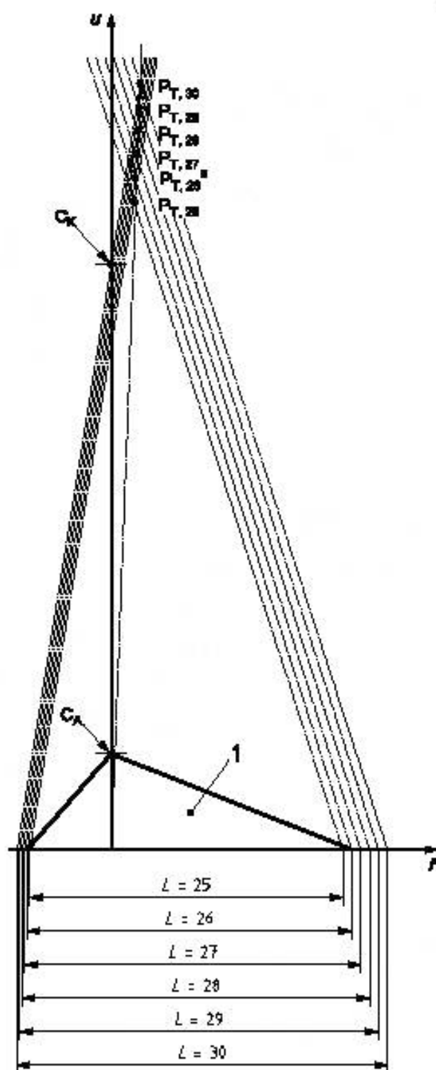
Рисунок 6 – Иллюстрация зависимости положения верхней точки приложения нагрузки P_T от длины узла стопы L (см. 2.2.3)
