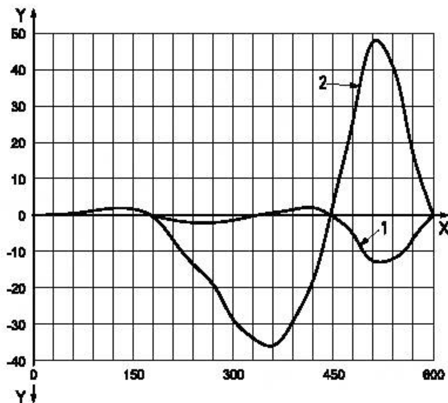
Рисунок 16 – Иллюстрация отклонения сил, воспроизводимых кривошипно-шатунным механизмом 60:40
