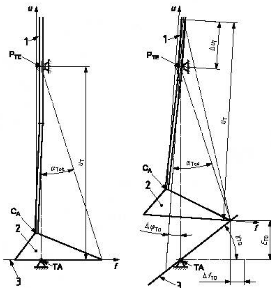
Рисунок 22 – Иллюстрация влияния A-P смещения \Delta f на угловое перемещение \Delta\phi испытываемого образца относительно «внешней» верхней точки приложения нагрузки P_{TE} в сборке согласно 3.3.3
