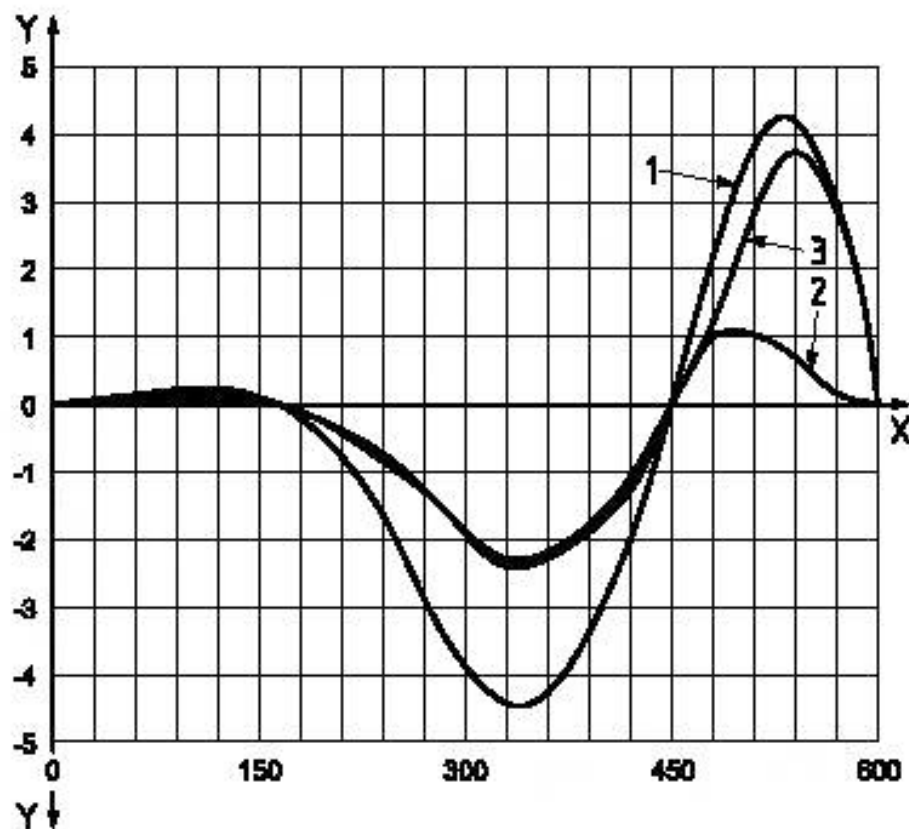
Рисунок 14 – Иллюстрация угловых отклонений, воспроизводимых кривошипно-шатунным механизмом 60:40
