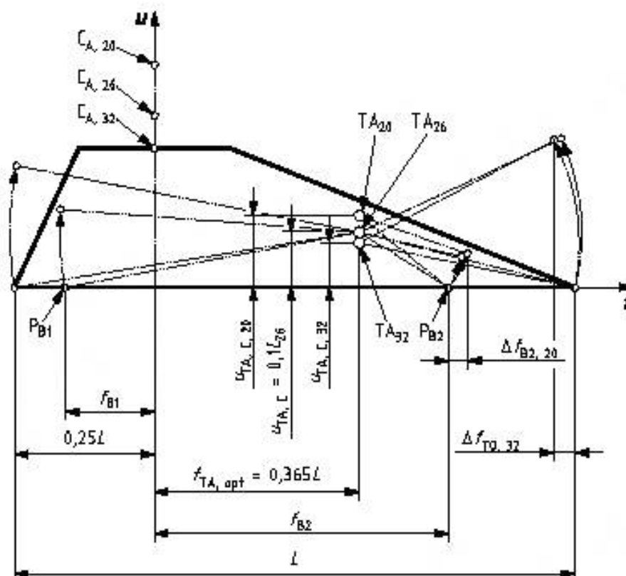
Рисунок 24 – Иллюстрация влияния постоянного компромиссного смещения u_{TA, C} оси наклона TA платформы стопы на A – P смещение \Delta f в узле стопы при разной длине узла стопы L [см. 3.8.2, пречисление с) 2)]
