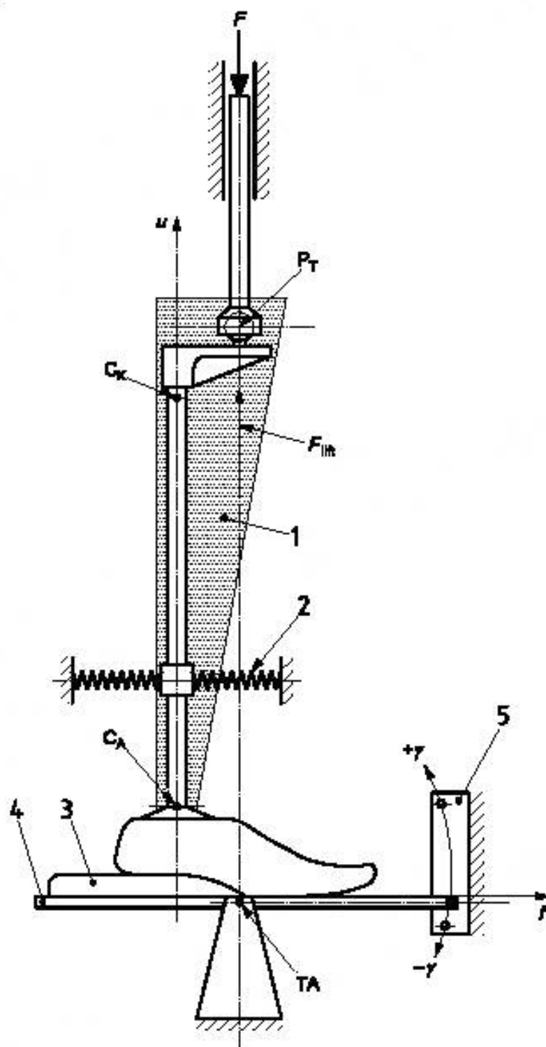
Рисунок 8 – Схематическое изображение испытательного оборудования с испытываемым образцом
