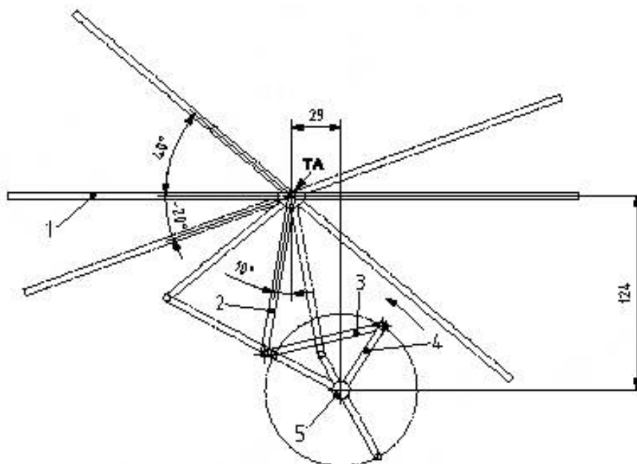
Рисунок 10 — Асимметричный (60:40) кривошипно-шатунный механизм по 3.4.2. Диапазон наклона от минус 20^\circ (контакт пятки) до плюс 40^\circ (отрыв носка)
