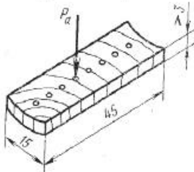
P_R – действие нагрузки вдоль волокон (в торец)
