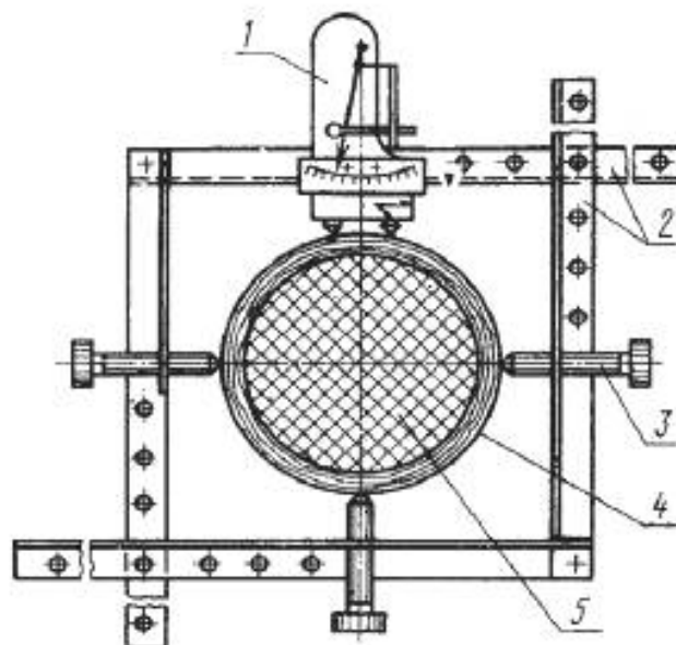
1 – тензометр; 2 – раздвижные планки; 3 – установочные винты; 4 – втулка; 5 – парафин
