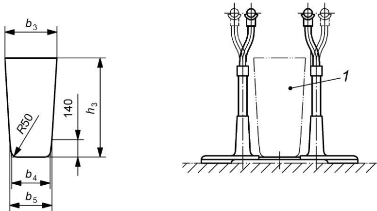
1 — испытательный шаблон в пространстве между стойками брусьев
