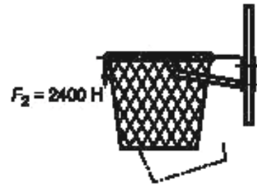
Рисунок Ж.2 — Схема приложения нагрузки к жестко закрепленному кольцу
