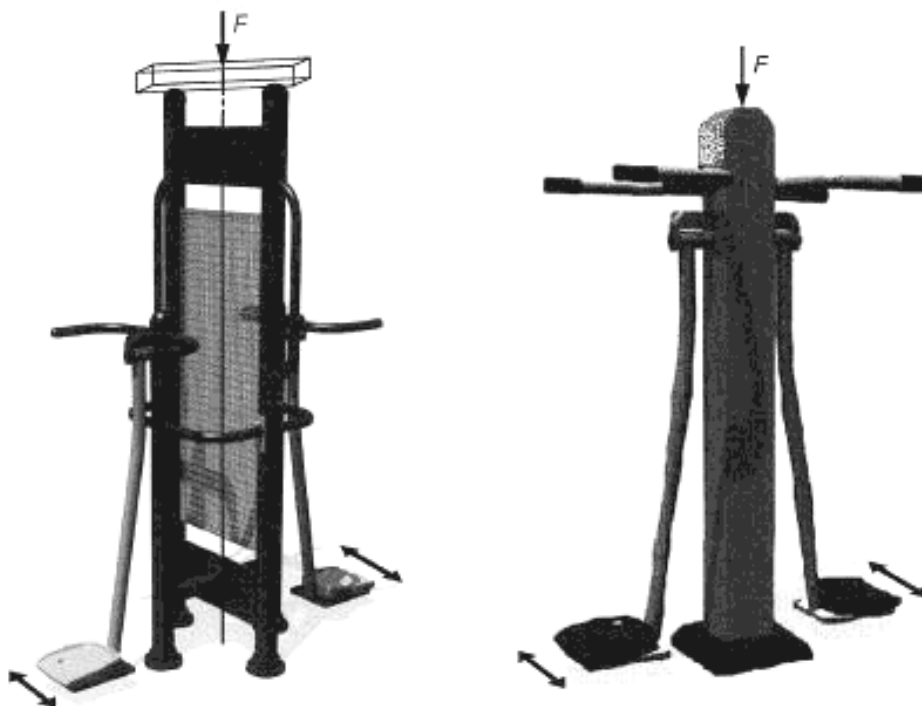
Рисунок Е.2 — Примеры приложения нагрузки
