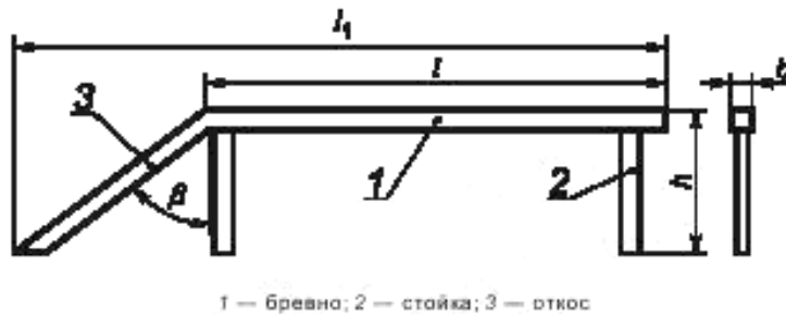
Рисунок 7 — Элементы конструкции бревна
