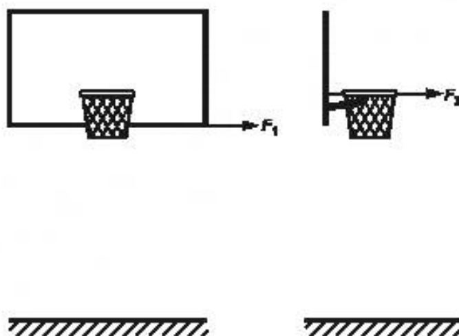
Рисунок Ж.3 — Нагружение при испытаниях на прочность
