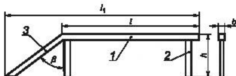
1 — бревно; 2 — стойка; 3 — откос
