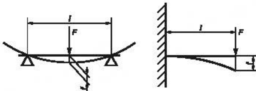
Рисунок 9 — Пример нагружения элементов тренажера
