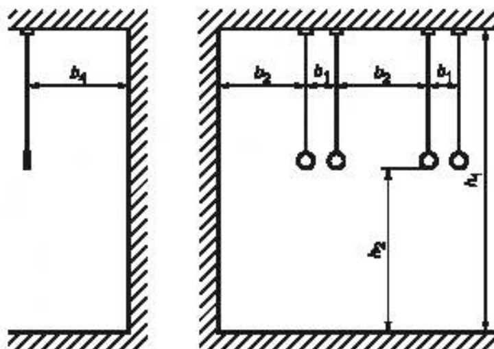
Рисунок 6 — Установочные размеры для колец
