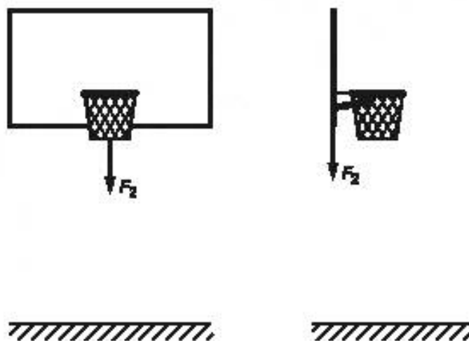
Рисунок Ж.4 — Нагружение при испытаниях на устойчивость
