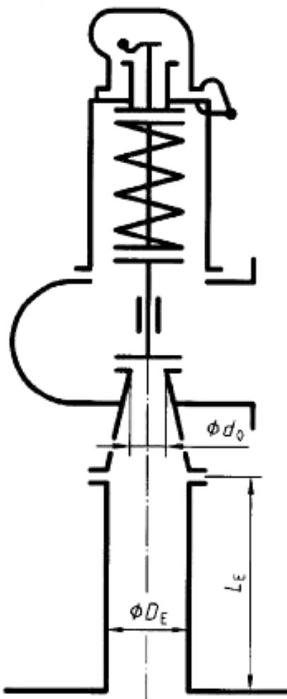
Рисунок 4.1 – Предохранительные клапаны
