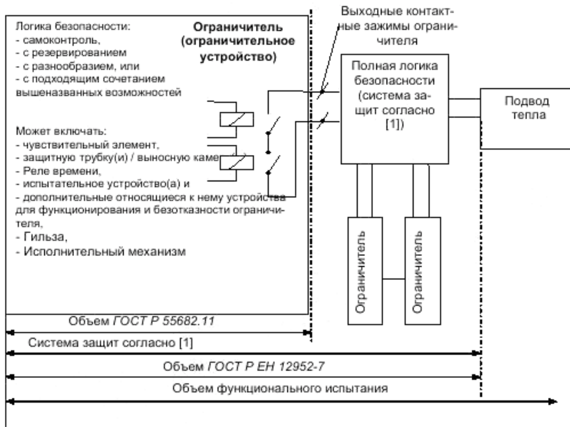
Рисунок А.1 – Ограничительное устройство
