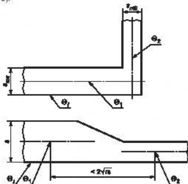
Рисунок 13.3-1 — Определение \Delta\theta
