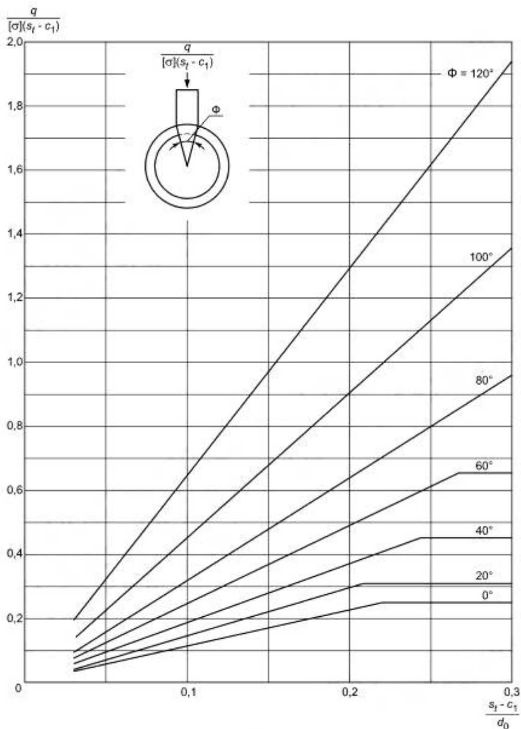
Рисунок 11.5-3 — Допустимая нагрузка сжатия для структурной технологической оснастки
