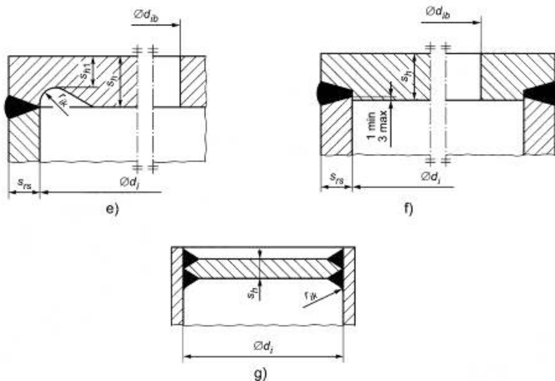
Рисунок 10.3-1, лист 2
