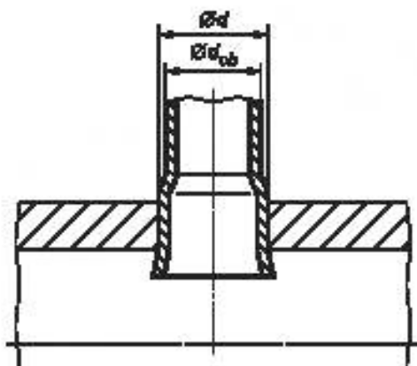
Рисунок 8.2-2 — Развальцованная труба
