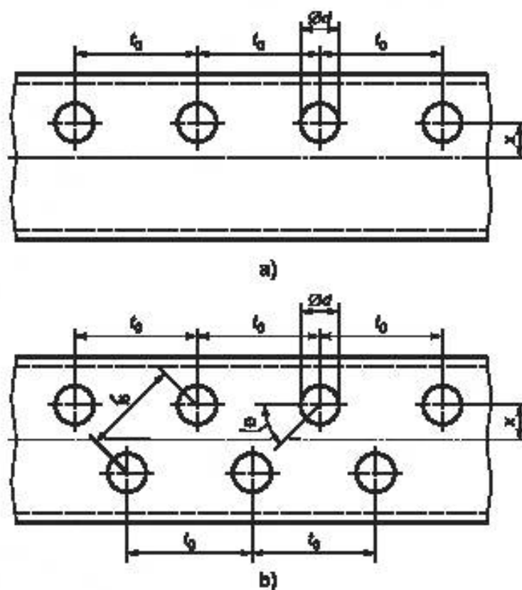
а) отверстия, расположенные по одной линии; б) отверстия, расположенные по двум параллельным линиям
