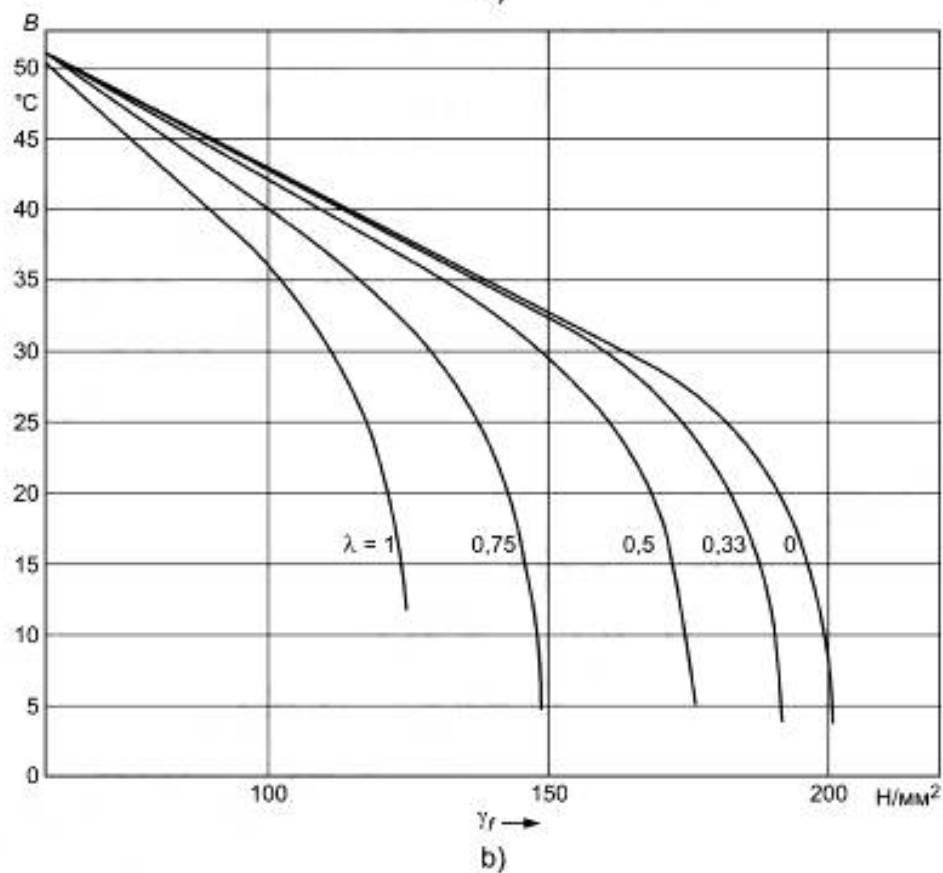
Рисунок 13.3-3 — Значения B для аустенитных нержавеющей сталей
