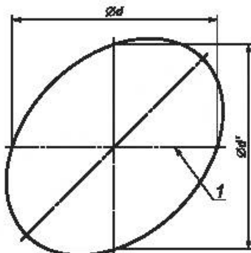
Рисунок 9.2-2 — Диаметры d и d^* для эллиптического отверстия
