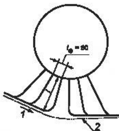
1 — поток дымового газа; 2 — граница потока дымового газа
