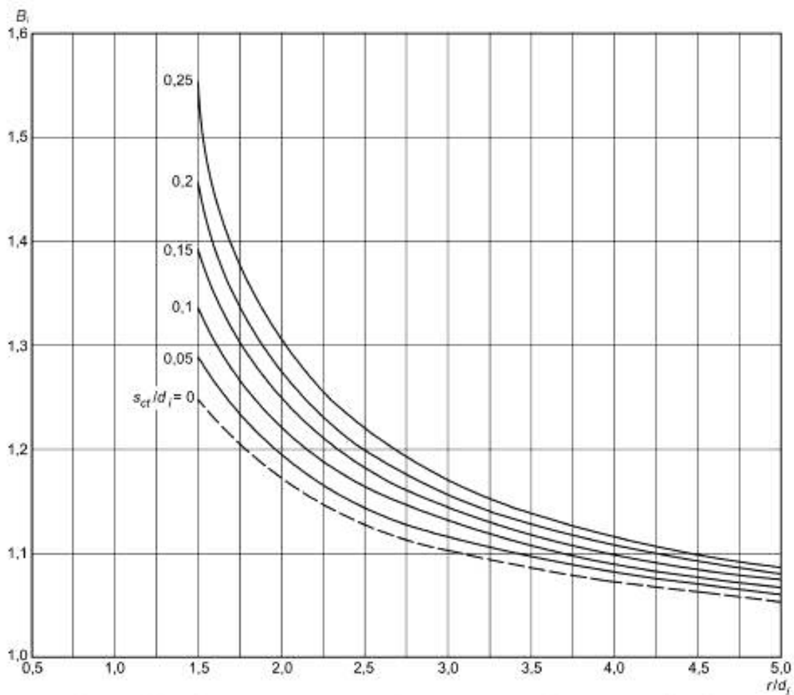
Рисунок А-2 — Расчетный коэффициент B_i для внутренней образующейгиба трубы с номинальным внутренним диаметром
