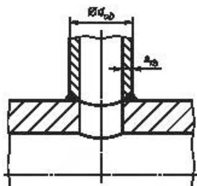
Рисунок 8.2-1 — Соединение трубы с основным корпусом
