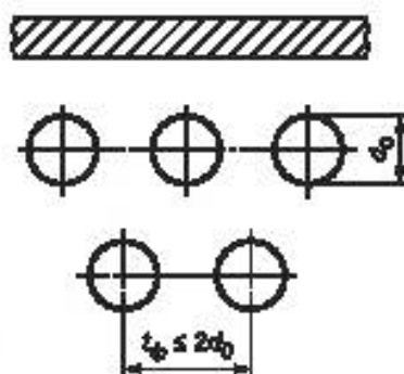
Рисунок 6.1-2 — Элементы, защищенные двумя рядами труб
