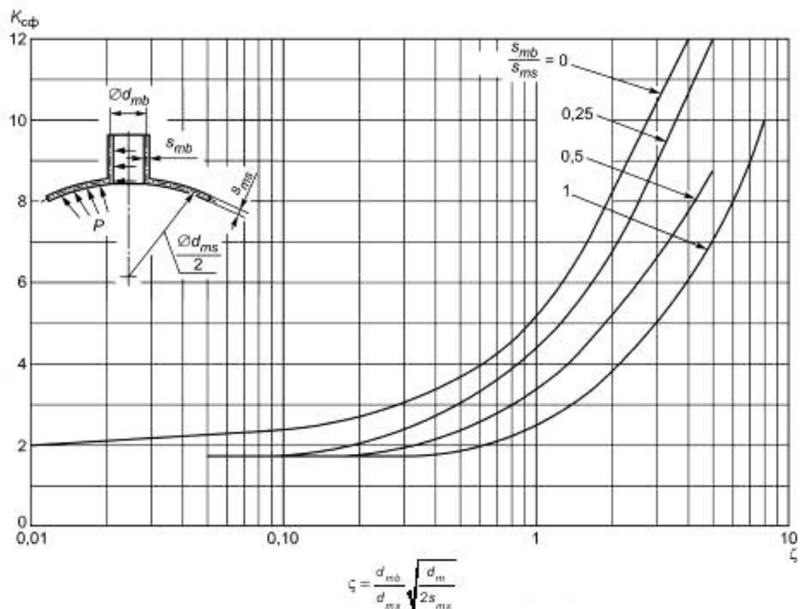
Рисунок 13.4-7, лист 2
