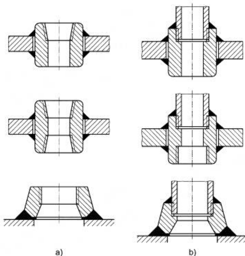
а) резьбовые; б) резьбовые и уплотненные сваркой
