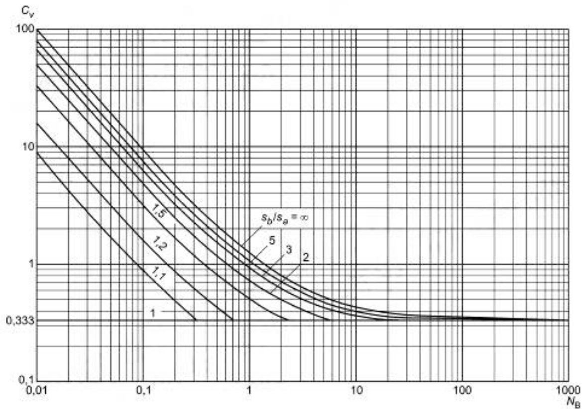
Рисунок 13.3-6 — Коэффициент C_v
