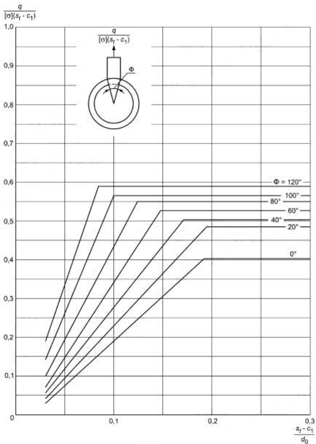
Рисунок 11.5-2 — Допустимая нагрузка растяжения для структурной технологической оснастки
