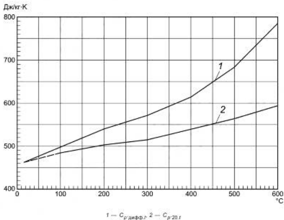
Рисунок D-3а — Теплоемкость сталей от группы 1 до группы 6 (9Cr1Mo)
