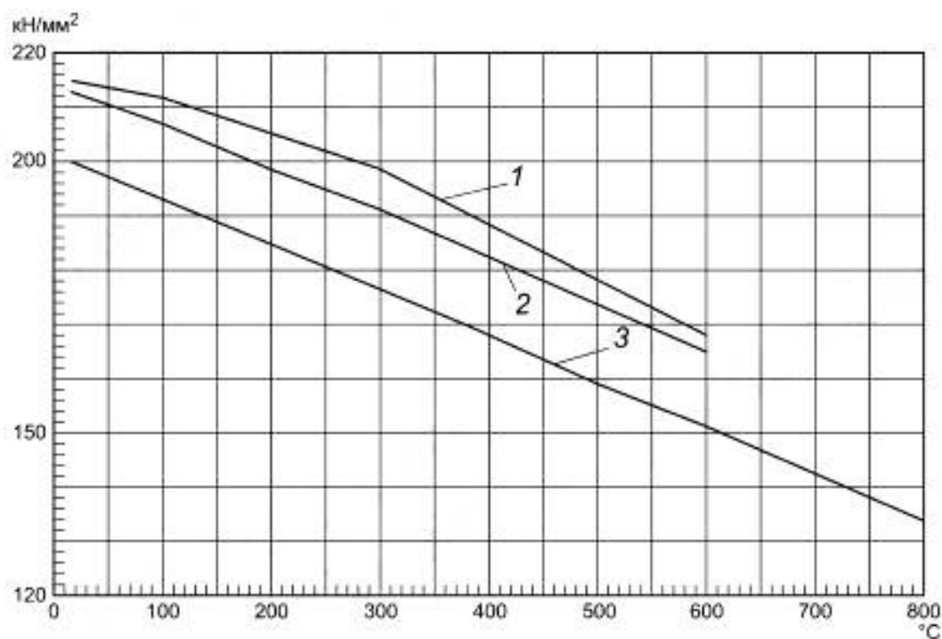
Рисунок D-1 — Модуль упругости
