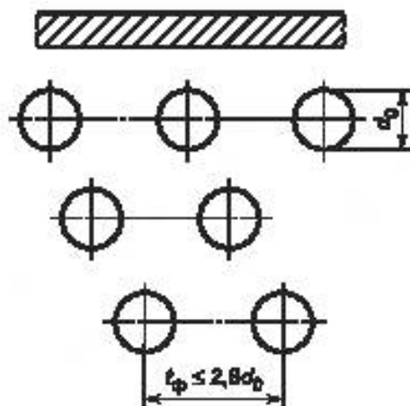
Рисунок 6.1-3 — Элементы, защищенные тремя рядами труб
