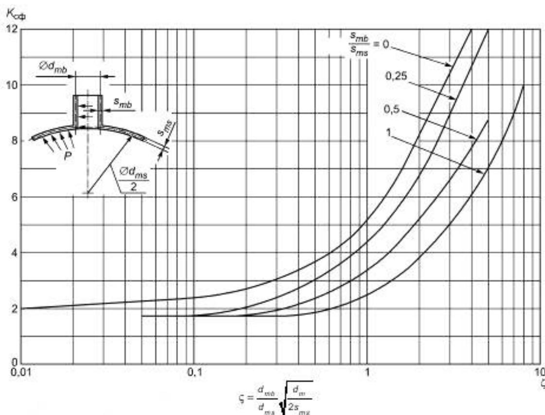
Рисунок 13.4-7, лист 1 — Коэффициент концентрации напряжений K_{сф} для сферических оболочек
