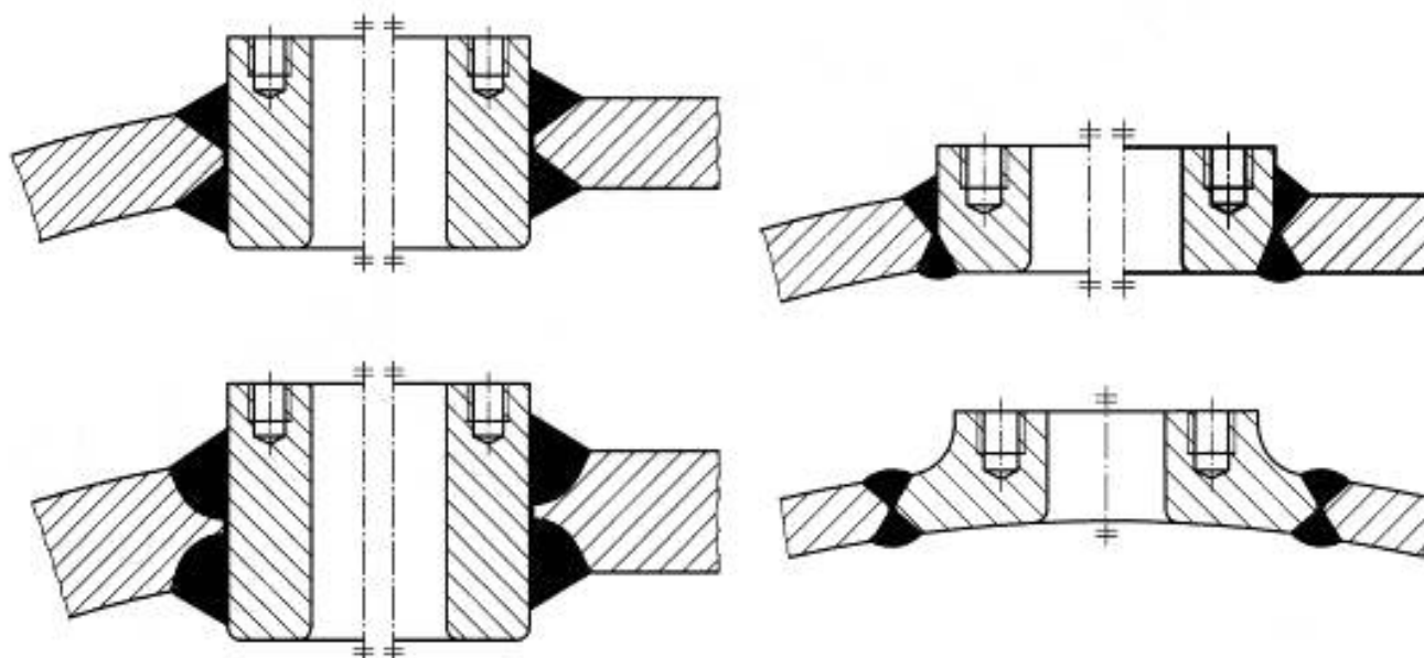
Рисунок 8.4-1 — Типовые примеры приварки усиливающих элементов
