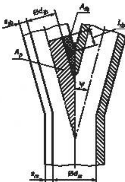
Рисунок 8.3-5 — Эпюра нагрузок для Y-образных развилок
