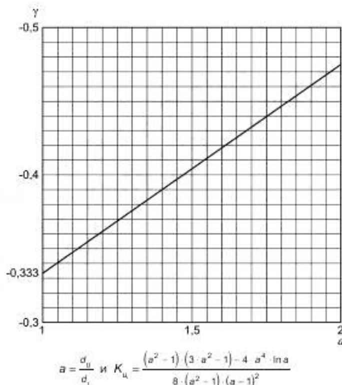
Рисунок 13.4-6 — Коэффициент формы K_u для цилиндрических обечаек
