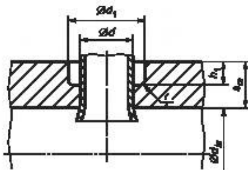
Рисунок 8.2-3 — Профиль отверстия для развальцованных труб
