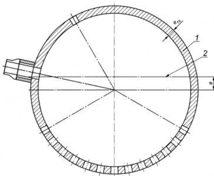
1 — поперечное сечение оболочки; 2 — нейтральная линия
