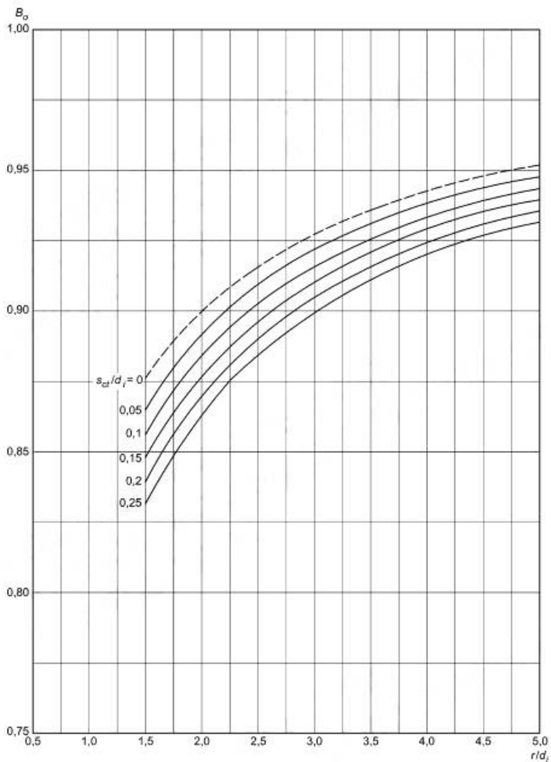
Рисунок А-4 — Расчетный коэффициент B_\sigma для наружной образующей гiba трубы с номинальным внутренним диаметром
