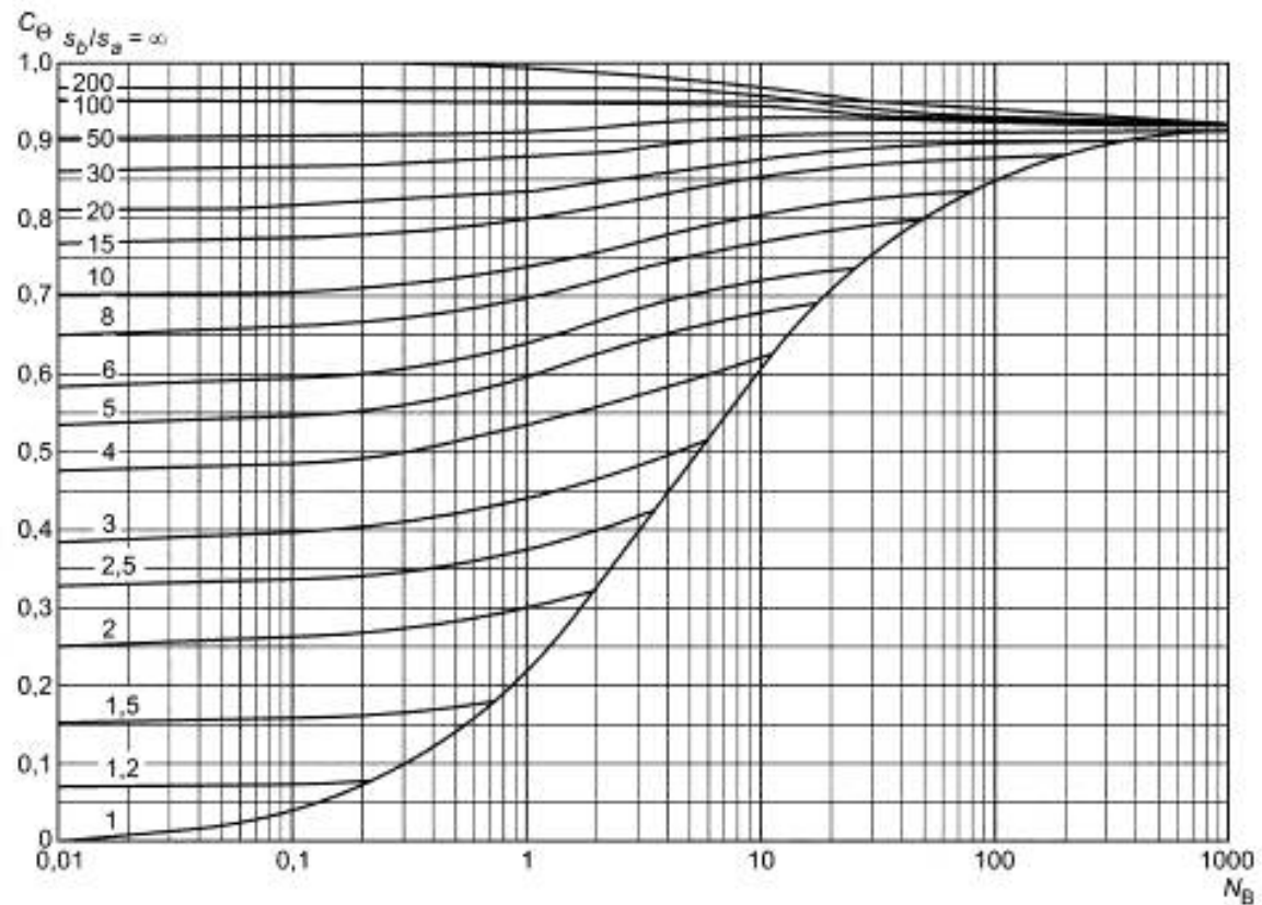
Рисунок 13.3-5 — Коэффициент C_\Theta
