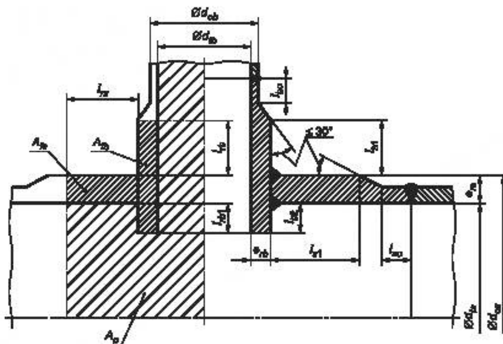
Рисунок 8.1-2 — Усиление обечайки штуцером, вваренным с полным проплавлением
