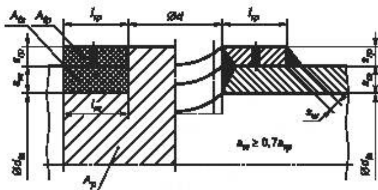
Рисунок 8.1-7 — Отверстие с усиливающей накладкой (допустимо для t_c < 250 °C)
