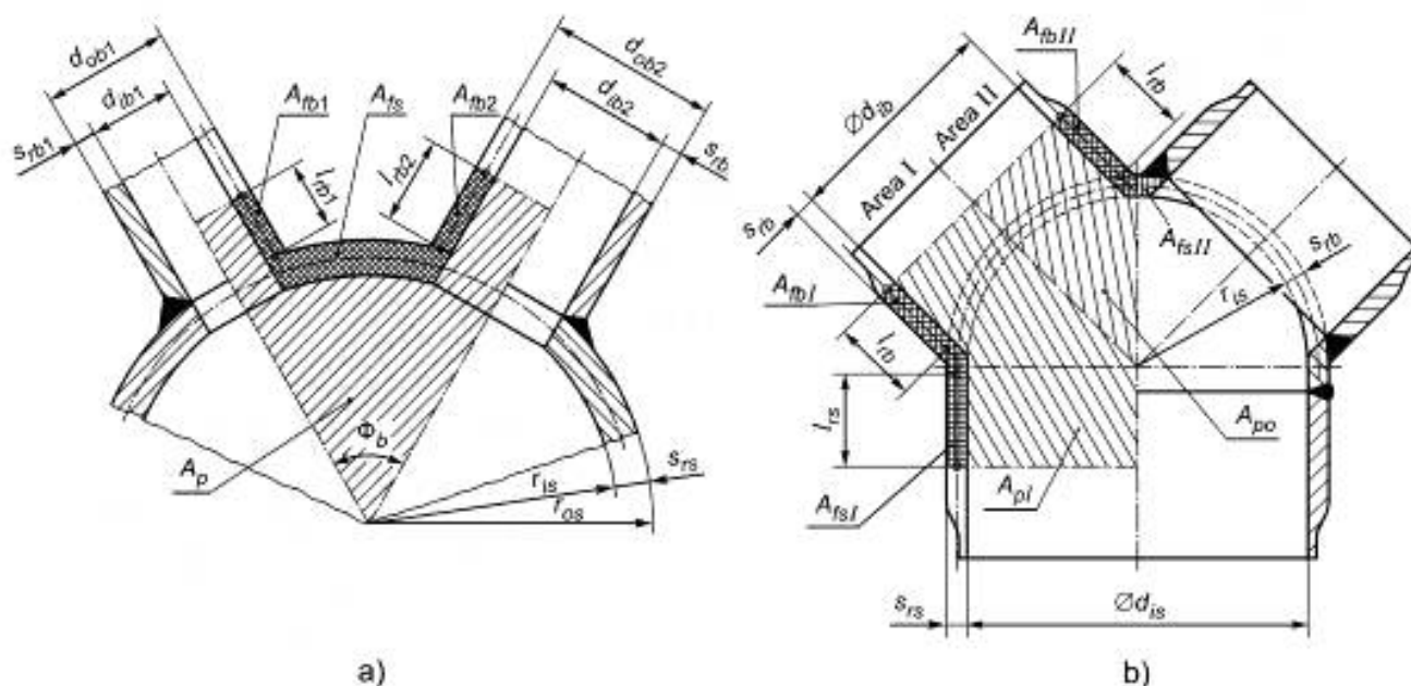
а) смежные штуцера; б) Y-образная развилка
