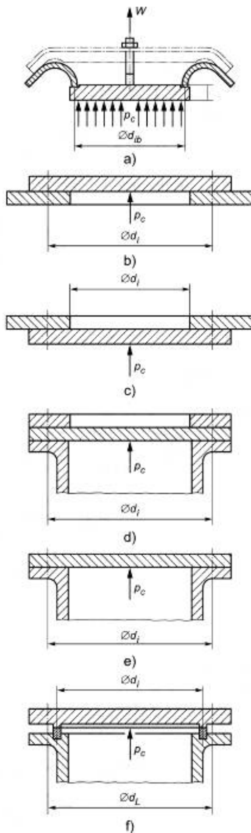
Рисунок 10.4-1 — Плоские съемные заглушки без анкерных связей
