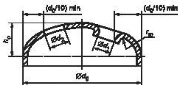
Рисунок 10.2-5 — Отверстия в днищах
