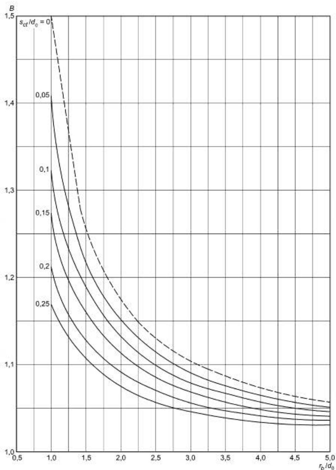
Рисунок А-6 — Расчетный коэффициент B для расчета гибов со стенками равной толщины ( s_{ct} = s_{nto} ) труб с номинальным наружным диаметром
