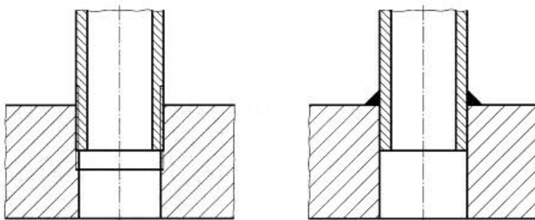
Рисунок 8.5-2 — Соединение на сваренной муфте и резьбовое соединение
