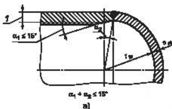
Рисунок 10.2-3 — Полусферическое днище
