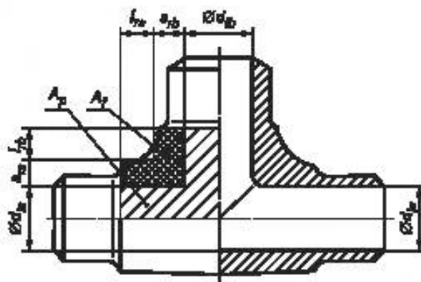
Рисунок 8.3-6 — Кованый и рассверленный тройник
