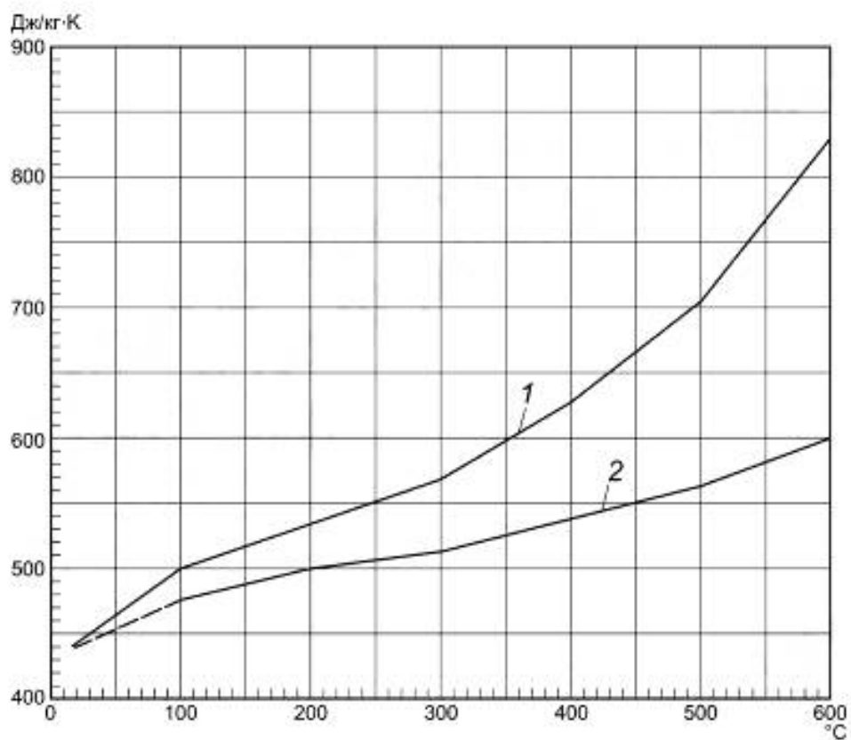
Рисунок D-3b — Теплоемкость сталей группы 6 (12Cr1MoV)
