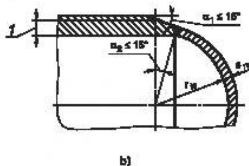
Рисунок 10.2-3 — Полусферическое днище
