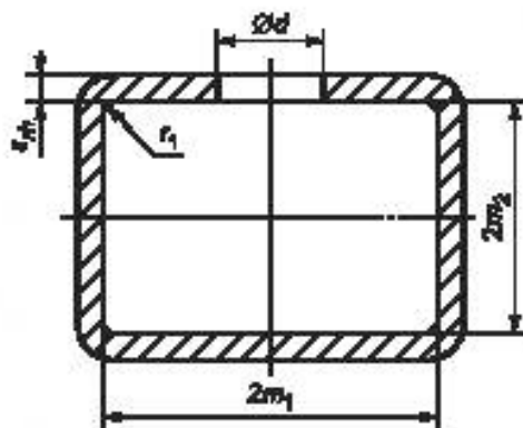
Рисунок 9.2-1 — Символы для прямоугольных коллекторов
