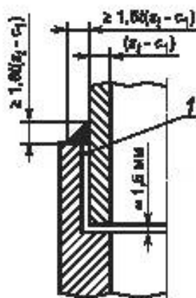
Рисунок 8.5-3 — Шов приварки муфты
