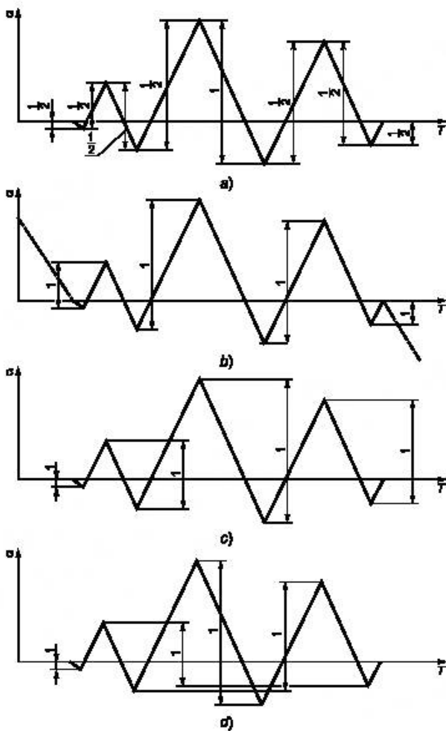
Рисунок В.5 — Варианты оценки величин в ОПГ
