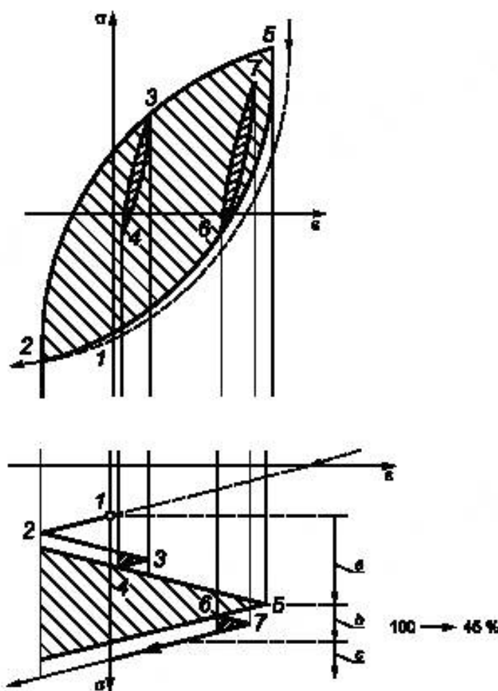
Рисунок В.2 — Схематическое изображение характеристики напряжения — деформации и расчет цикла нагружения
