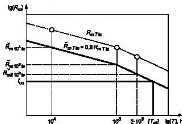
Рисунок А.1 — Диаграмма для определения [T_{эл}]
