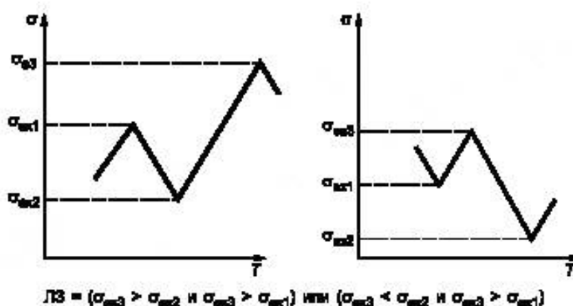
Рисунок В.6 — Критерий для расчета цикла нагрузки с использованием метода с)
