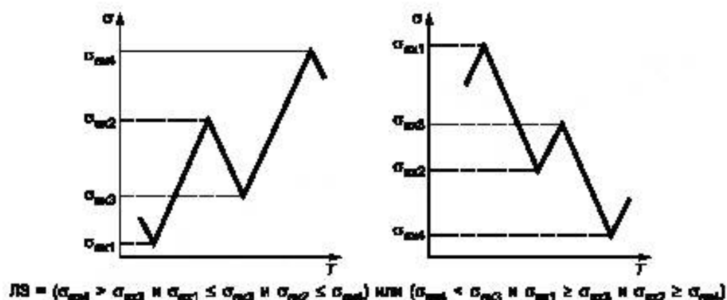
Рисунок В.3 — Критерий для цикла нагружения с диапазоном \Delta\sigma_{\text{ex}} = |\sigma_{\text{ex}2} - \sigma_{\text{ex}3}| с применением метода дождевого потока и метода парной амплитуды
