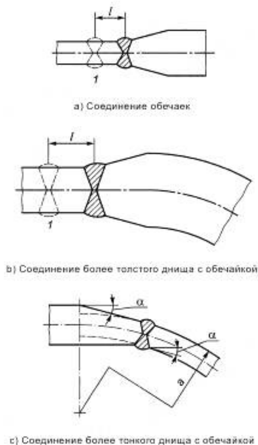
а) Соединение обечайек б) Соединение более толстого днища с обечайкой в) Соединение более тонкого днища с обечайкой \alpha \leq 15^\circ , см. также рисунок 10.2-3 ГОСТ Р 55682.3; а — R_f или r_f (радиус кривизны); l — расстояние между швами; 1 — положение сварного шва
