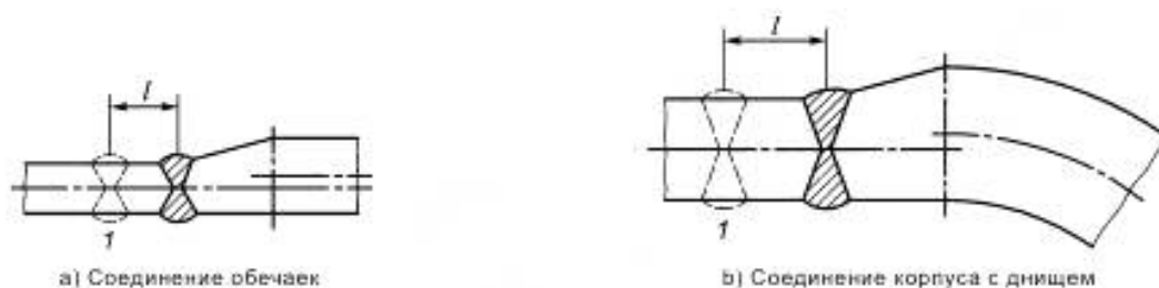
Рисунок 8.9-1 — Стыковые швы листов разной толщины с переходом осей (средних линий)
