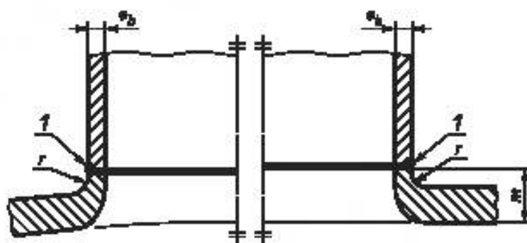
Рисунок В.2 — Примеры присоединения труб к отверстиям с наружной горловиной
