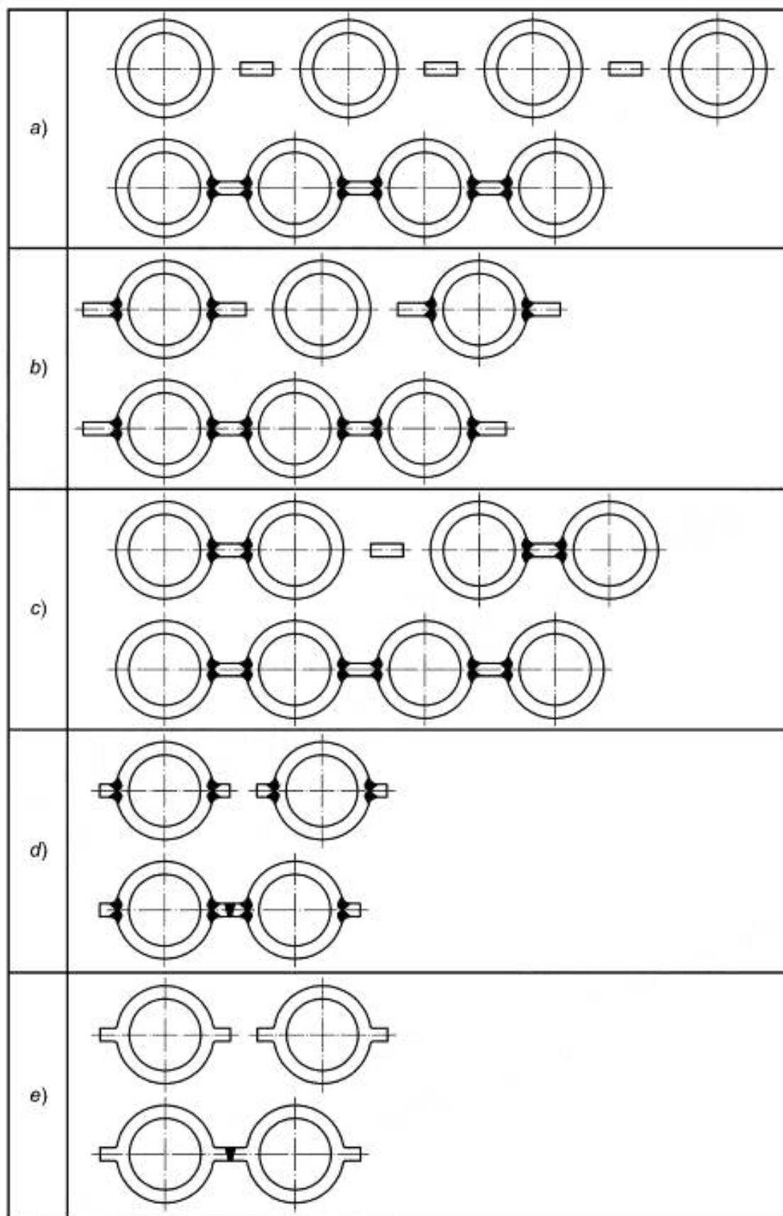
Рисунок С.1 — Примеры конструкций мембранных панелей
