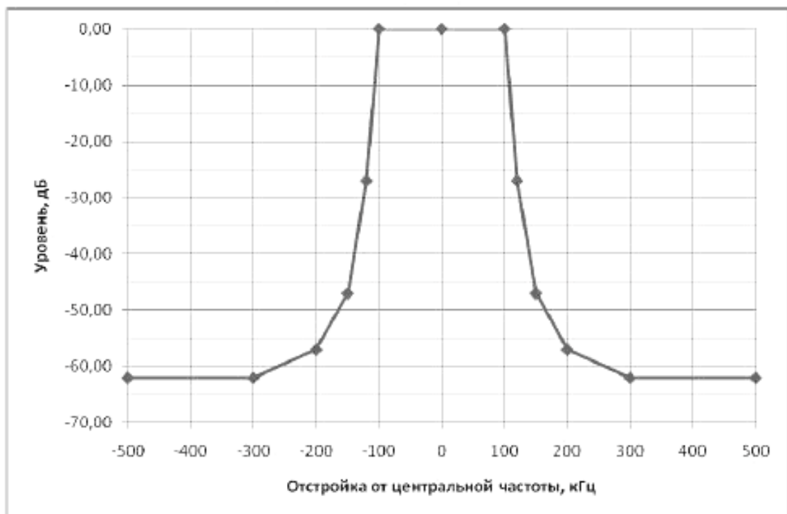
Рисунок 2 – Маска огибающей внеполосных радиколебаний для ширины полосы частот 200 кГц
