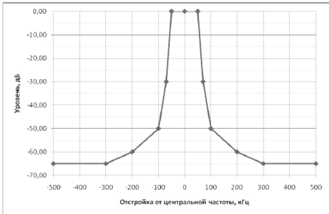
Рисунок 1 – Маска огибающей внеполосных радиколебаний для ширины полосы частот 100 кГц
