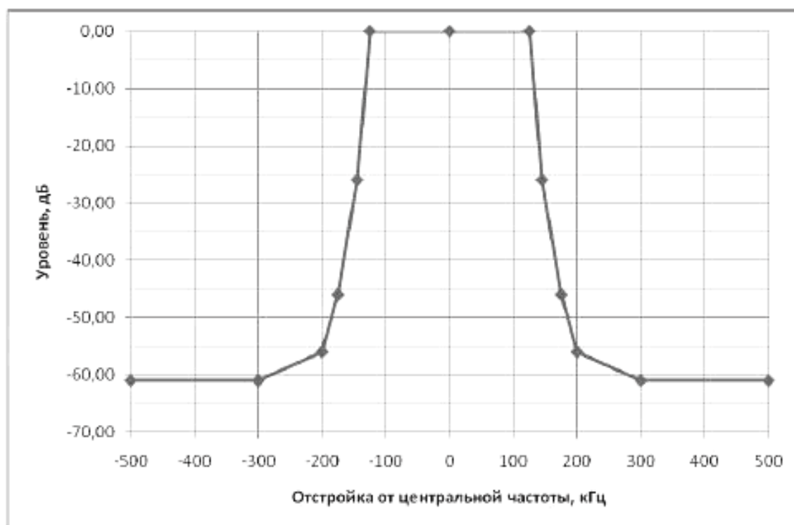
Рисунок 3 – Маска огибающей внеполосных радиополюбов для ширины полосы частот 250 кГц
