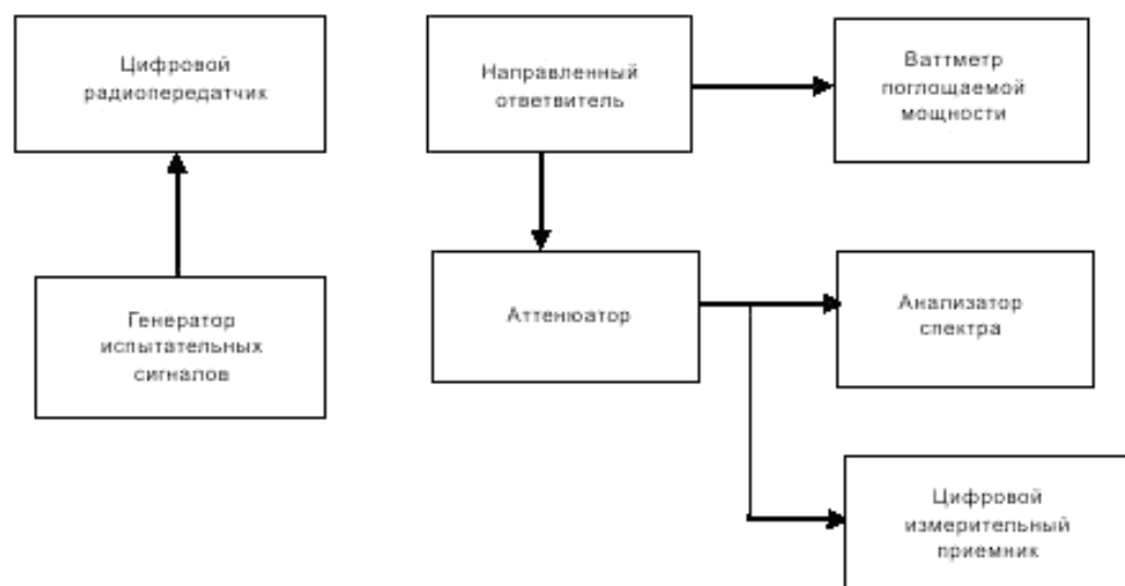
Рисунок 2 - Структурная схема для измерения параметров цифровых радиопередатчиков
