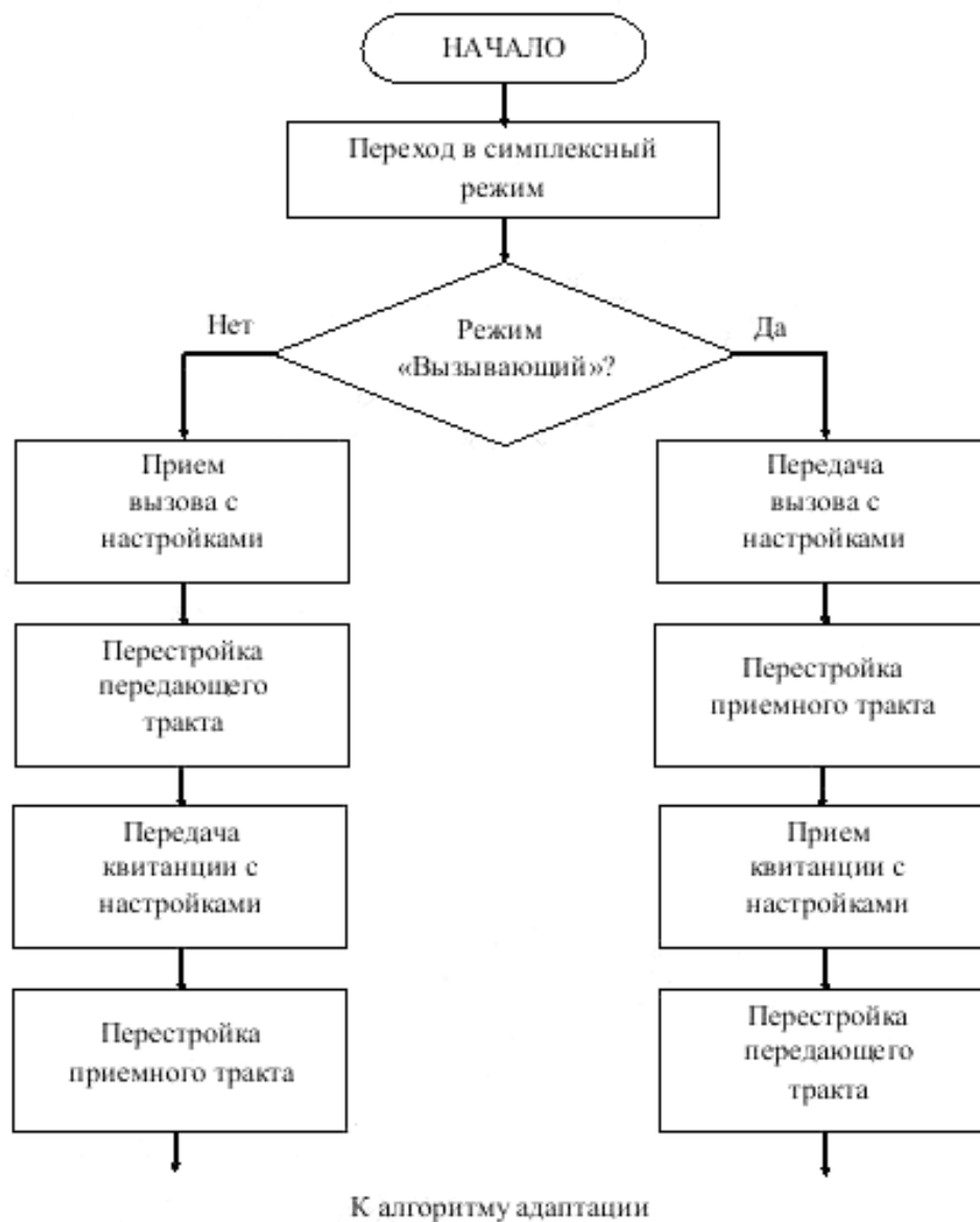
Рисунок 3 – Блок-схема алгоритма перехода в дуплексный режим
