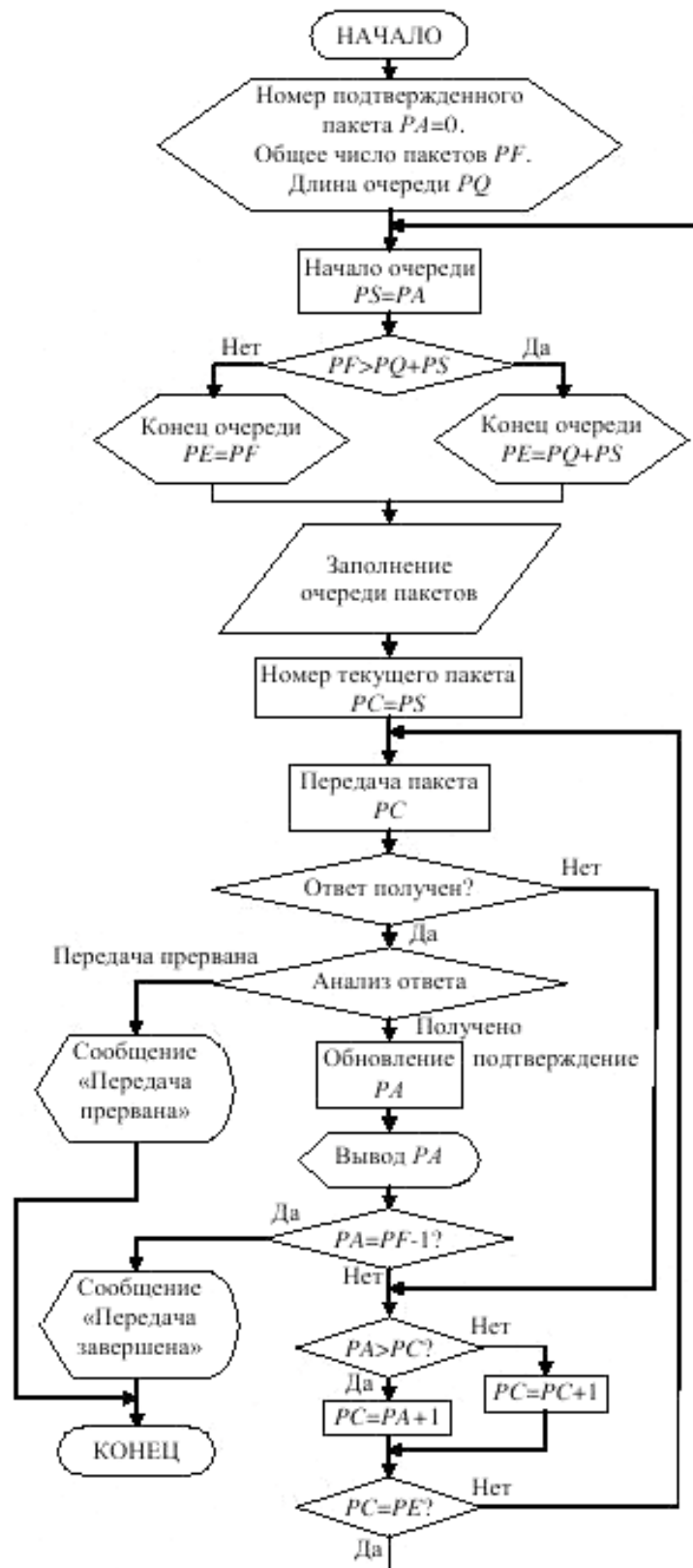
Рисунок 7 – Блок-схема алгоритма процесса передачи данных файла
