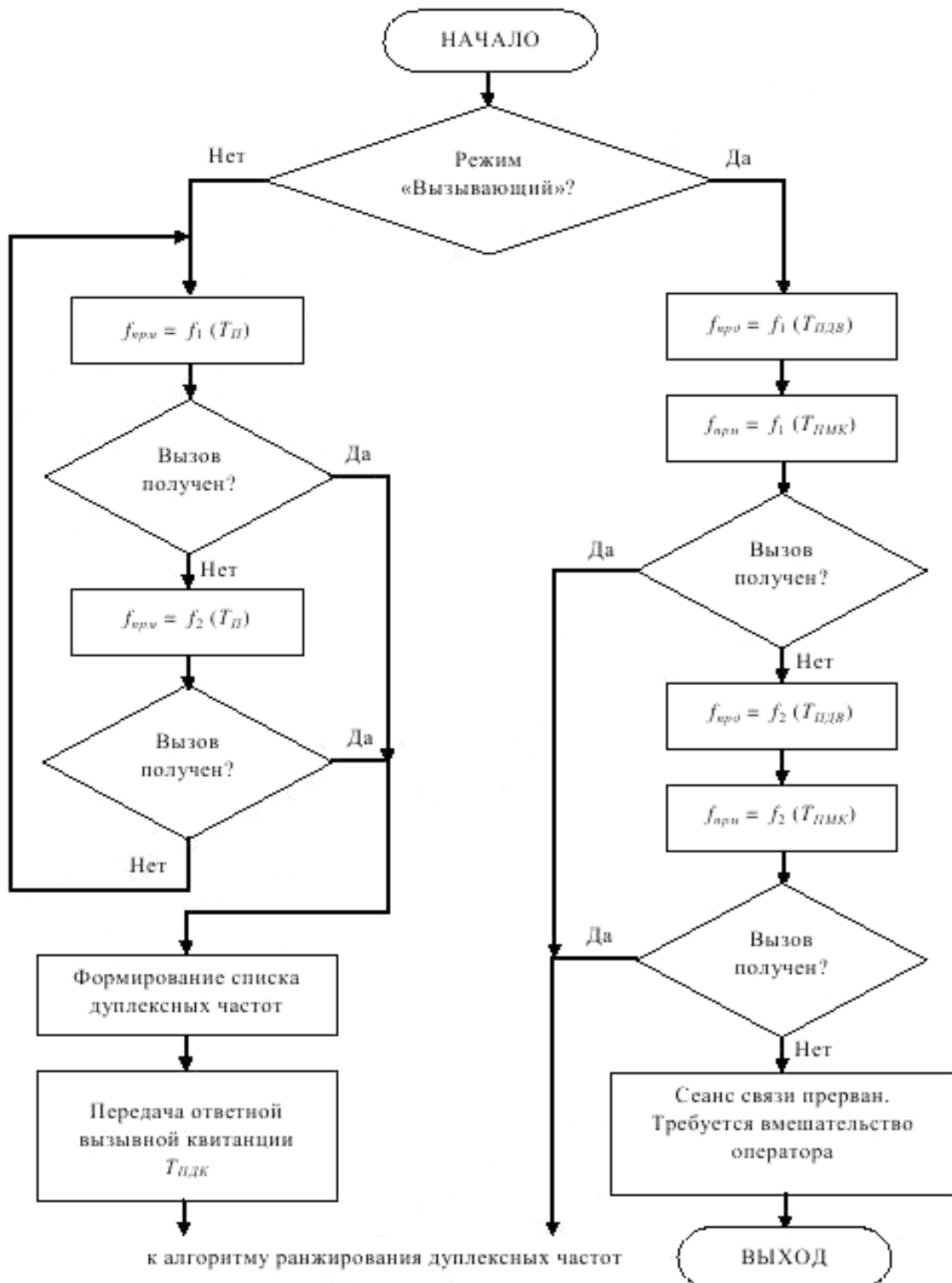
Рисунок 1 – Блок-схема алгоритма вхождения в связь
