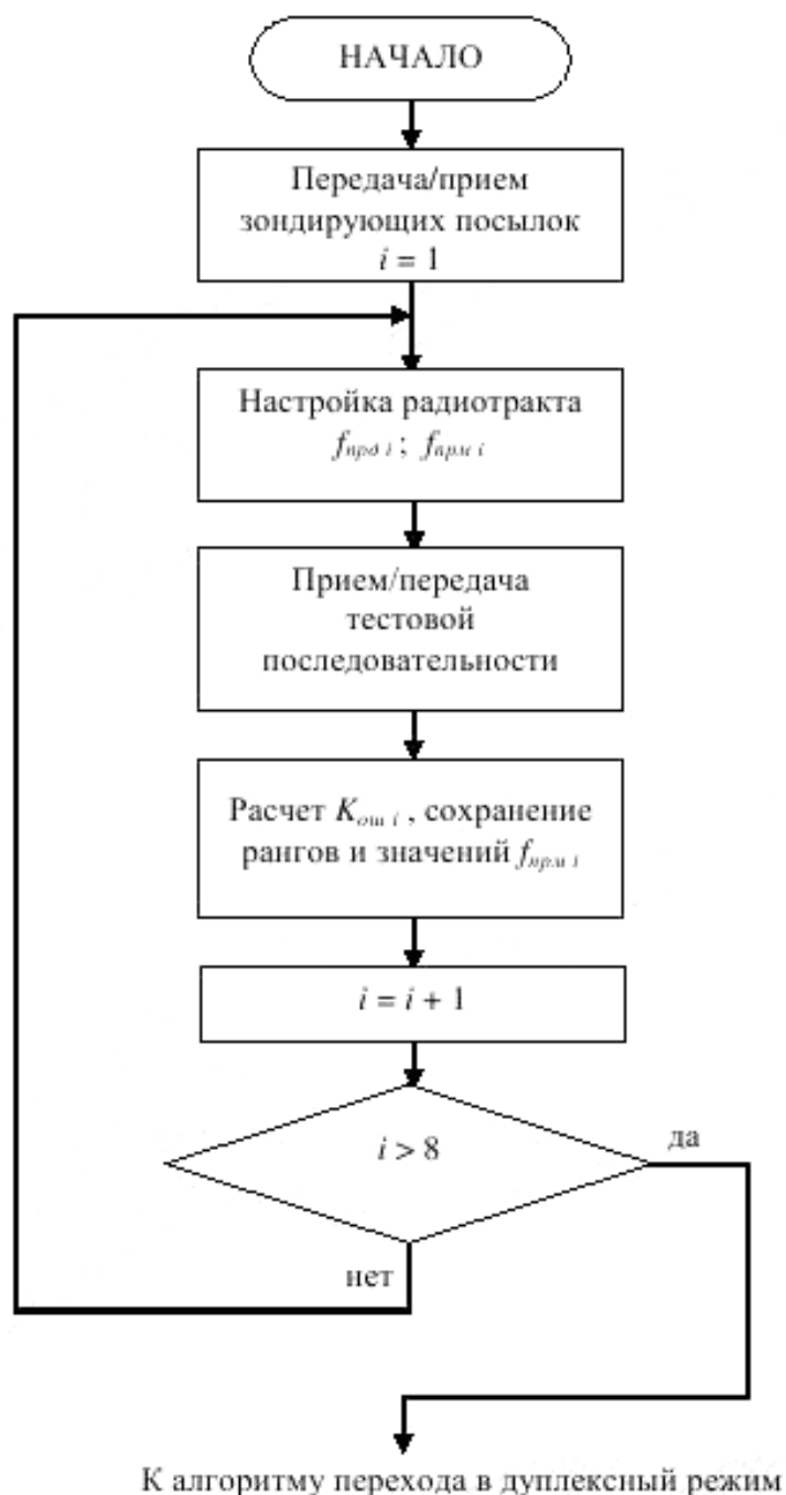
Рисунок 2 – Блок-схема алгоритма ранжирования частот радионаправления
