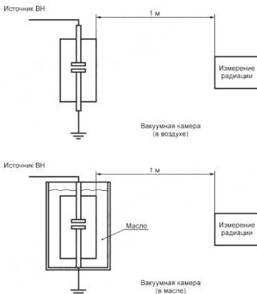
Рисунок 3 — Расположение дозиметра при испытаниях
