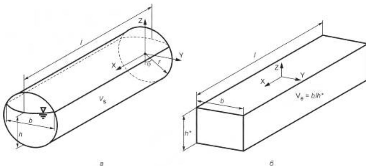
Рисунок 12 — Модель горизонтального цилиндрического сосуда с жидкостью при воздействии в продольном направлении ( h_e^* , h_1^* )
