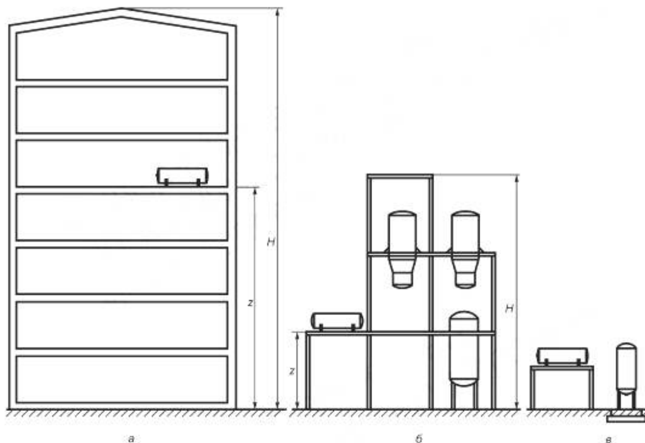
Рисунок 1 — Варианты установки сосуда
