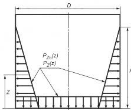
Рисунок 10 — Гидродинамическое давление на стенки и днище от сейсмического воздействия в вертикальном направлении
