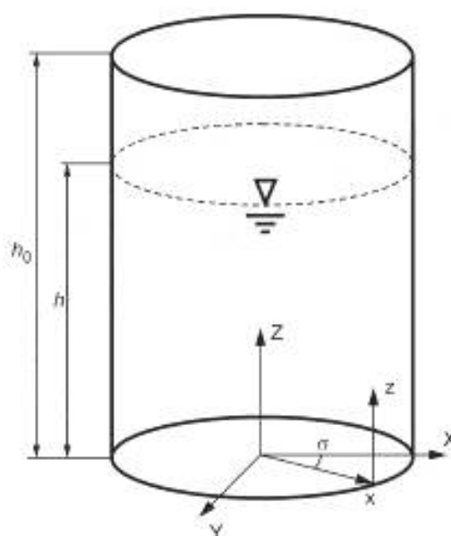
Рисунок 2 — Модель цилиндрического сосуда с жидкостью
