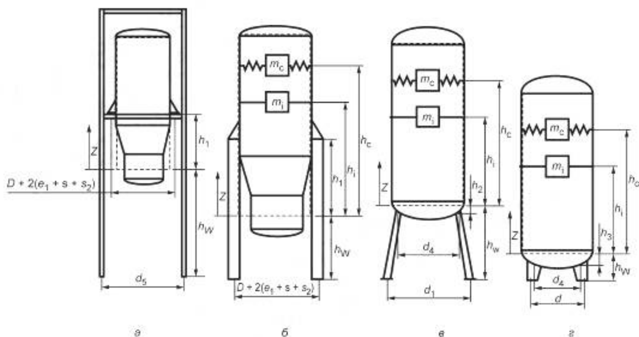
Рисунок 8 — Вертикальный сосуд
