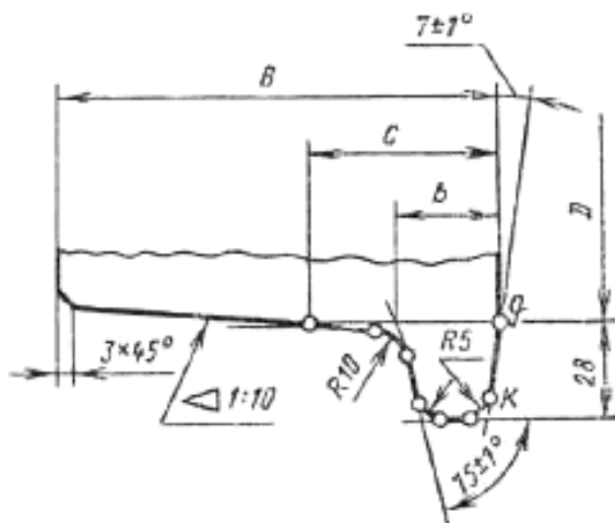
Рисунок Б.1 – Профиль катания обода
