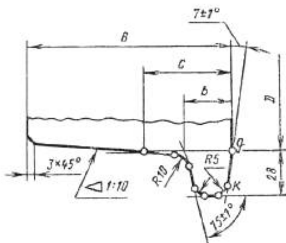
Рисунок Б.1 – Профиль катания обода
