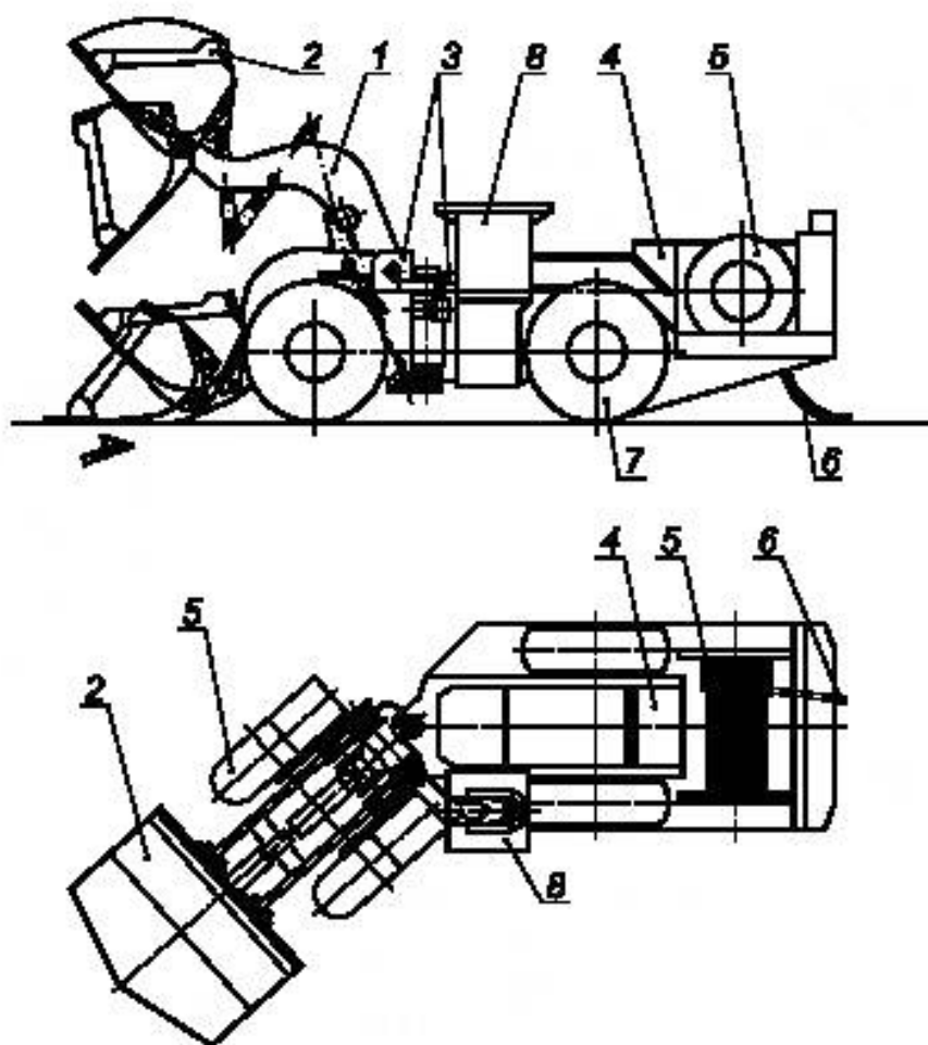
1 — манипуляционное устройство; 2 — ковш; 3 — шарнирно сочлененная рама; 4 — электрический привод; 5 — кабельный барабан; 6 — силовой питающий кабель; 7 — ходовая часть; 8 — кабина
