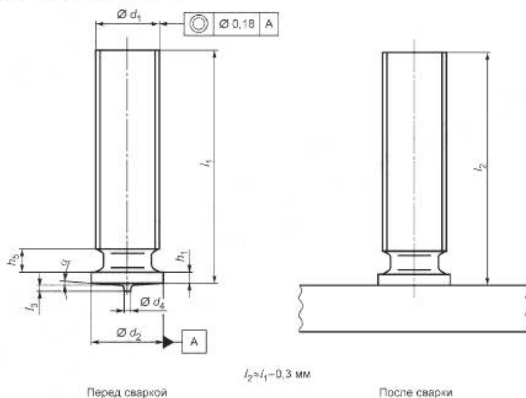
Рисунок 9 — Шпилька с резьбой (PT)
