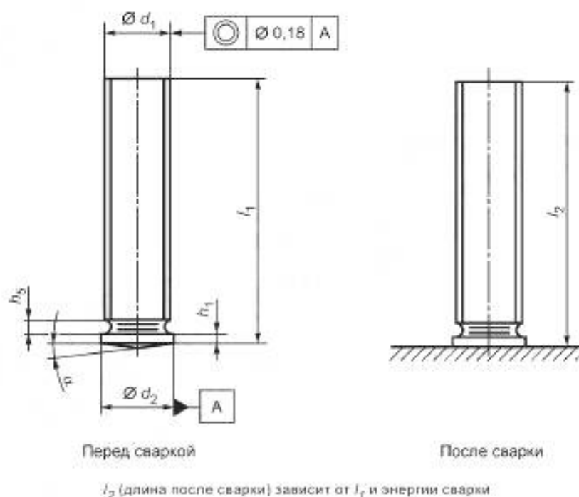
Рисунок 6 — Шпилька с резьбой с фланцем (PS)
