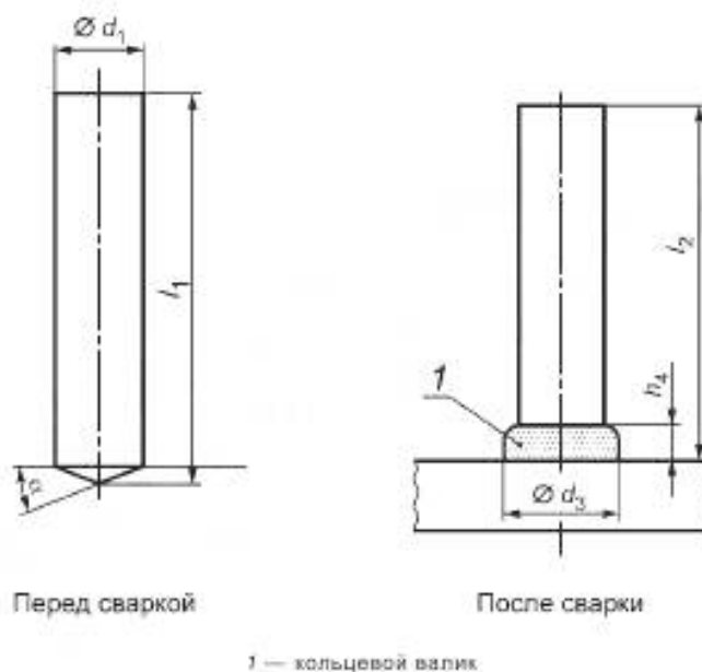
Рисунок 3 — Шпилька без резьбы (UD)
