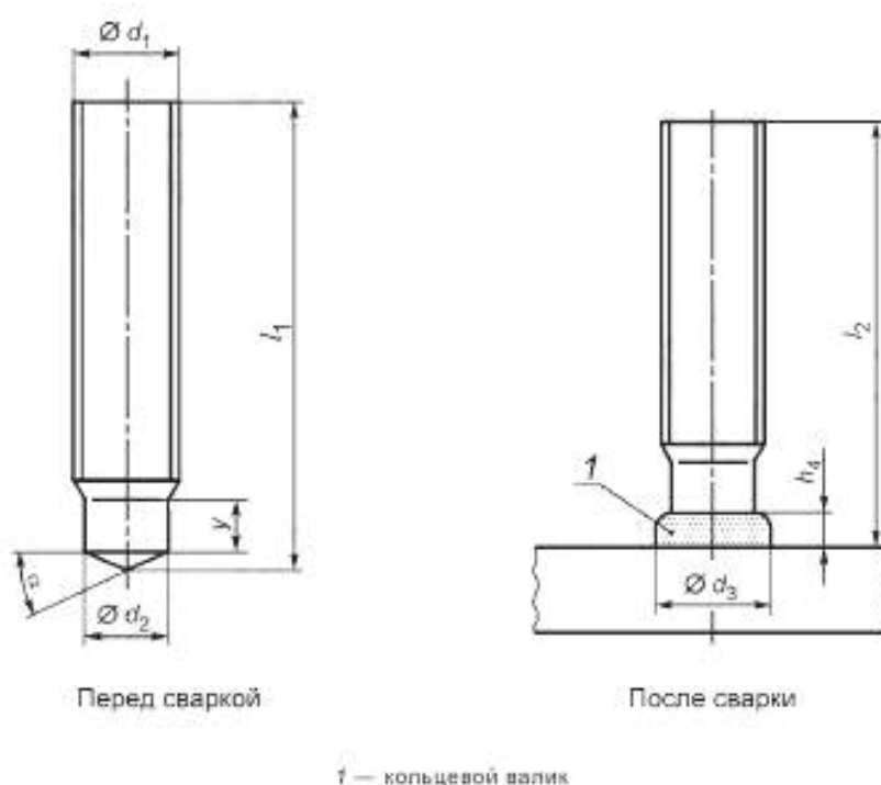
Рисунок 2 — Шпилька с резьбой с редуцированным стержнем (RD)
