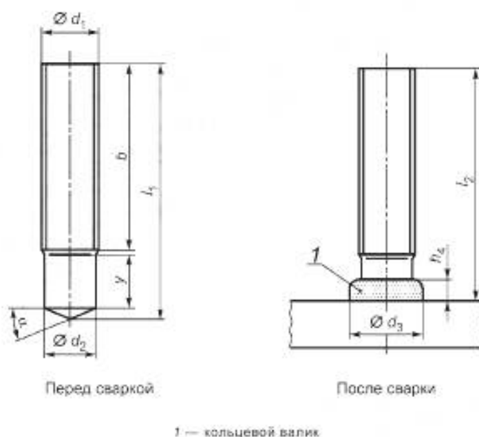
Рисунок 1 — Шпилька с резьбой (PD)
