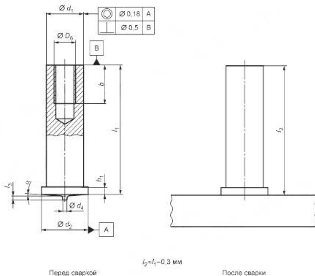
Рисунок 11 — Шпилька с внутренней резьбой (IT)
