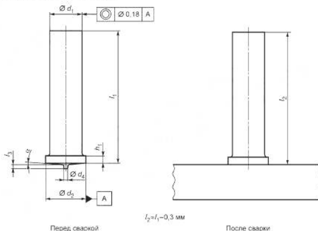
Рисунок 10 — Шпилька без резьбы (UT)
