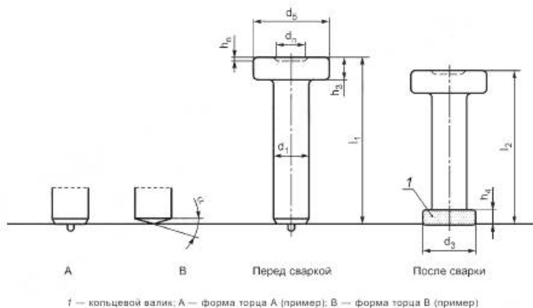
Рисунок 5 — Шпилька-упор (SD)
