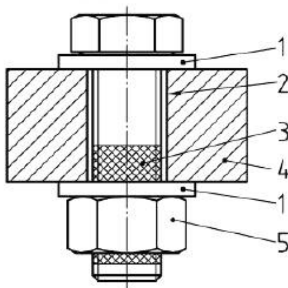
Рисунок 3 – Схема испытания с контрольной плитой
