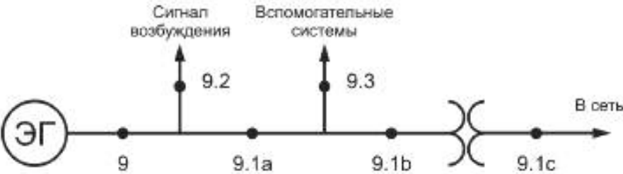
Рисунок 3 — Определение точек для измерения электрической мощности
