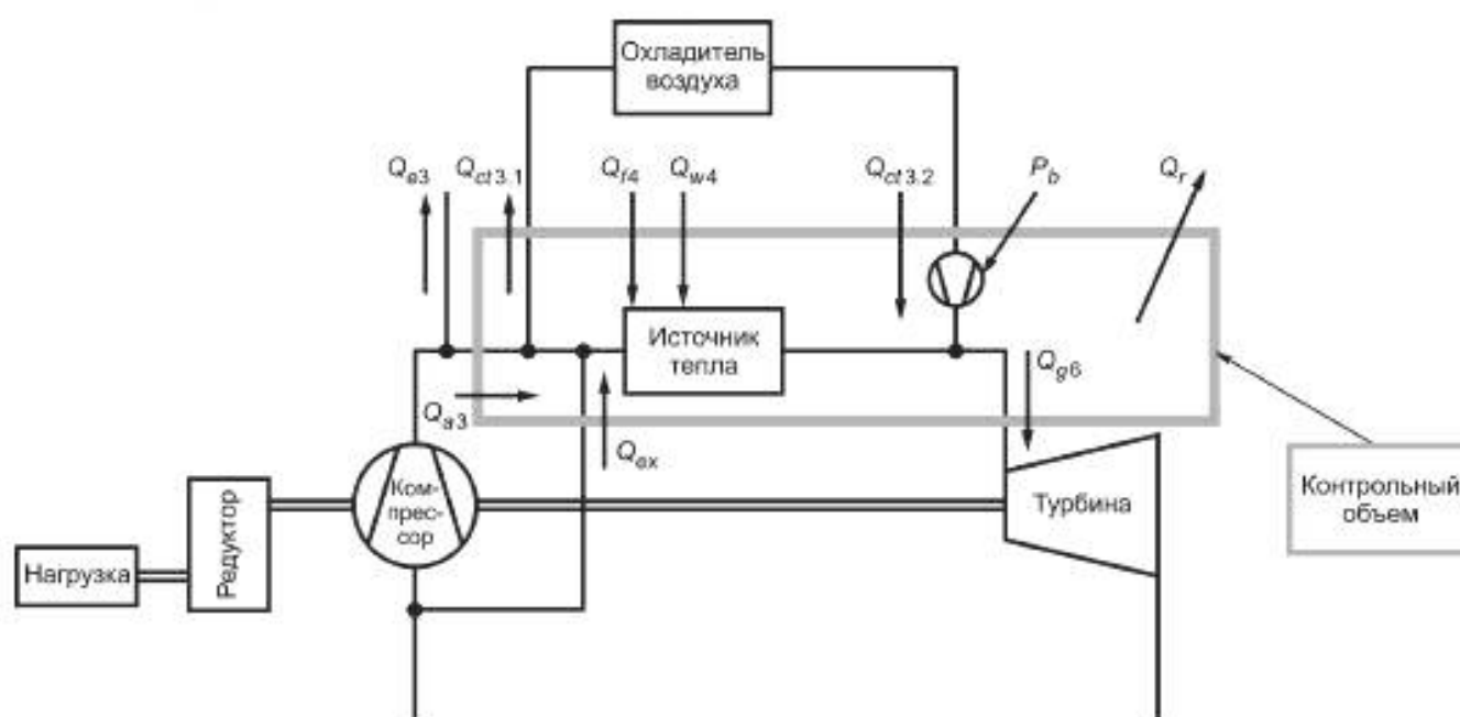
Рисунок 5 — Контрольный объем для энергетического баланса камеры сгорания
