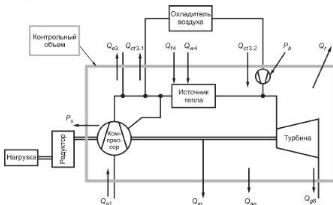
Рисунок 4 — Контрольный объем для энергетического баланса системы
