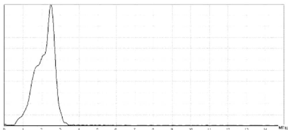
Рисунок 2 – Амплитудный спектр для сильно корродированной резьбы.
