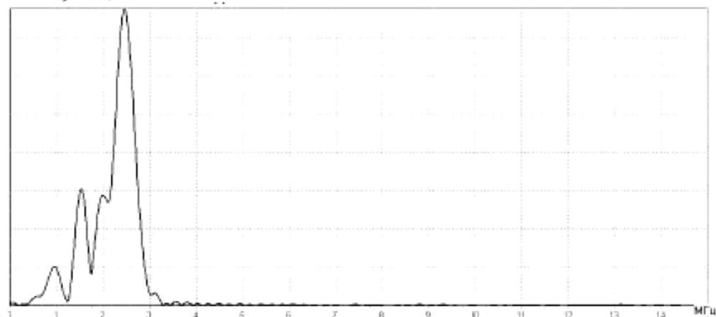
Рисунок 1 – Амплитудный спектр для резьбы СОП.
