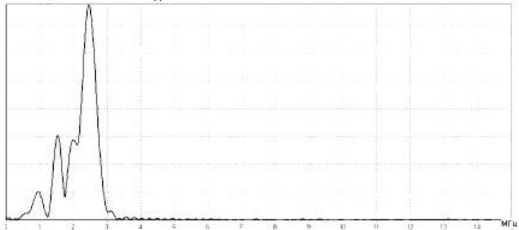
Рисунок 1 – Амплитудный спектр для резьбы СОП.
