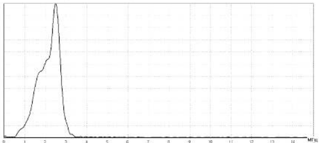
Рисунок 2 – Амплитудный спектр для сильно корродированной резьбы.
