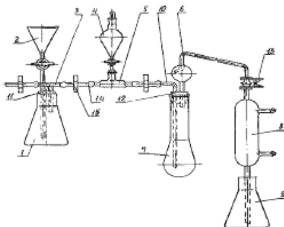
1 – коническая колба вместимостью 500 см 3 ; 2 – воронка с краном; 3 – Т-образная трубка; 4 – делительная воронка вместимостью 100 см 3 ; 5 – переходник; 6 – каплеуловитель; 7 – колба Кельдаля вместимостью 250 см 3 ; 8 – шариковый холодильник; 9 – приемная мерная колба вместимостью 50 см 3 ; 10 – изогнутая трубка; 11, 12 – резиновые пробки; 13, 15 – зажим; 14 – резиновые трубки
