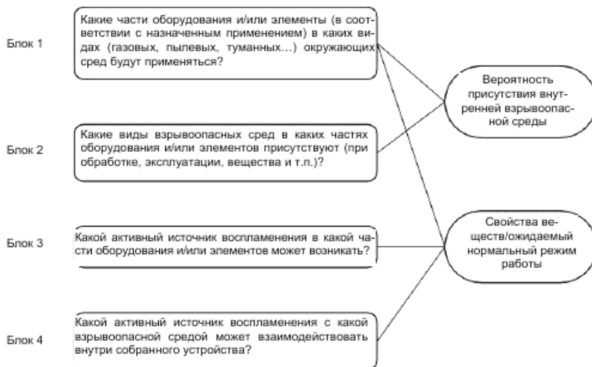
Рисунок 2 — Выявление опасностей воспламенения
