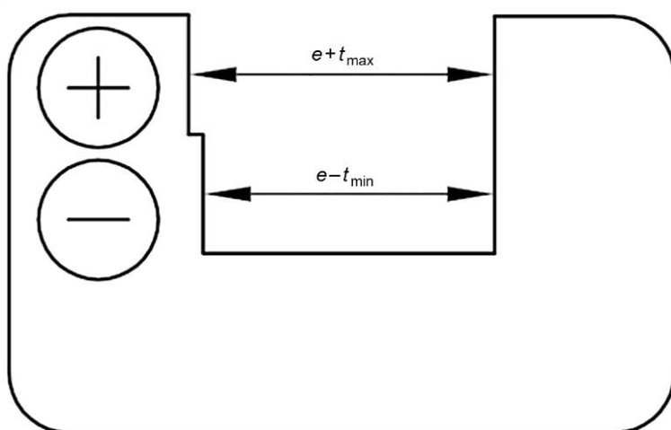
Рисунок Е.6 — Шаблон контроля толщины шейки рельса
