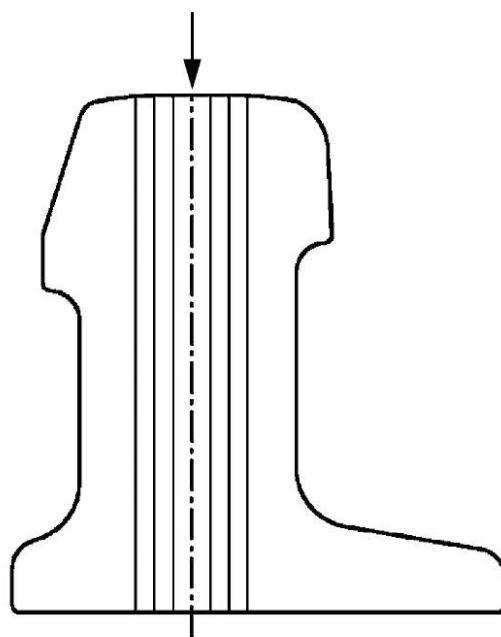
Рисунок В.1 — Схема прозвучивания приемо-сдаточных испытаниях методом «А»
