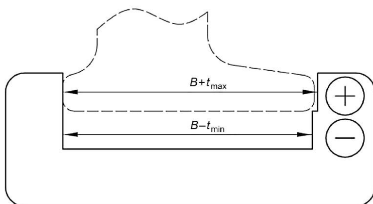
Рисунок Е.5 — Шаблон контроля ширины подошвы рельса
