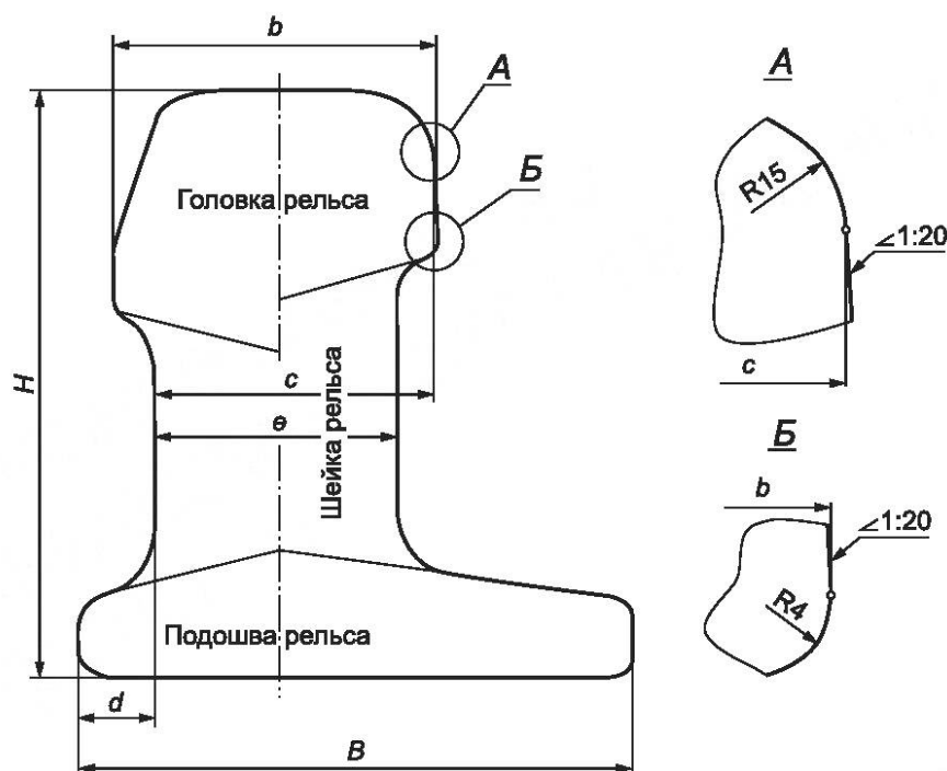
Рисунок 4 — Основные (контролируемые) размеры поперечного сечения рельсов
