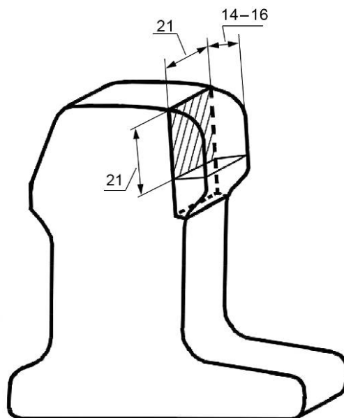
Рисунок 5 — Схема вырезки шлифа для контроля неметаллических включений
