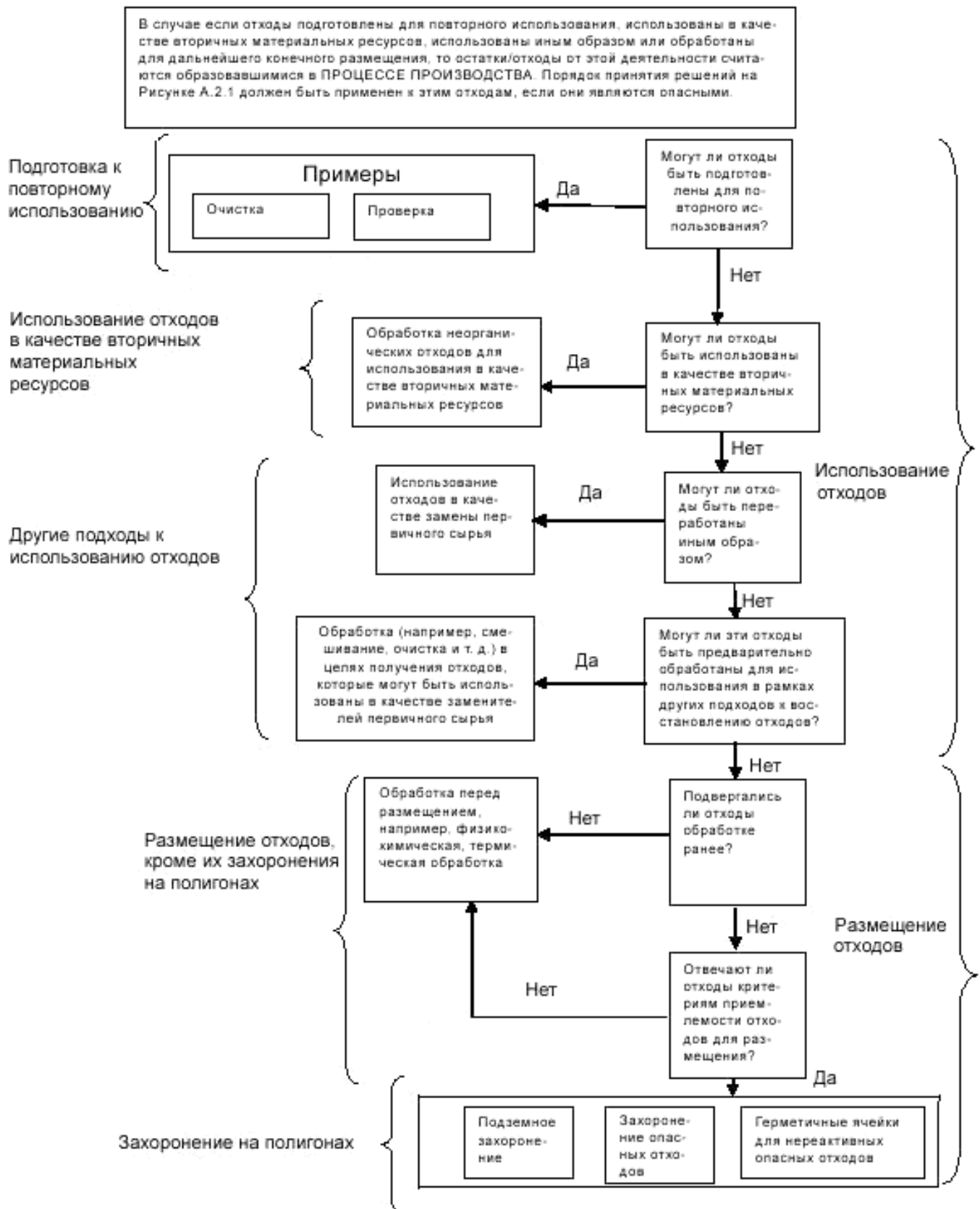
Рисунок Б.5.1 — Порядок принятия решений при обращении с неорганическими отходами
