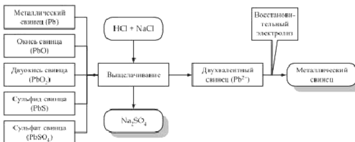
Рисунок 4 - Электрохимические процессы при гидрометаллургическом производстве свинца
