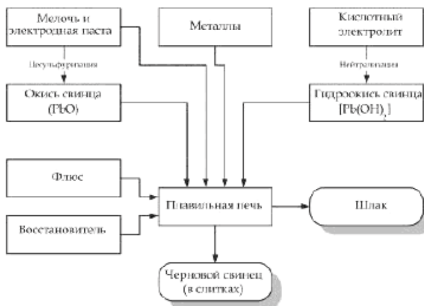
Рисунок 3 Технологическая схема выплавки свинца.
