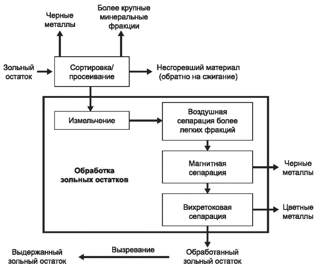
Рисунок 1 — Технологическая схема примера процесса обработки зольного остатка мусоросжигательного завода, включая этапы механического разделения
