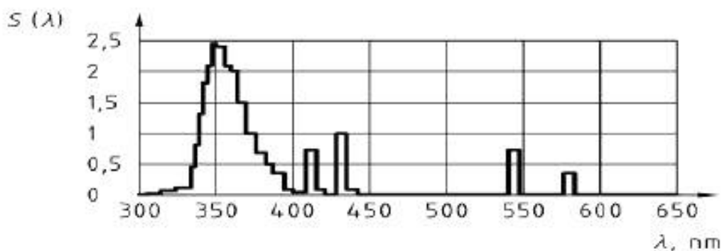
Рисунок В.1 – Спектральное распределение лампы
