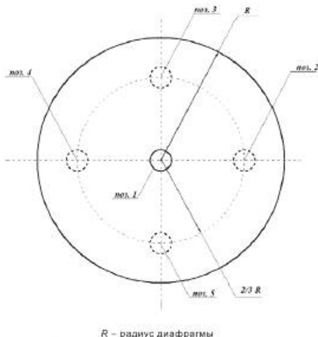
Рисунок В.7 — Расположение круглой диафрагмы относительно входного отверстия приемной поверхности фотометрической головки
