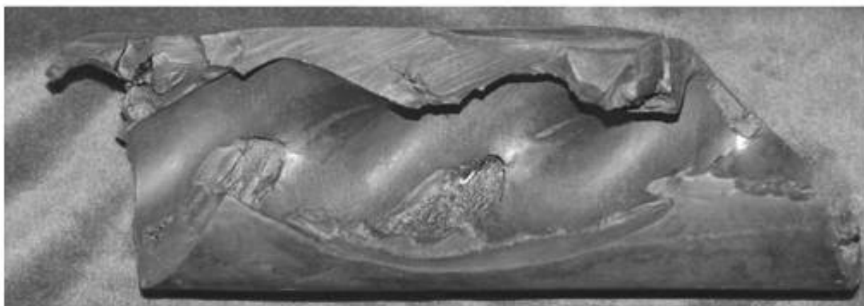
Рисунок 1.8 — Расслоение статора
