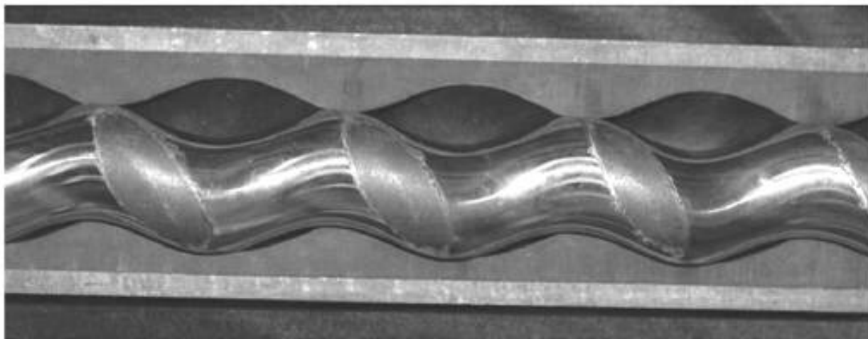
Рисунок 1.2 — Изношенный ротор
