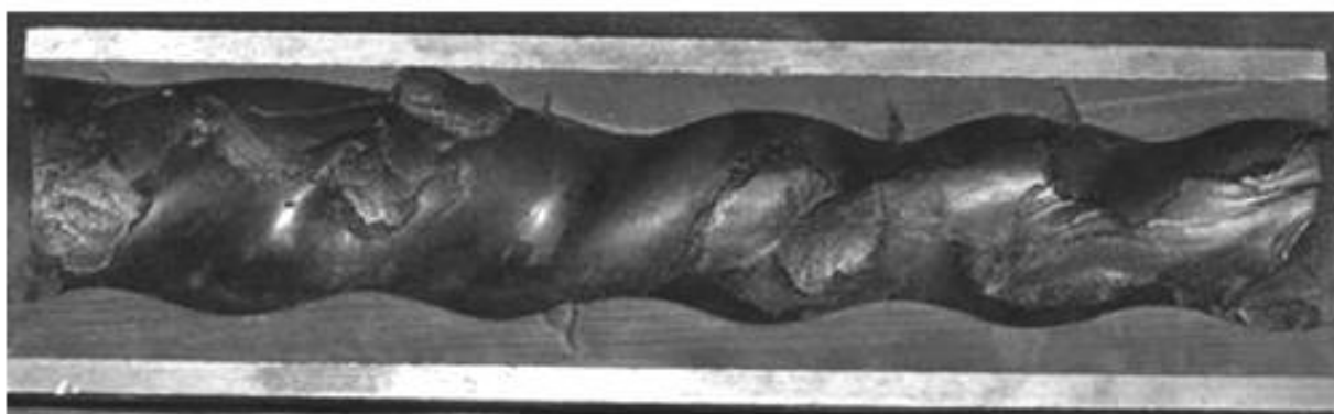
Рисунок 1.10 — Рванный /разбитый статор
