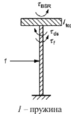
Рисунок В.1 — Насос с заклинившим рабочим органом
