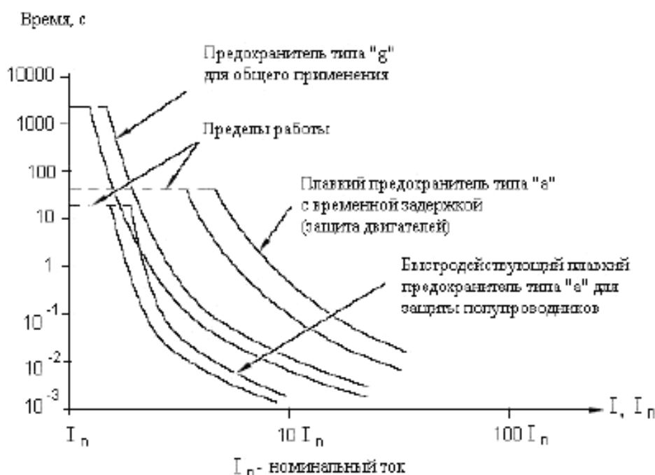
Рисунок А.1 – Сравнение времятоковых характеристик высоковольтных предохранителей типа «а» и «g»
