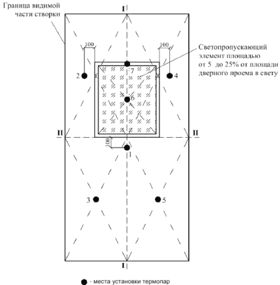
Рисунок А.2 - Схема установки термодпар на необогреваемой поверхности створок одностворчатой распашной и горизонтально-раздвижной двери бокового открывания со светопропускающим элементом створок свыше 5 до 25% от площади дверного проема в свету
