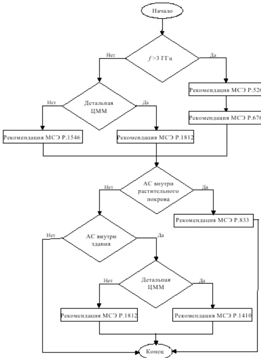
Рисунок 4.3 - Блок-схема алгоритма расчета ослабления радиосигнала на трассе
