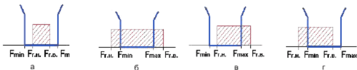
Рисунок 9.1 — Положение полосы частот радиоизлучения на гармонике относительно полосы пропускания приемника
