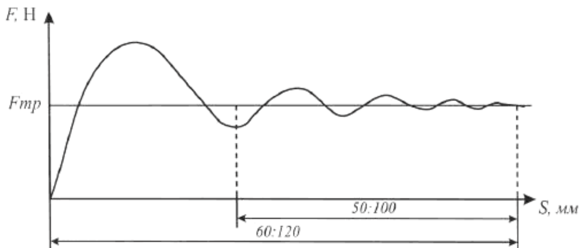
Рисунок 4 - Принципиальная схема зависимости сдвигающей силы от перемещения
