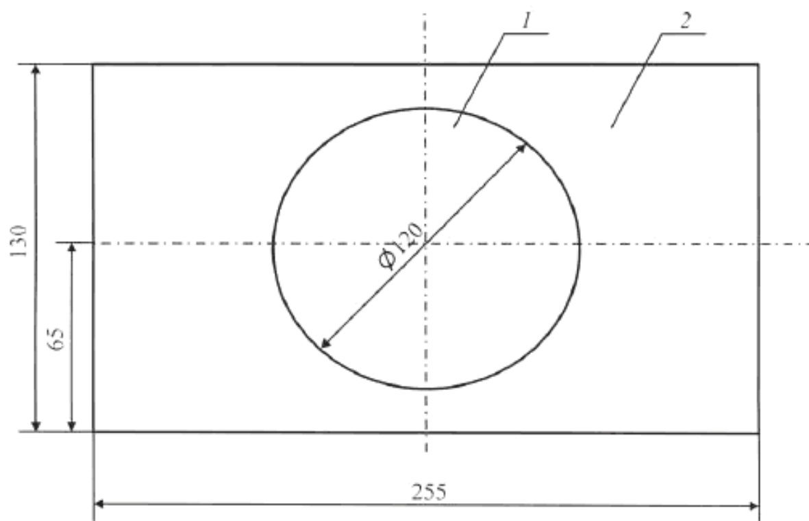
Рисунок 3 – Схема крепления рабочего эталона подошвы ноги человека
