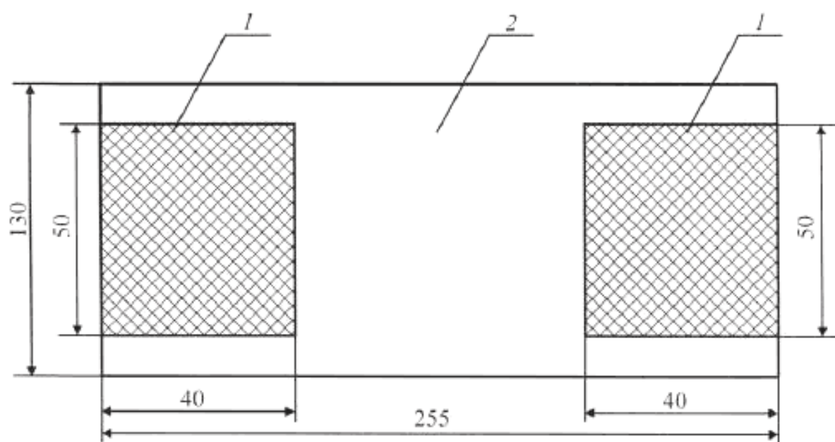
Рисунок 2 – Схема крепления рабочего эталона подошвы обуви
