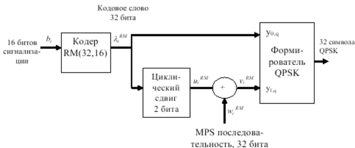
Р и с у н о к 20 – Устойчивый (робастный) заголовок FECFrame
