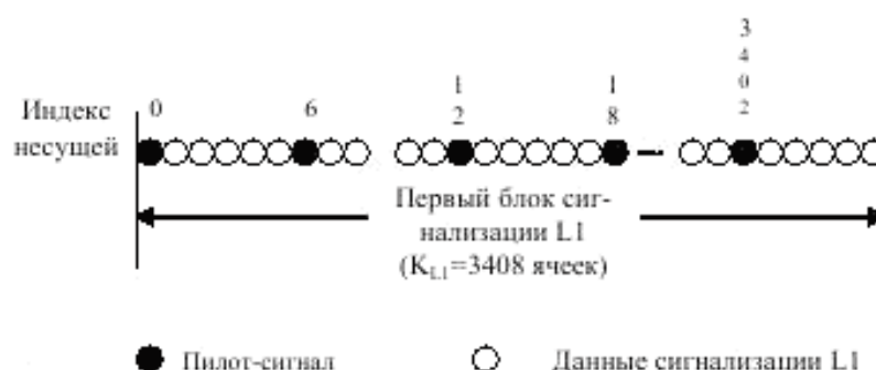
Р и с у н о к 37 – Блок сигнализации L1
