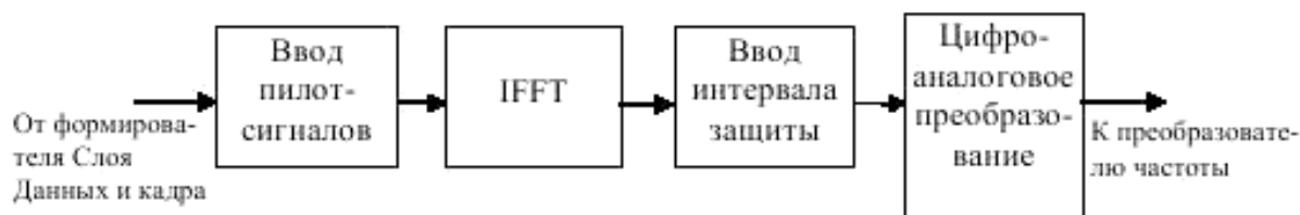
Р и с у н о к 5 – Блок-схема подсистемы формирования сигнала OFDM
