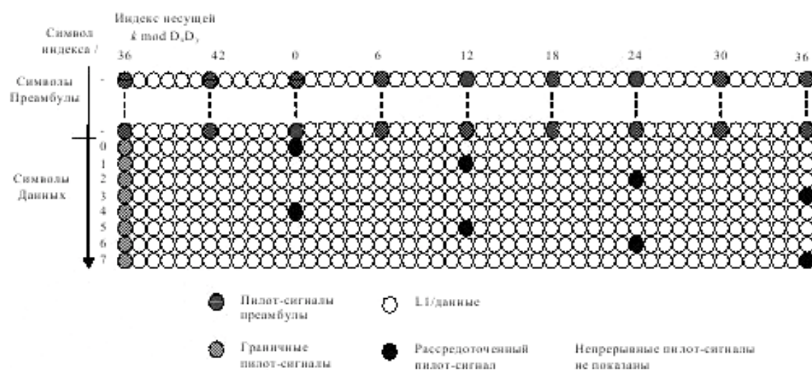
Р и с у н о к Е.4 – Распределенный пилот-сигнал для GI 1/64 с низкочастотной границей k \bmod D_x D_y = 36
