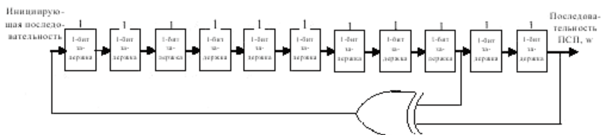
Р и с у н о к 34 – Формирование псевдослучайной последовательности
