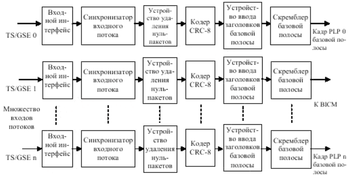
Р и с у н о к 2 – Блок-схема подсистемы адаптации множества входных потоков
