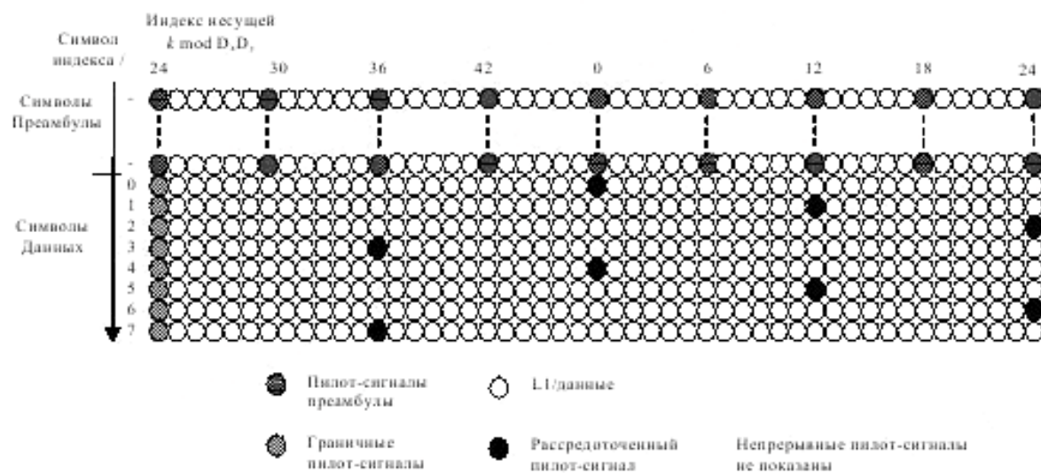
Р и с у н о к Е.3 – Рассредоточенный пилот-сигнал для GI 1/64 с низкочастотной границей k \bmod D_x D_y = 24
