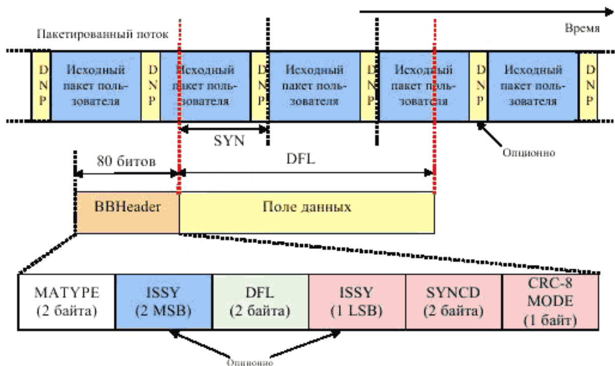
Р и с у н о к 10 – Формат потока TS на выходе адаптера режима HEM
