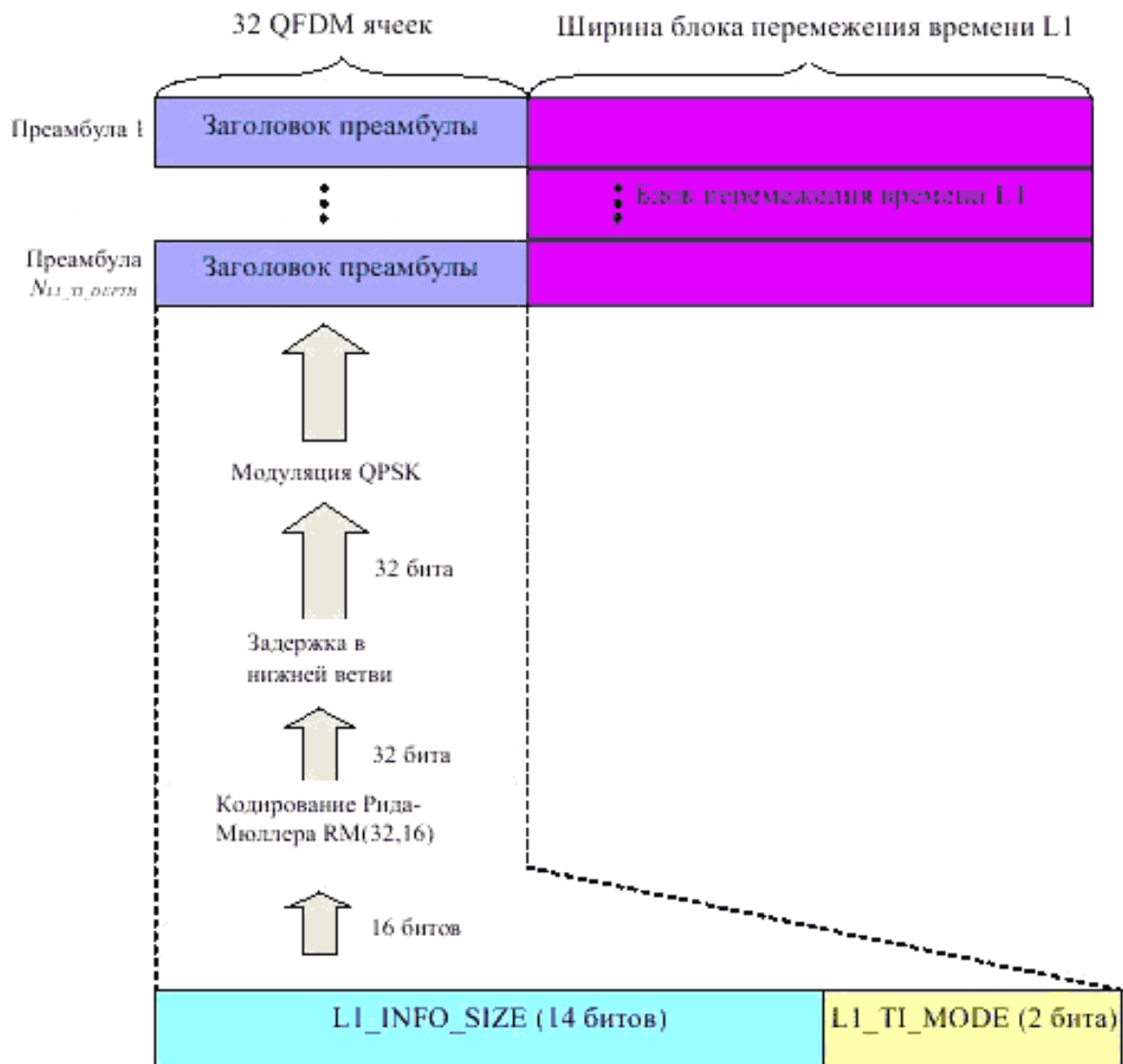
Р и с у н о к 23 – Формирование заголовка преамбулы и полей сигнализации
