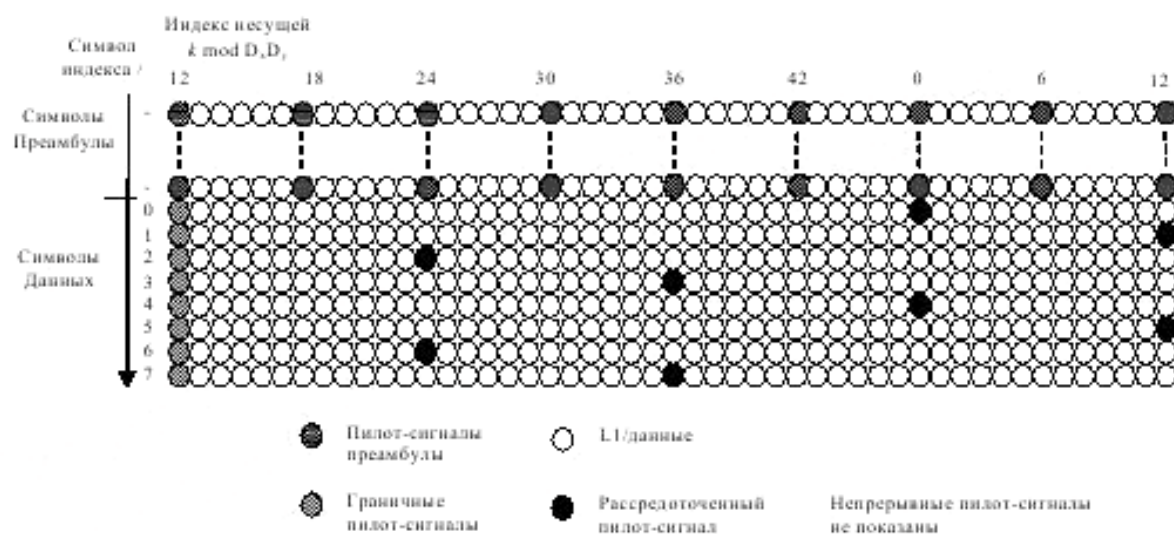
Р и с у н о к Е.2 – Рассредоточенный пилот-сигнал для GI 1/64 с низкочастотной границей k \bmod D_x D_y = 12
