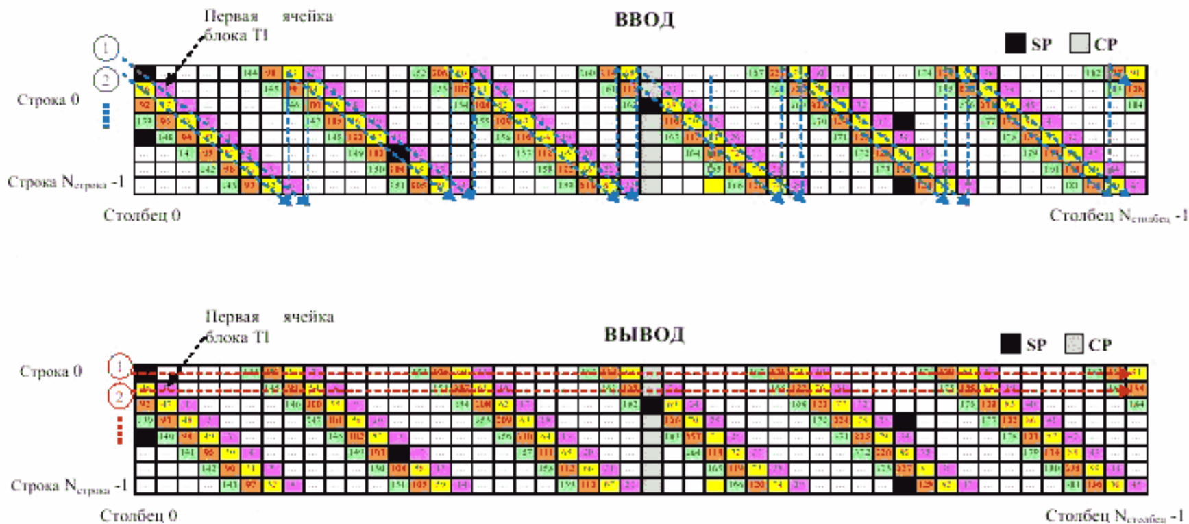
Р и с у н о к 39 – Схема записи и считывания ячеек в переключателе времени ( D_s=12 , GI=1/64 , N_s=8 , N_c=48 , DSLICE\_WIDTH=4 )
