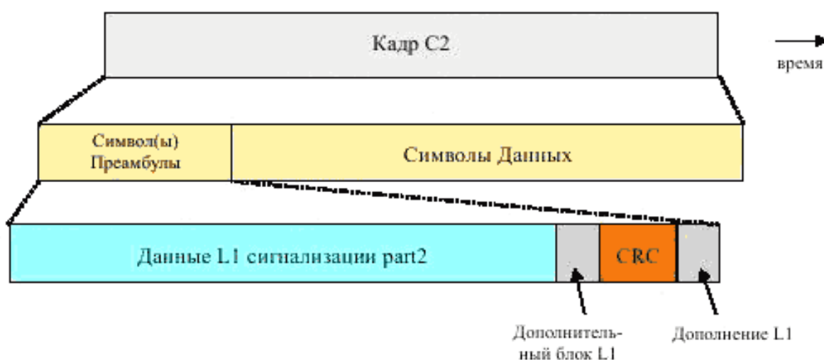
Р и с у н о к 22 – Структура данных сигнализации L1-part2
