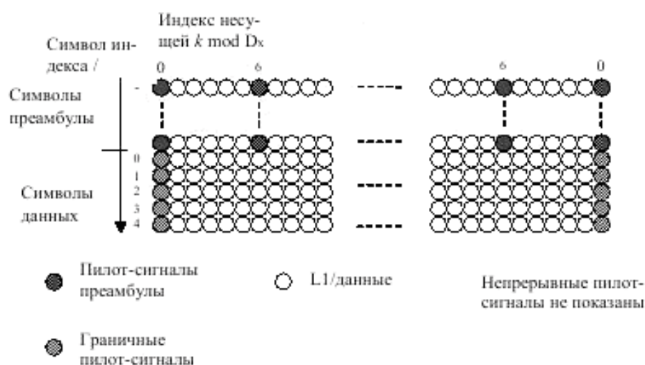
Р и с у н о к 41 – Расположение граничных пилот-сигналов в спектре OFDM сигнала
