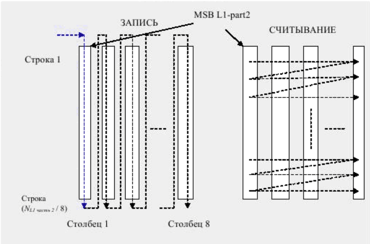
Р и с у н о к 30 – Схема перемежителя битов данных L1-part2 (16QAM)
