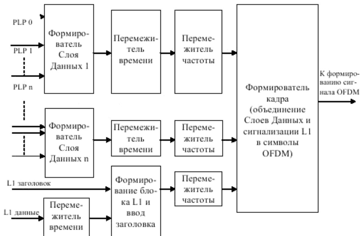
Р и с у н о к 4 – Блок-схема подсистемы формирования Слоя данных и ядра
