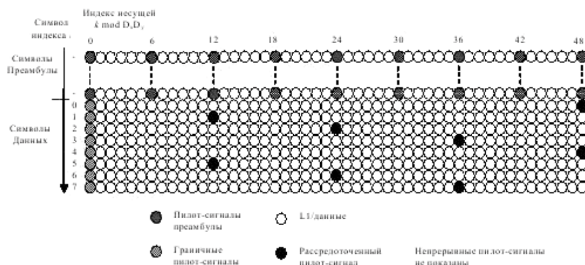
Рисунок Е.1 – Рассредоточенный пилот-сигнал для G_I 1/64 с низкочастотной границей k \bmod D_x D_y = 0
