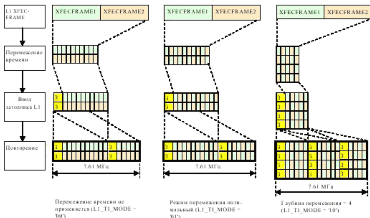
Р и с у н о к 31 – Перемежение времени данных сигнализации L1-part2
