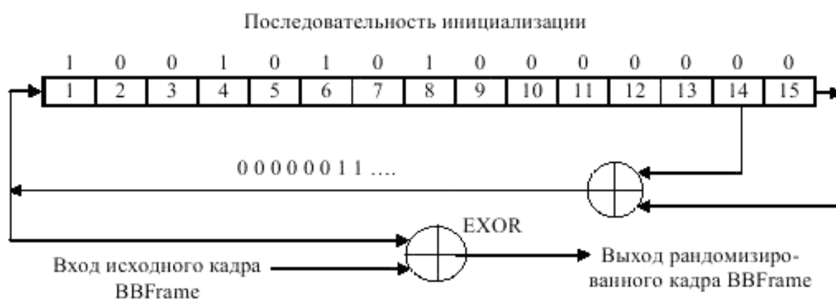
Р и с у н о к 13 – Структурная схема возможной реализации кодера псевдослучайной последовательности
