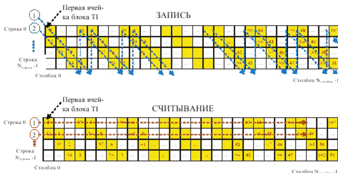
Р и с у н о к 32 – Перемежение времени данных сигнализации L1 (NMOD TOTAL=208, NLI TI DEPTH=4)
