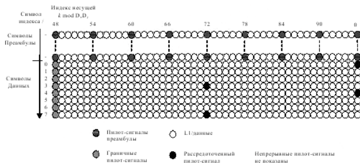
Р и с у н о к Е.7 – Рассредоточенный пилот-сигнал для GI 1/128 с низкочастотной границей k \bmod D_x D_y = 48
