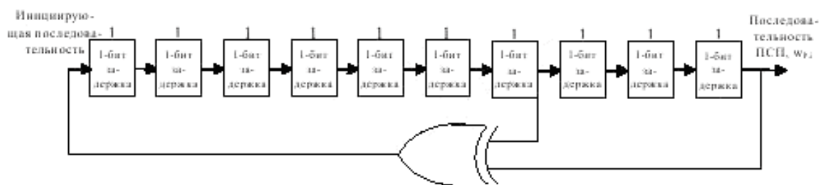
Р и с у н о к 35 – Схема генератора ПСП для модуляции пилот-сигналов
