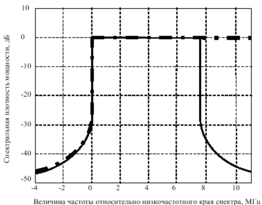
Р и с у н о к 43 – Расчетные спектры сигнала DVB-C2 для относительного интервала защиты 1/128 и с разными полосами пропускания (8 МГц и 445 МГц (только низкочастотный край спектра))
