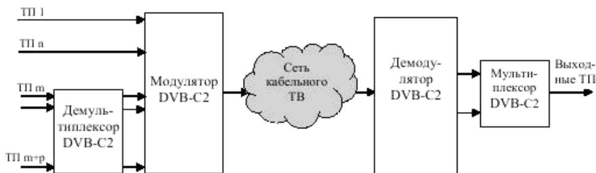
Р и с у н о к Б.1 – Расширение функциональных возможностей системы DVB-C2 при использовании демультимплексирования и мультимплексирования
