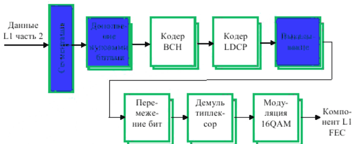
Р и с у н о к 25 – Структурная схема процессов кодирования и модуляции данных сигнализации L1-part2
