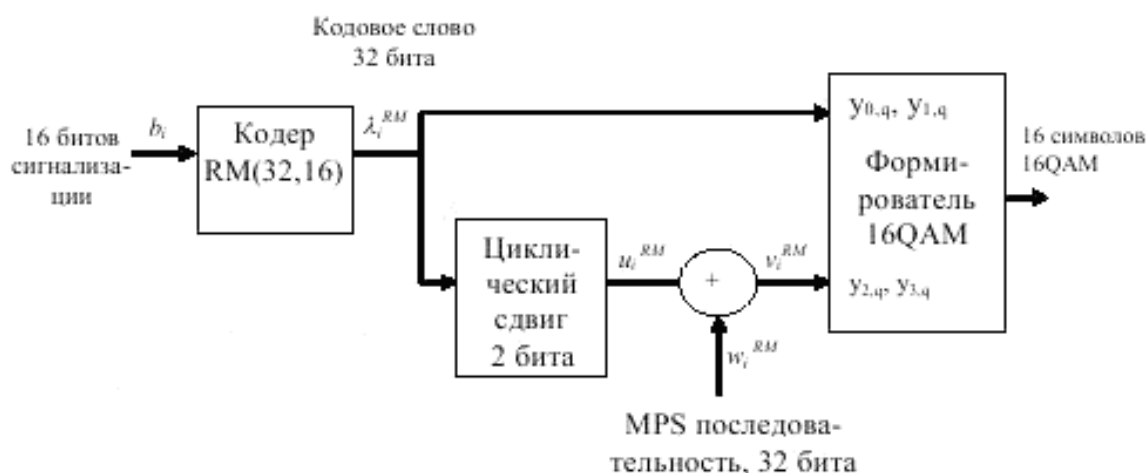
Р и с у н о к 21 – Заголовок FECFrame высокой производительности
