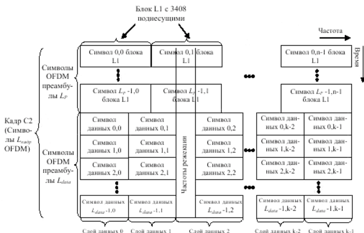
Р и с у н о к 33 – Структура кадра C2
