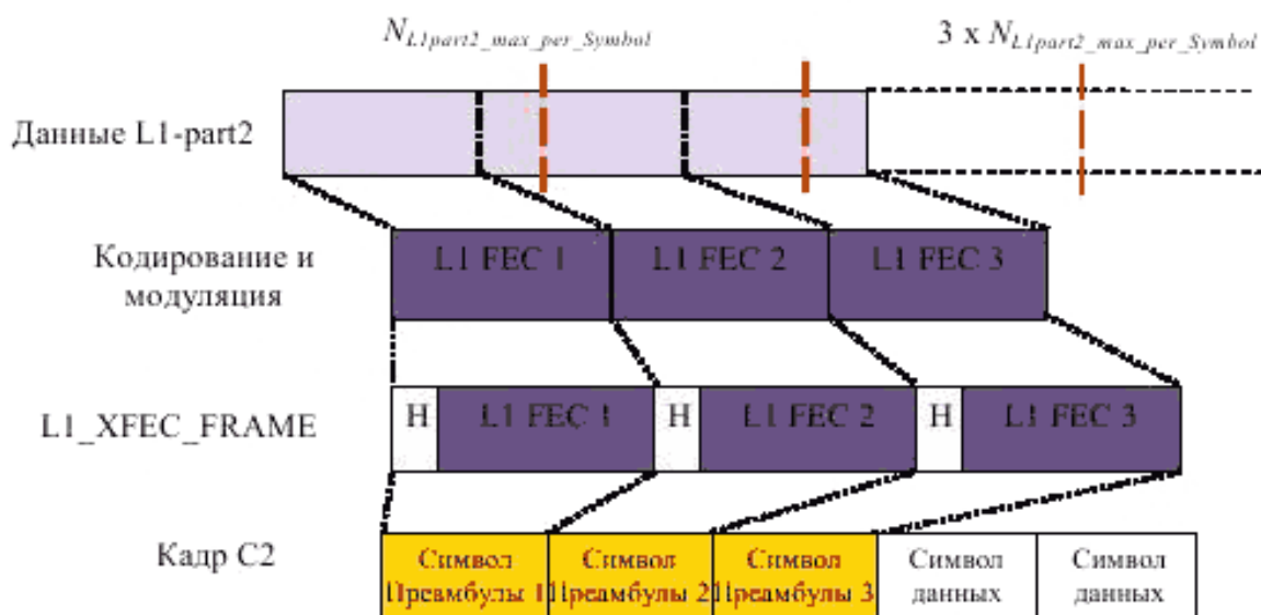
Рисунок 27 – Длина кодированных данных
