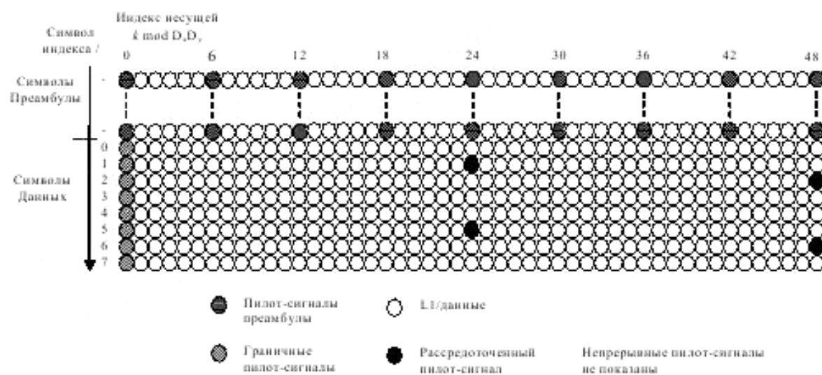
Р и с у н о к Е.5 – Распределенный пилот-сигнал для GI 1/128 с низкочастотной границей k \bmod D_x D_y = 0
