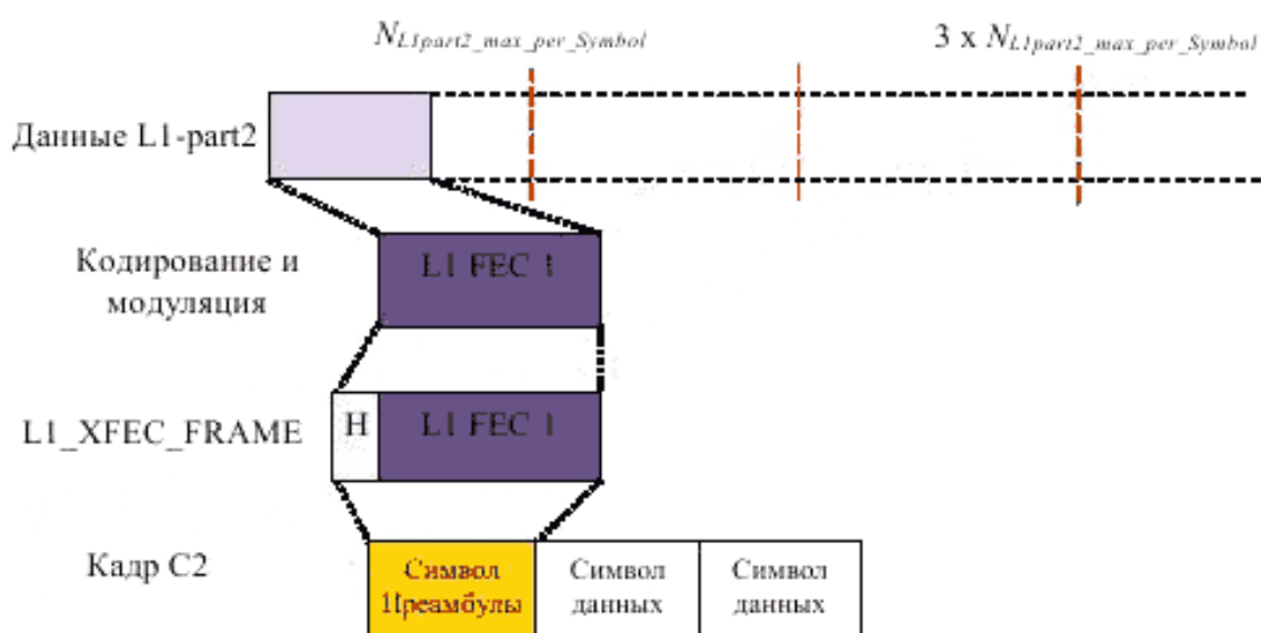
Рисунок 26 – Кодированные данные L1-part2
