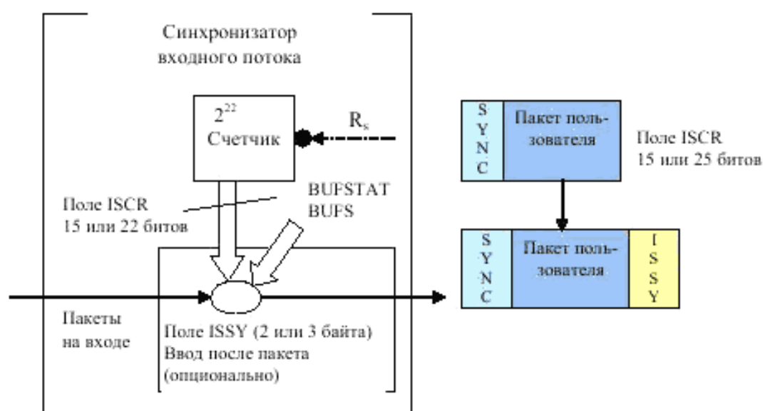
Р и с у н о к А.1 – Блок-схема синхронизатора входного потока
