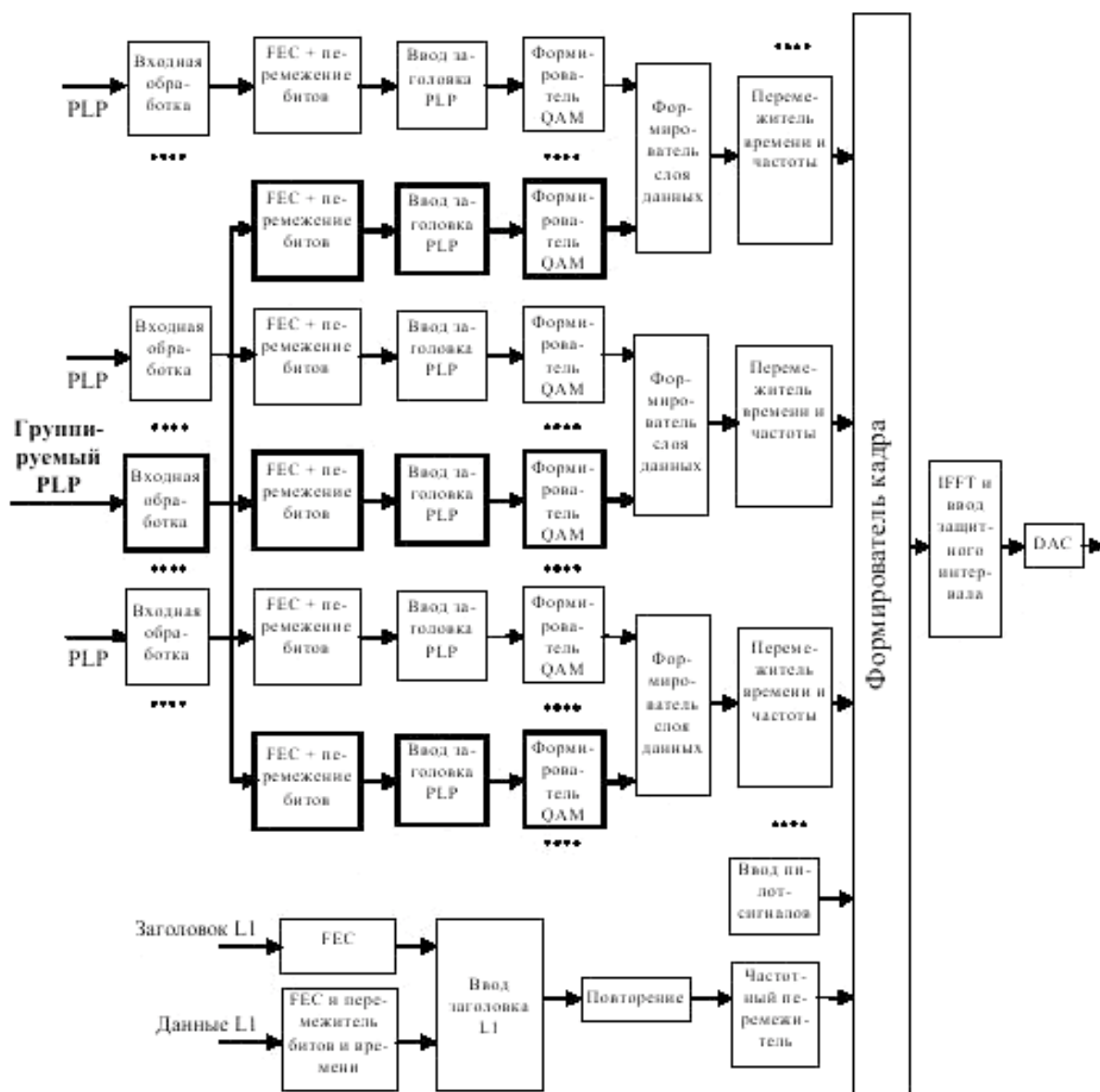
Р и с у н о к Г.1 – Блок-схема режима группирования PLP
