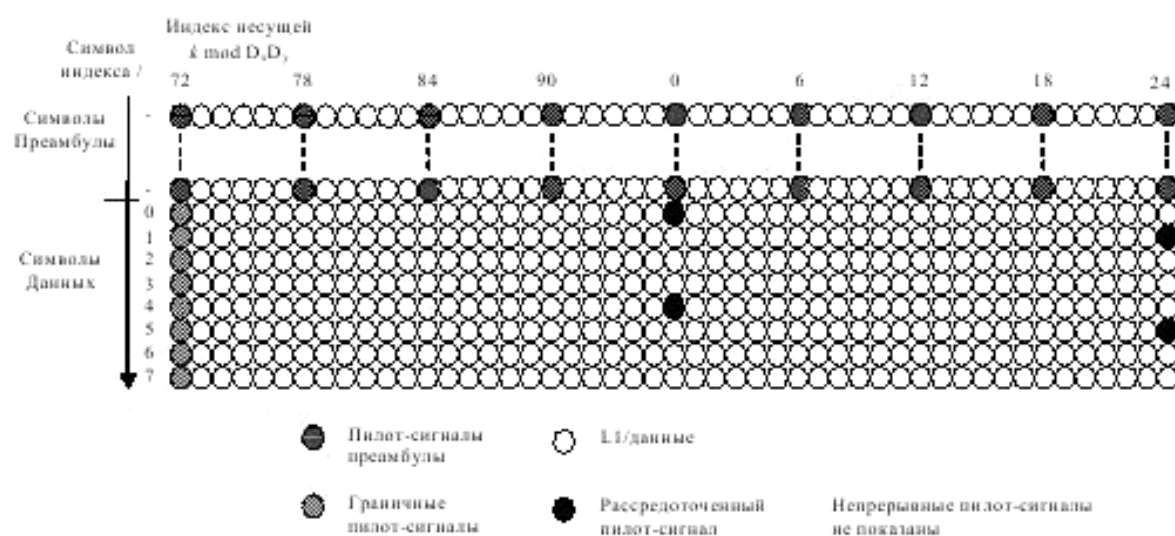
Р и с у н о к Е.8 – Рассредоточенный пилот-сигнал для GI 1/128 с низкочастотной границей k \bmod D_x D_y = 72
