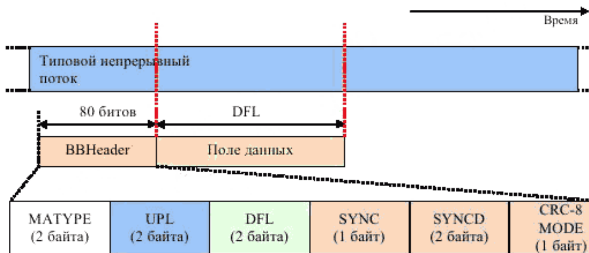
Р и с у н о к 11– Форматы потока GSE и GCS на выходе адаптера режима NM
