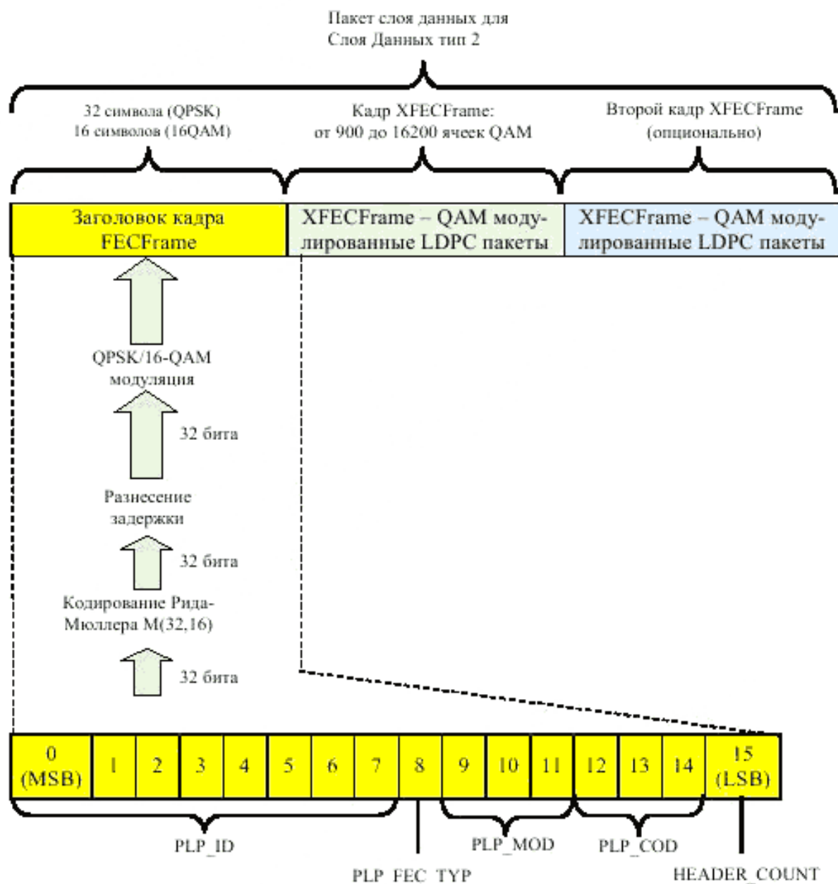
Р и с у н о к 19 – Пакет Слая Данных Тип 2, состоящий из заголовка FECFrame и следующих за ним пакетов XFECFrame
