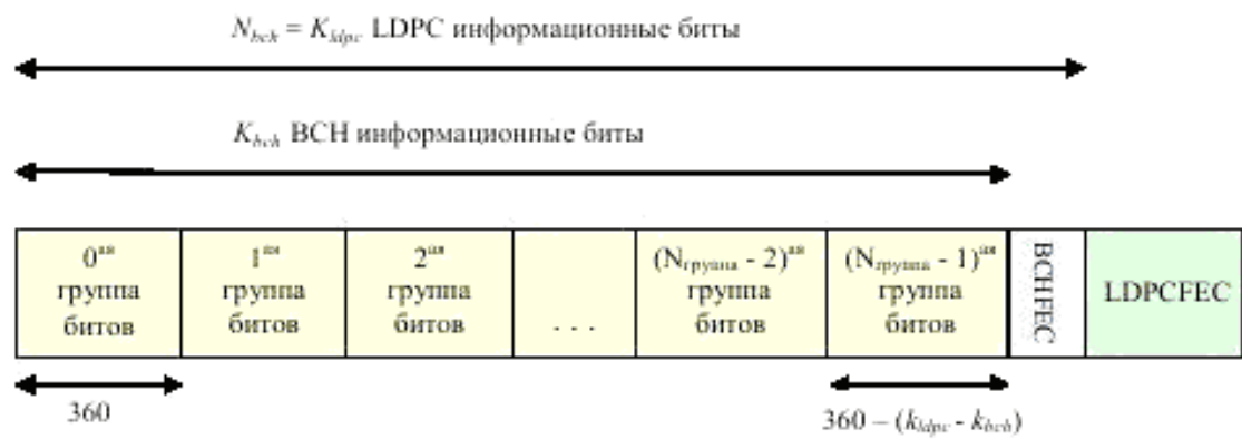
Р и с у н о к 29 – Формат данных сигнализации L1-part2 после кодирования LDPC
