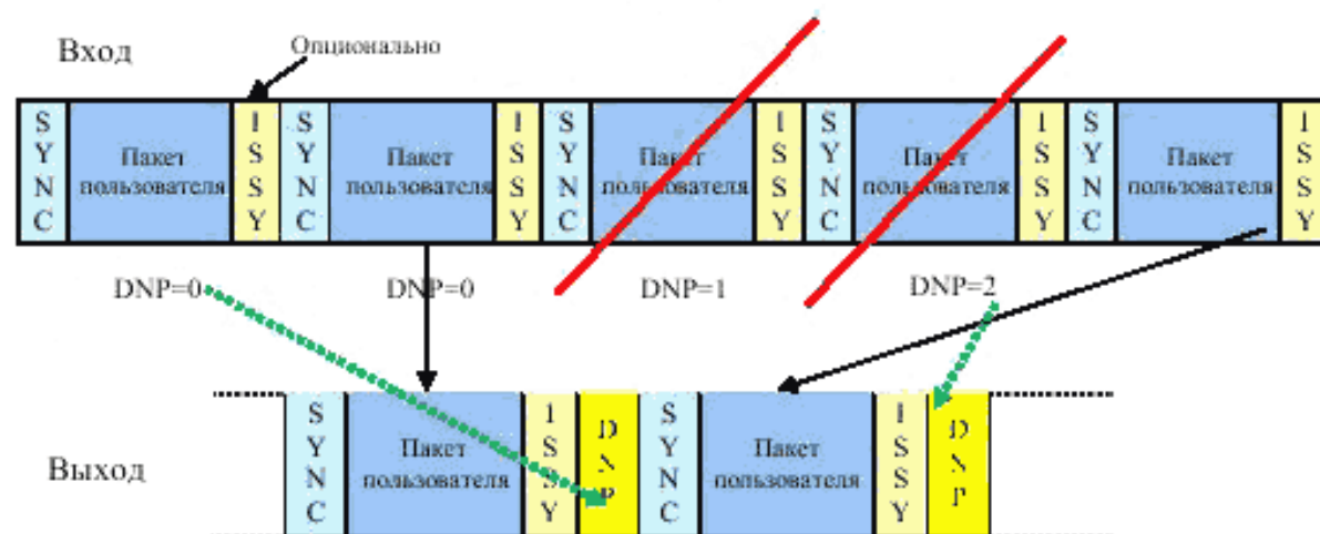
Р и с у н о к 6 – Схема удаления нулевых пакетов
