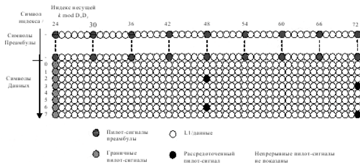
Р и с у н о к Е.6 – Рассредоточенный пилот-сигнал для GI 1/128 с низкочастотной границей k \bmod D_x D_y = 24
