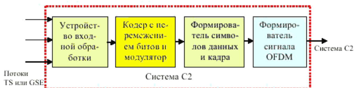
Р и с у н о к 1 – Обобщенная модель формирования Системы C2
