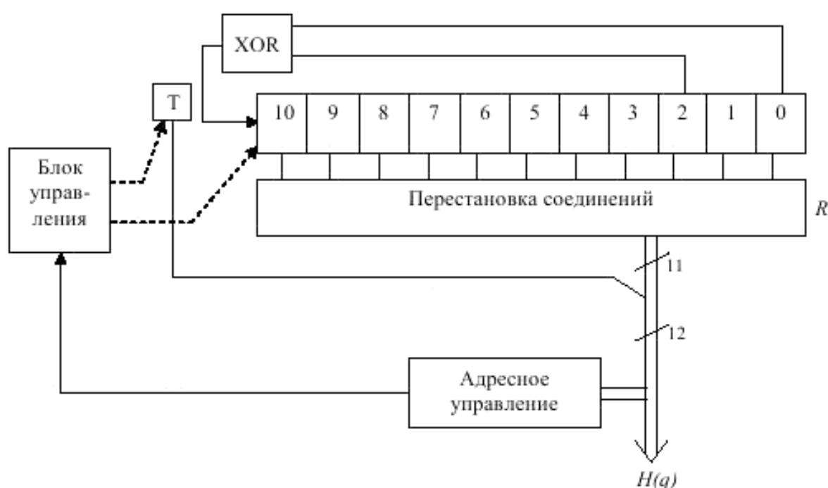
Р и с у н о к 40 – Блок-схема алгоритма формирования функции перестановки перемешителя частоты режима 4К
