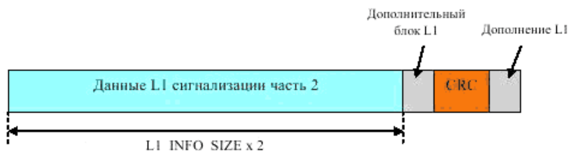
Р и с у н о к 24 – Размер поля L1_INFO_SIZE
