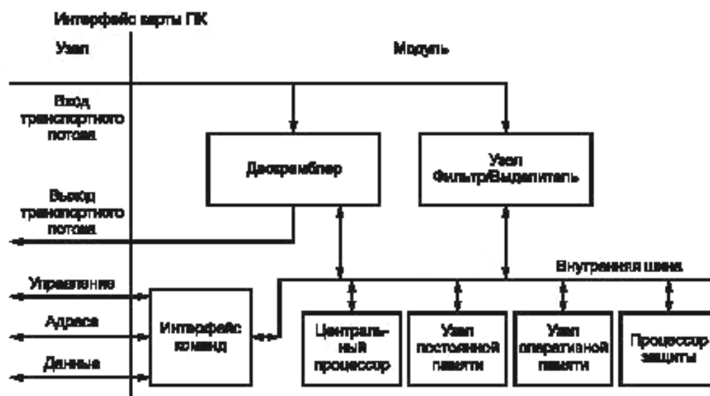
Рисунок А.1 — Типичная архитектура модуля
