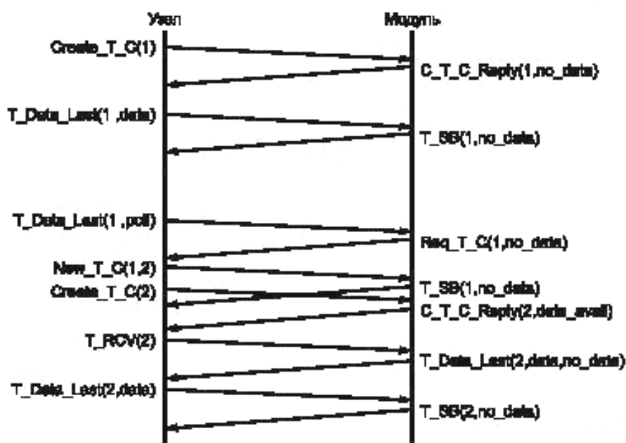
Рисунок 7 — Пример передачи объектов транспортного протокола
