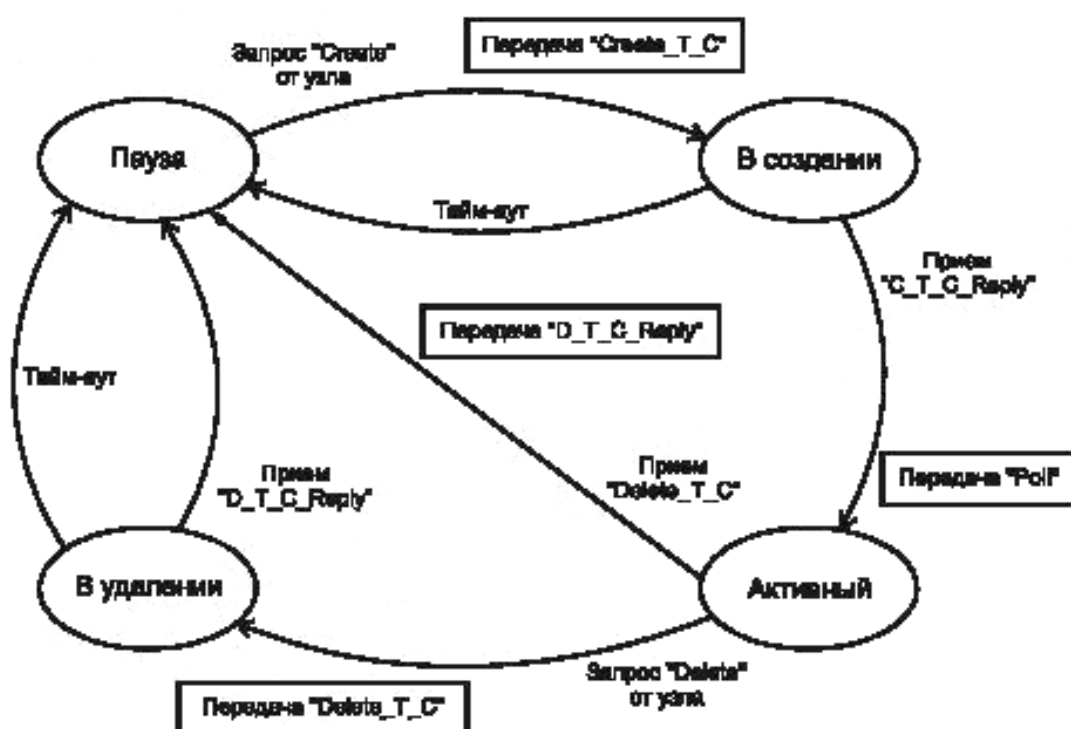
Рисунок 5 — Диаграмма состояний транспортного протокола на узле
