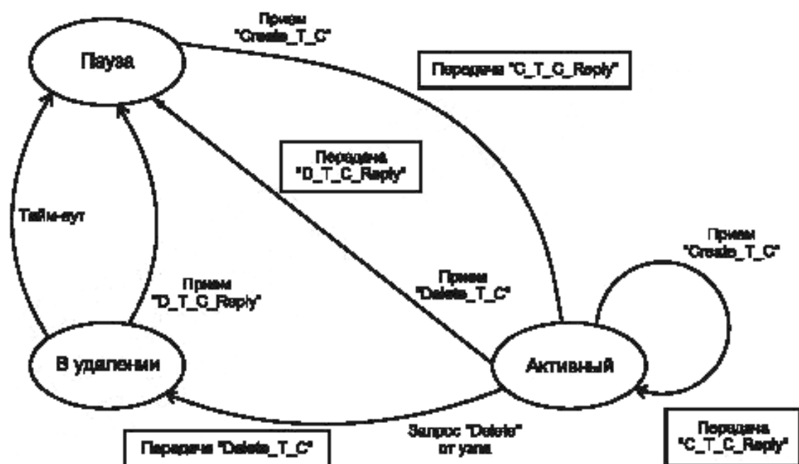
Рисунок 6 — Диаграмма состояний транспортного протокола на модуле
