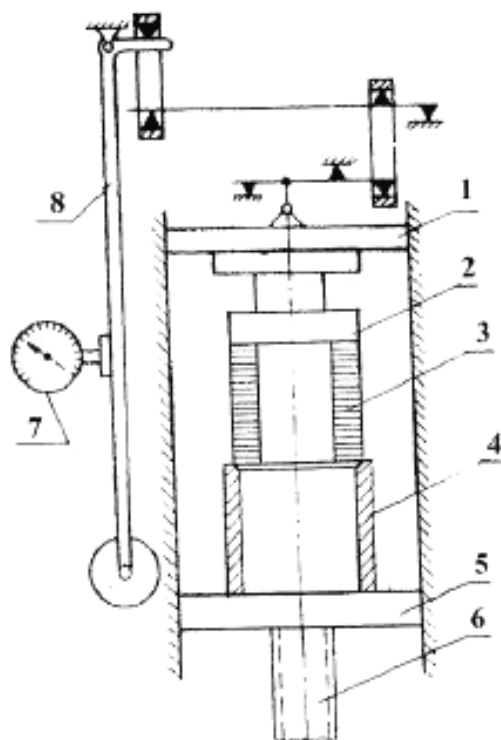
1 — верхняя плита; 2 — плунсон; 3 — втулка из МД; 4 — металлическая обойма; 5 — нижняя плита; 6 — винт; 7 — измеритель усилия; 8 — маятник
