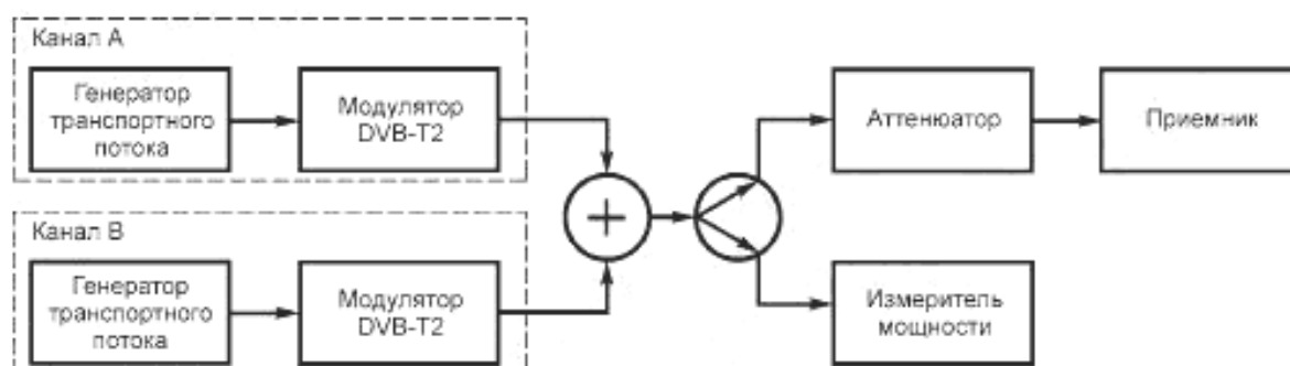
Рисунок 3 — Схема проверки 3
