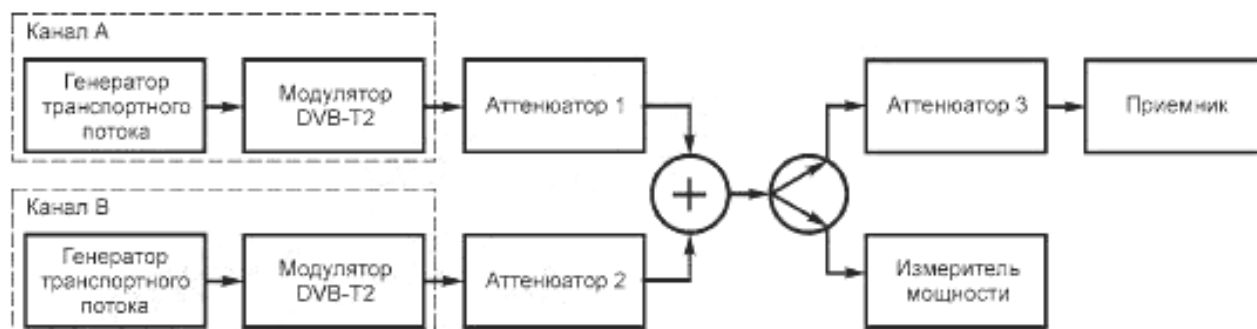
Рисунок 4 — Схема проверки 4
