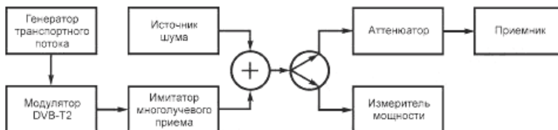
Рисунок 2 — Схема проверки 2
