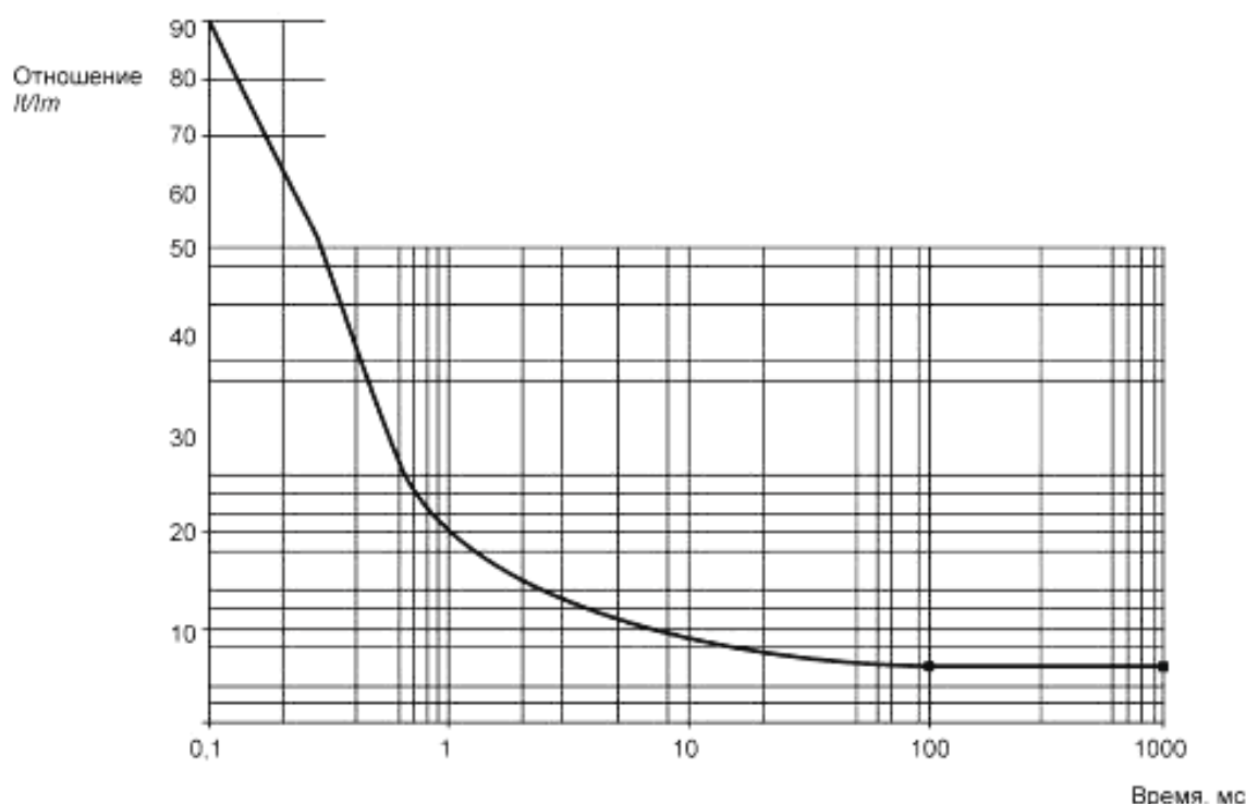
Рисунок 2 — Максимальный пусковой ток для телекоммуникационного оборудования
