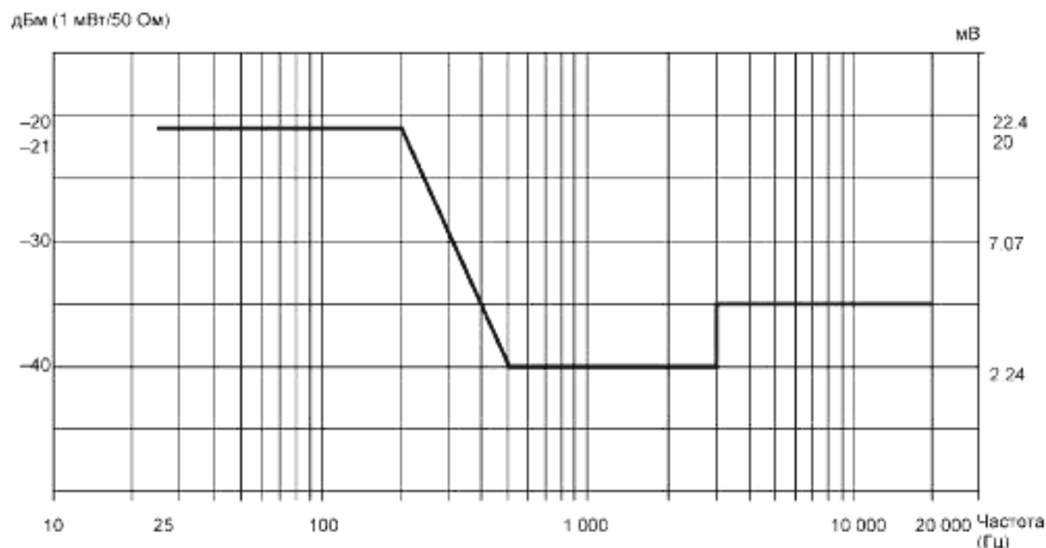
Рисунок 6 — Максимальные уровни узкополосного шума
