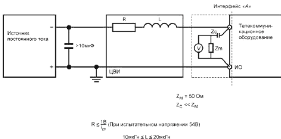
Рисунок 7 — Схема измерения для внесенного узкополосного и широкополосного шума
