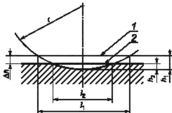
1, 2 — поверхность трения до и после изнашивания соответственно; l_1 , l_2 — длина лунки до и после изнашивания соответственно; h_1 , h_2 — глубина лунки до и после изнашивания соответственно; \Delta h — линейный износ, r — радиус вращения вершины резца
