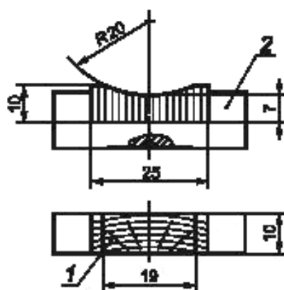
1 — образец из МД; 2 — оправка
