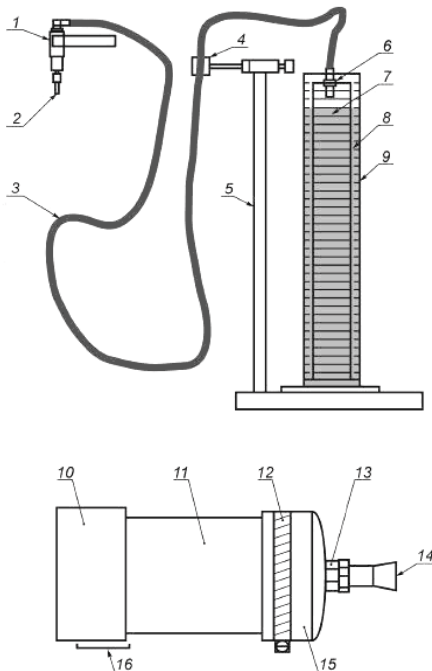
1 — клапан отключения; 2 — разъем быстрого соединения («папа»); 3 — гибкий шланг; 4 — зажим шланга; 5 — станка для бюретки; 6 — штуцер перегородки; 7 — заполняющая жидкость; 8 — внутренний градуированный цилиндр; 9 — большой внешний градуированный цилиндр; 10 — крышка из ПВХ трубки толщиной стенки 40 мм; 11 — ПВХ трубка толщиной стенки 40 мм, диаметр и высота которой определяется размером хвоста; 12 — зажимное устройство; 13 — штуцер перегородки; 14 — разъем быстрого соединения («мама»); 15 — крышка из резины или ПВХ; 16 — клеевое соединение
