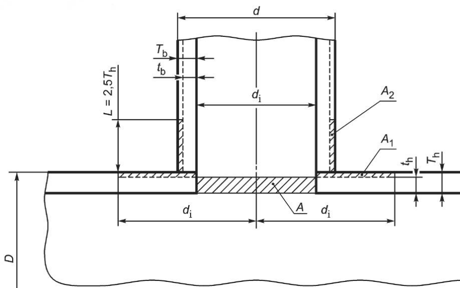
Рисунок Б.1 — Схема для расчета TC (сечение продольной плоскостью симметрии — фрагмент)
