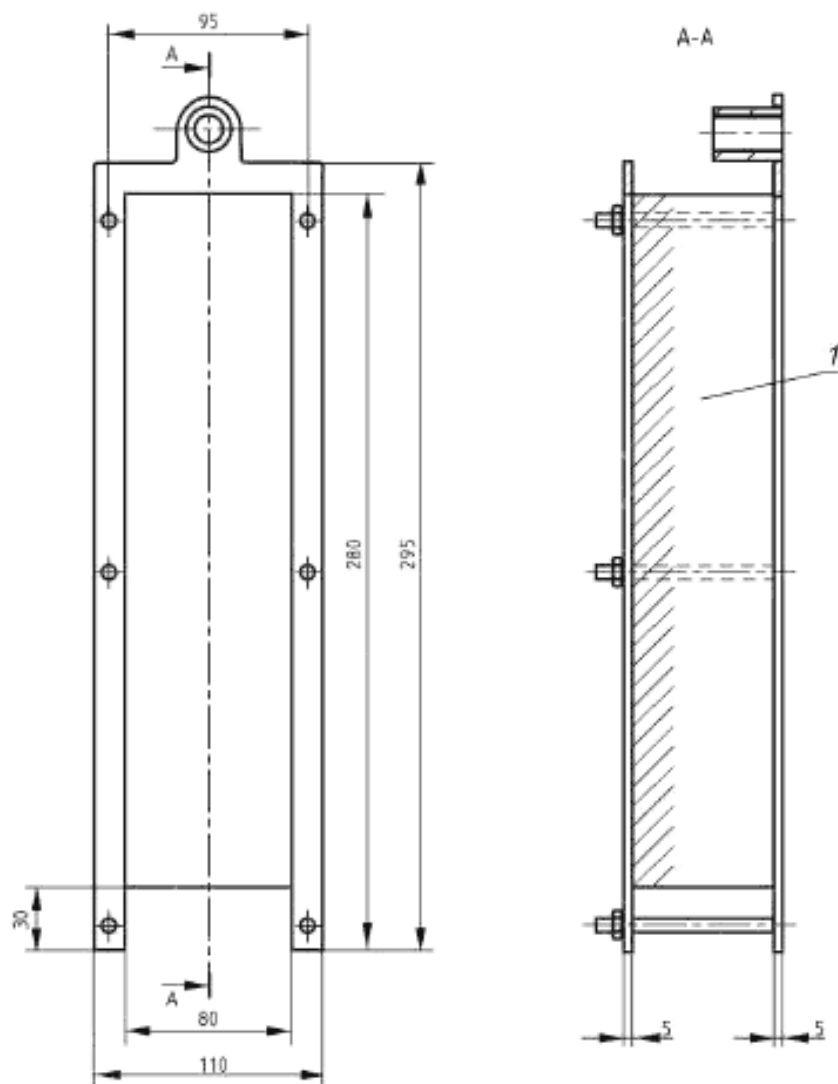
Рисунок Б.1 – Держатель образца
